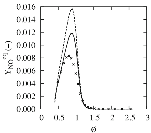
(d) NO mass fraction
