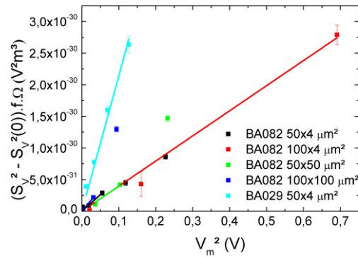
Figure IV-6 Densité spectrale de bruit en tension multiplié par la fréquence et le volume en fonction de V_m^2 .
