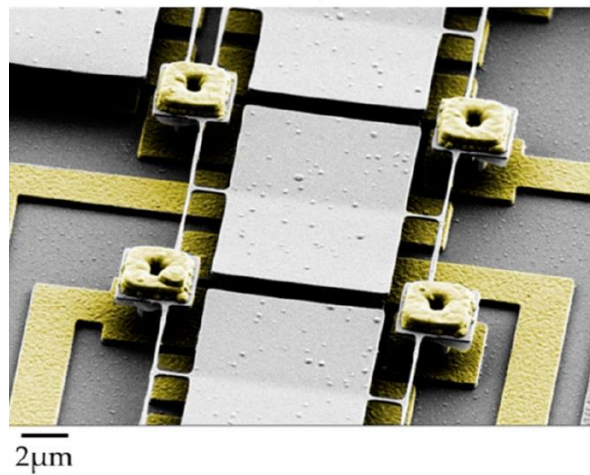
Figure I-5 Exemple de nano résonateur [Duraffourg 2018].
