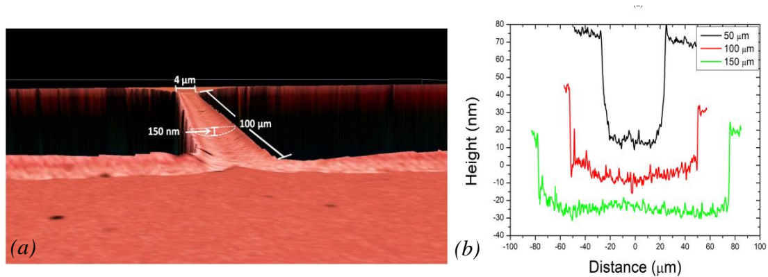
Figure II-18 Image au microscope confocal 3D d'un pont suspendu de 4\ \mu\text{m} de large, 100\ \mu\text{m} de longueur, structuré dans un film LSMO de 75\ \text{nm} d'épaisseur déposé sur \text{STO}/\text{Si} ; (b) les lignes de profil en coupe le long de la longueur (mesurée au centre de la largeur du pont) des ponts LSMO de 50 , 100 et 150\ \mu\text{m} de longueur ( CA508-17A) [S. Liu 2019].
