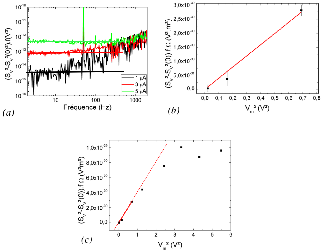
Figure IV-5 Exemple de la méthode d'extraction du paramètre normalise de Hooge à partir des mesures de densités spectrales de bruit en tension pour le pont 100 \times 4 \mu\text{m}^2 (BA082). (a) Soustraction de la densité spectrale de bruit en tension à courant nul pour chaque densité spectrale de bruit en tension mesurée à un courant donné (Figure IV-7) puis multiplication par la fréquence, pour estimer le bruit en 1/f à 1 Hz (b) Densités spectrales de bruit en tension de l'échantillon à 1 Hz en fonction de V_m^2 pour des courants entre 1 et 5 \mu\text{A} . (c) Densités spectrales de bruit en tension de l'échantillon à 1 Hz en fonction de V_m^2 pour courants entre 1 et 15 \mu\text{A} .
