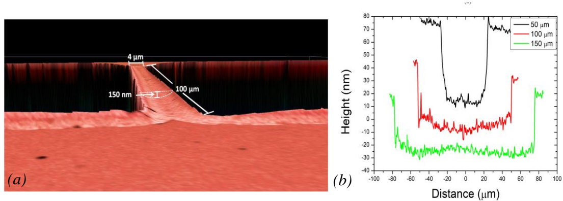
Figure II-18 Image au microscope confocal 3D d'un pont suspendu de 4\ \mu\text{m} de large, 100\ \mu\text{m} de longueur, structuré dans un film LSMO de 75\ \text{nm} d'épaisseur déposé sur \text{STO}/\text{Si} ; (b) les lignes de profil en coupe le long de la longueur (mesurée au centre de la largeur du pont) des ponts LSMO de 50 , 100 et 150\ \mu\text{m} de longueur ( CA508-17A) [S. Liu 2019].
