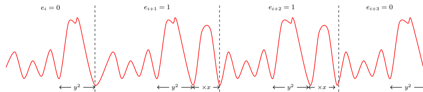
FIGURE 4.1 – Illustration d'une SPA contre l'exponentiation rapide
