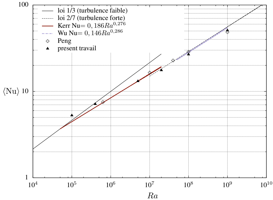
Figure 4.12 : Evolution du nombre de Nusselt \langle \text{Nu} \rangle à la paroi avec les deux lois de turbulence.
