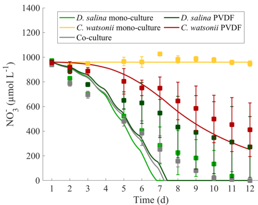
Figure 76 : Expérience 1 de calibration : concentration en nitrates au cours du temps en mono-culture, co-culture et co-culture PVDF
