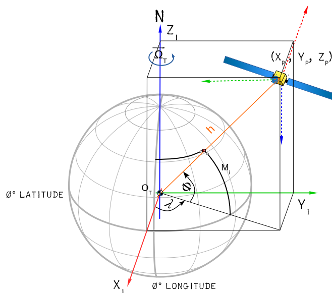
FIGURE 1.5 – Coordonnées tangentielles
