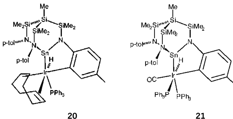
Figura 3.53 Complejos heterobimetálicos \text{Ir}^{\text{III}}\text{-Sn}^{\text{IV}} reportados por el grupo de investigación de Lutz H. Gade. 59,60
