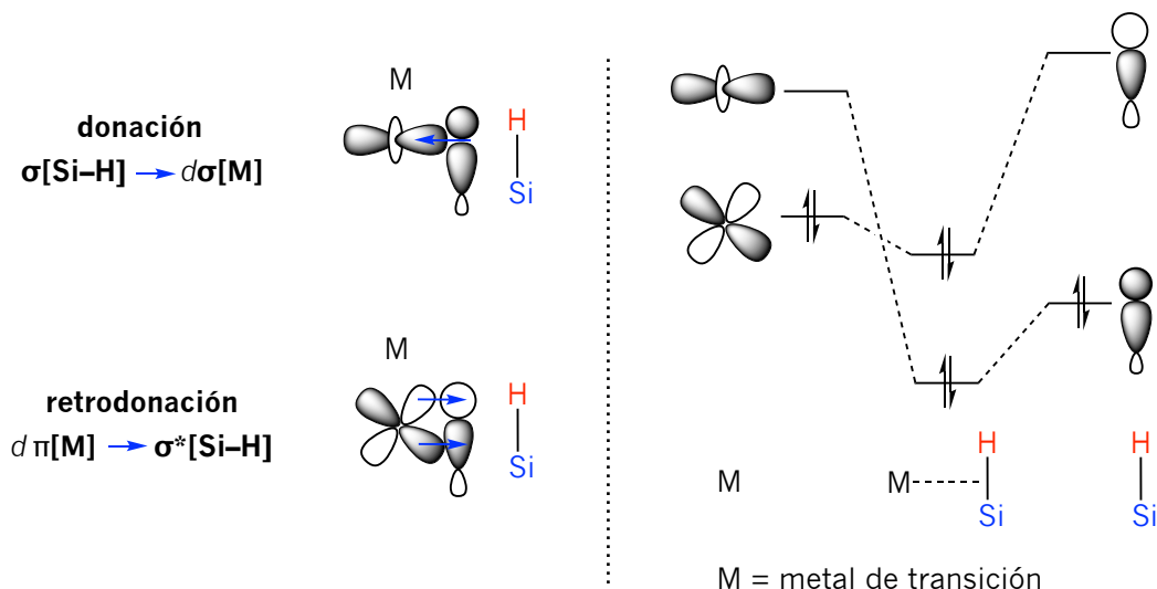
Figura 1.4 Representación esquemática del enlace sinérgico donación/retrodonación [\text{Si-H}] \rightarrow \text{M} / \text{M} \rightarrow [\text{Si-H}] .
