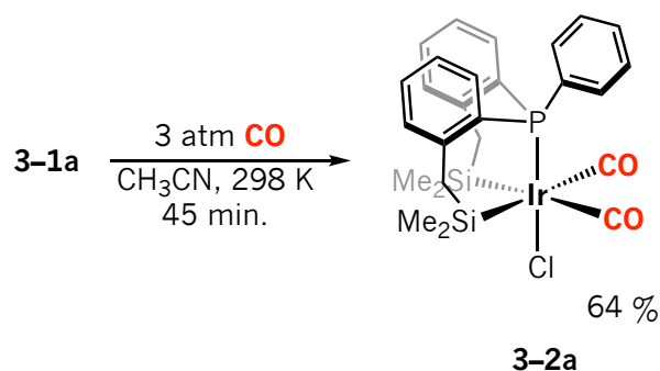
Esquema 3.6 Síntesis del complejo dicarbonilo [(\text{SiPSi})\text{IrCl}(\text{CO})_2] 3-2a .
