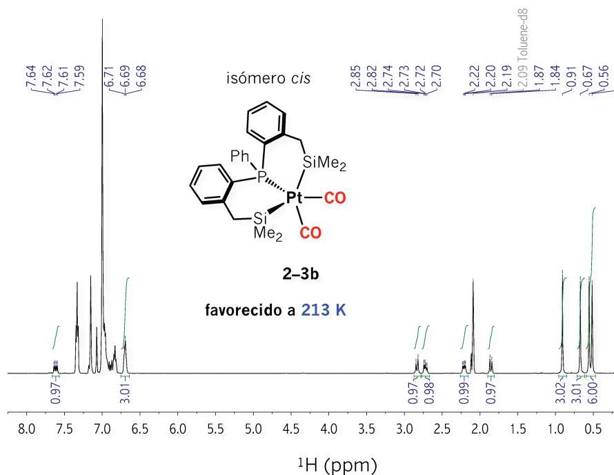
Figura 2A.8. Espectro de RMN de ^1\text{H} (500 MHz, 213 K, \text{tol}-d_8 ) correspondiente a la reacción del complejo 2-1 frente a 3 atm de CO en \text{tol}-d_8 llevada a cabo en un tubo de RMN de presión. Detección espectroscópica de la isomerización cis/trans 2-3b/2-3a .
