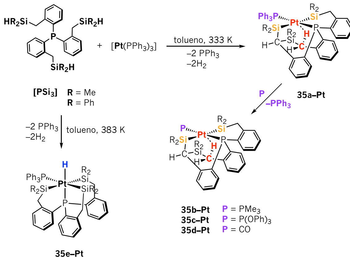
Esquema 1.43 Síntesis de complejos de Pt^{II} , d^8 cuadrado planos 35a-Pt , 35b-Pt , 35c-Pt y 35d-Pt ; e hidruro de Pt^{IV} 35e-Pt a partir del ligando [PSi_3] frente al precursor de platino [Pt(PPh_3)_3] . 97,25
