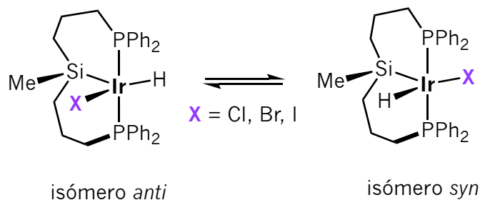
Esquema 3.21 Isomerización de complejos de \text{Ir}^{\text{III}} d^6 pentacoordinados [\text{IrX}(\text{biPSi})] propuestos por el grupo de investigación de Sola. 9t
