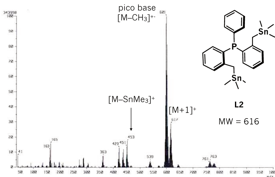
Figura 3.50 Espectro de masas (ionización química) correspondiente al ligando L2 .
