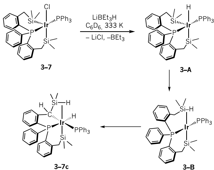
Esquema 3.24 Mecanismo propuesto para la formación del complejo 3-7c .
