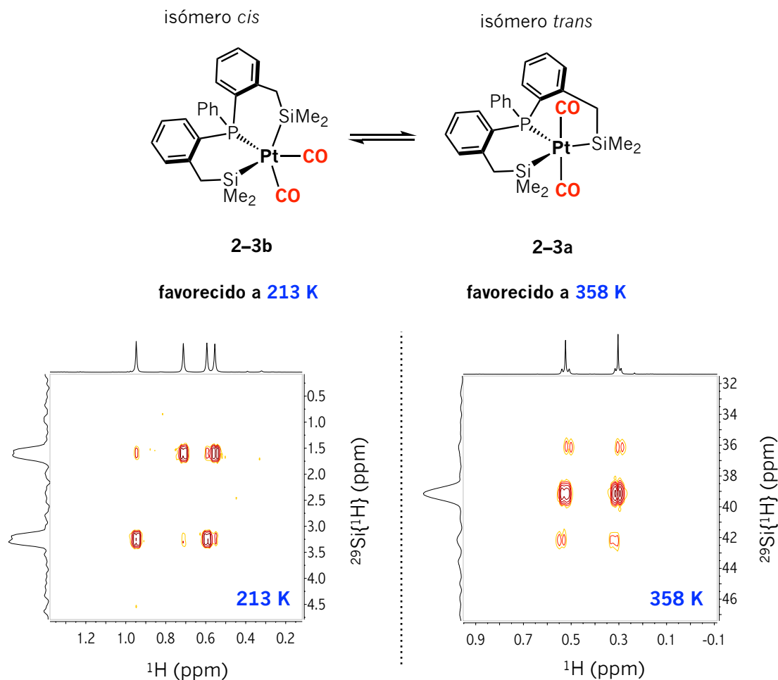
Figura 2.11 Espectros de RMN de 2D ^1H - ^{29}Si HMQC adquiridos a 213 y 358 K correspondientes a la reacción del complejo 2-1 frente a 3 atm de CO en tol-d_8 llevada a cabo en un tubo de RMN de presión. Detección espectroscópica de la isomerización cis / trans 2-3b / 2-3a .
