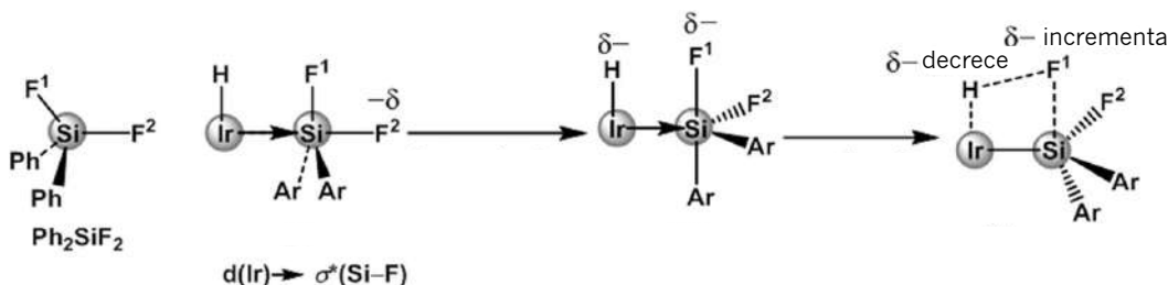
Esquema 1.17 Secuencia de reacción de la activación del enlace Si-F de 12 por el precursor metálico [Ir(H)(CO)(PPh_3)_3] . 65
