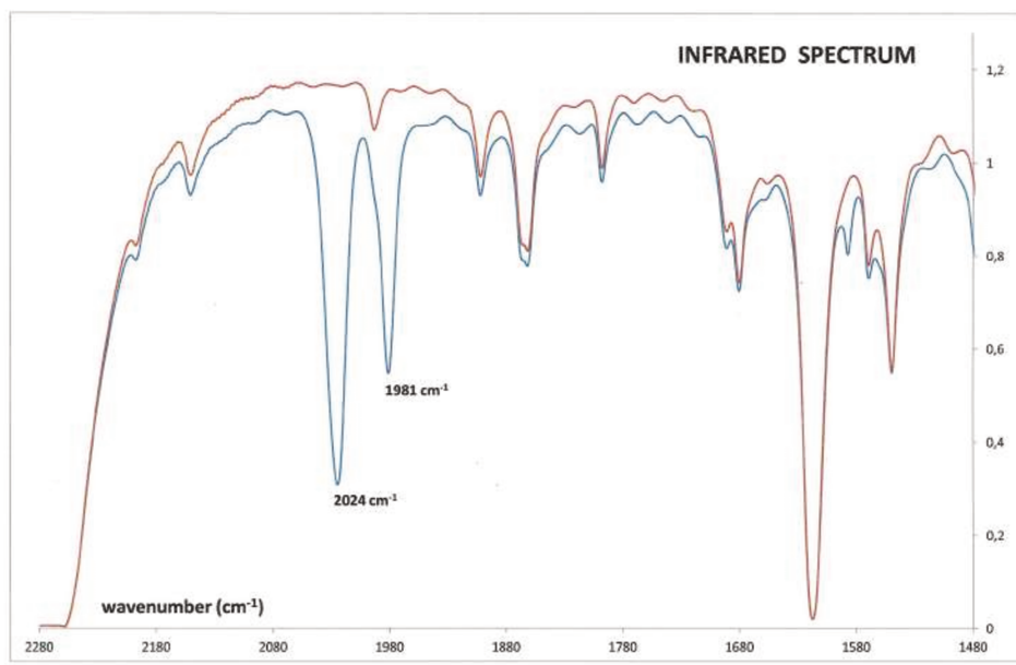
Figura 2A.7. Espectro IR-ATR medido a 298 K en disolución de \text{C}_6\text{D}_6 correspondiente a la reacción del complejo 2-1 frente a 1 atm de CO (espectro azul). El espectro rojo corresponde al del disolvente, \text{C}_6\text{D}_6 .
