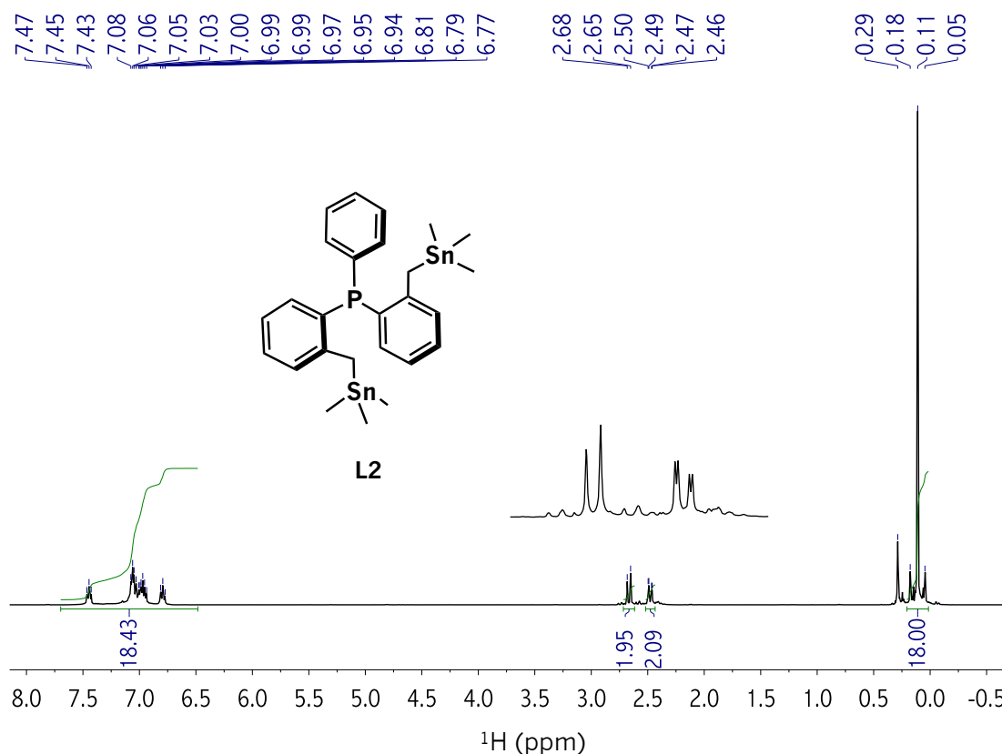
Figura 3.51 Espectro de RMN ^1\text{H} (400 MHz, 298 K, \text{C}_6\text{D}_6 ) correspondiente al ligando L2 .
