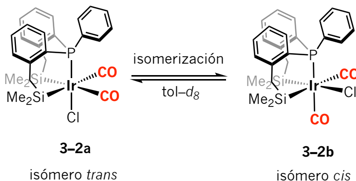
Esquema 3.7 Isomerización cis/trans del complejo 3-2a en solución de tol-d 8 .
