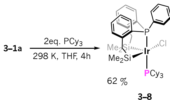
Esquema 3.25 Síntesis del complejo [(\text{SiPSi})\text{Ir}(\text{Cl})(\text{PCy}_3)] 3-8 .
