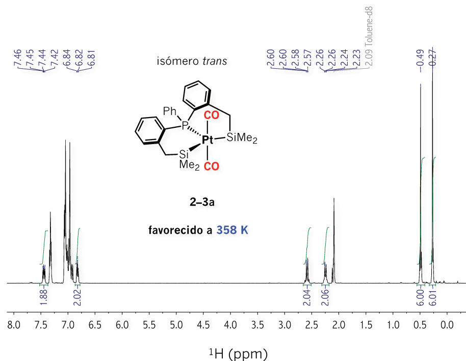
Figura 2A.9. Espectro de RMN de ^1\text{H} (500 MHz, 358 K , \text{tol-}d_8 ) correspondiente a la reacción del complejo 2-1 frente a 3 atm de CO en \text{tol-}d_8 llevada a cabo en un tubo de RMN de presión. Detección espectroscópica de la isomerización cis/trans 2-3b/2-3a .
