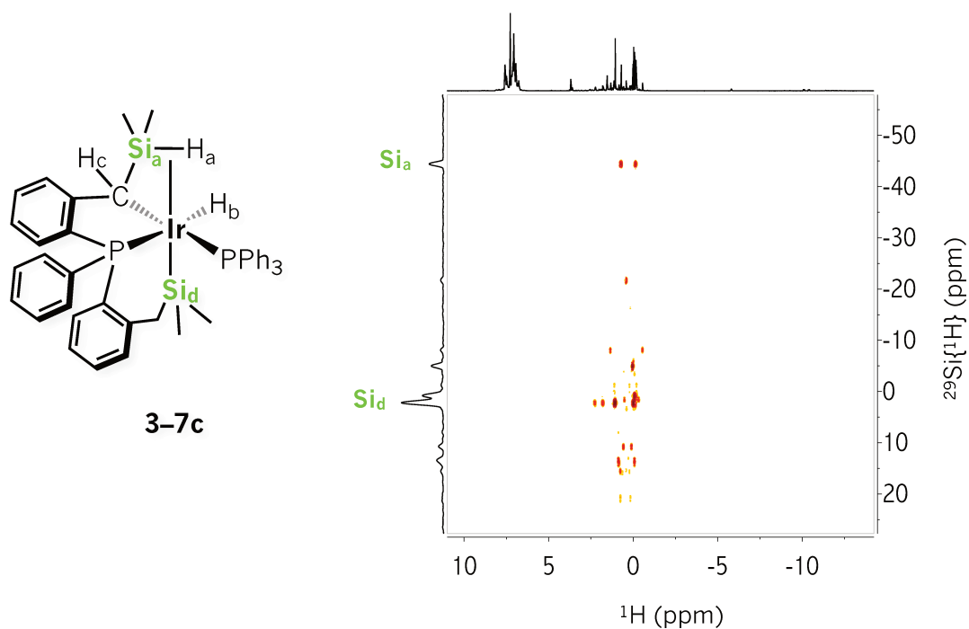
Figura 3A.26 RMN de 2D ^1\text{H} - ^{29}\text{Si} HMQC (298 K, \text{C}_6\text{D}_6 ) correspondiente a la reacción del complejo 3-7 frente a 1 eq. de \text{LiBET}_3\text{H} en disolución de \text{C}_6\text{D}_6 a 333 K. Detección espectroscópica del complejo 3-7c .
