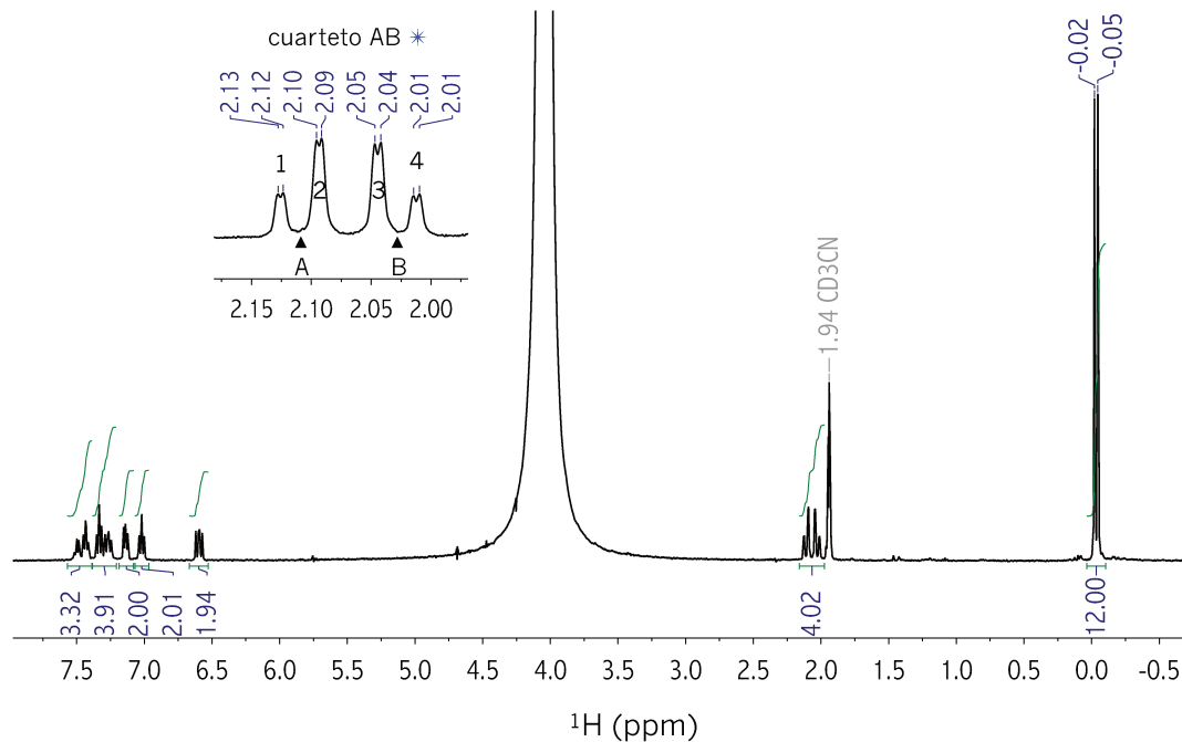
Figura 3.22 RMN de ^1\text{H} (400 MHz, 298 K, \text{CD}_3\text{CN} ) correspondiente a la reacción del complejo 3-1a en disolución de \text{CD}_3\text{CN} con un exceso de agua a 298 K. 36 Detección espectroscópica del aducto 3-4c . * |J_{AB}| = (\nu_1 - \nu_2) = (\nu_3 - \nu_4) = 12.0 \text{ Hz} , J = 4.0 \text{ Hz} , \Delta\nu_{AB} = \sqrt{(\nu_1 - \nu_4)(\nu_2 - \nu_3)} = 30.3 \text{ Hz} .
