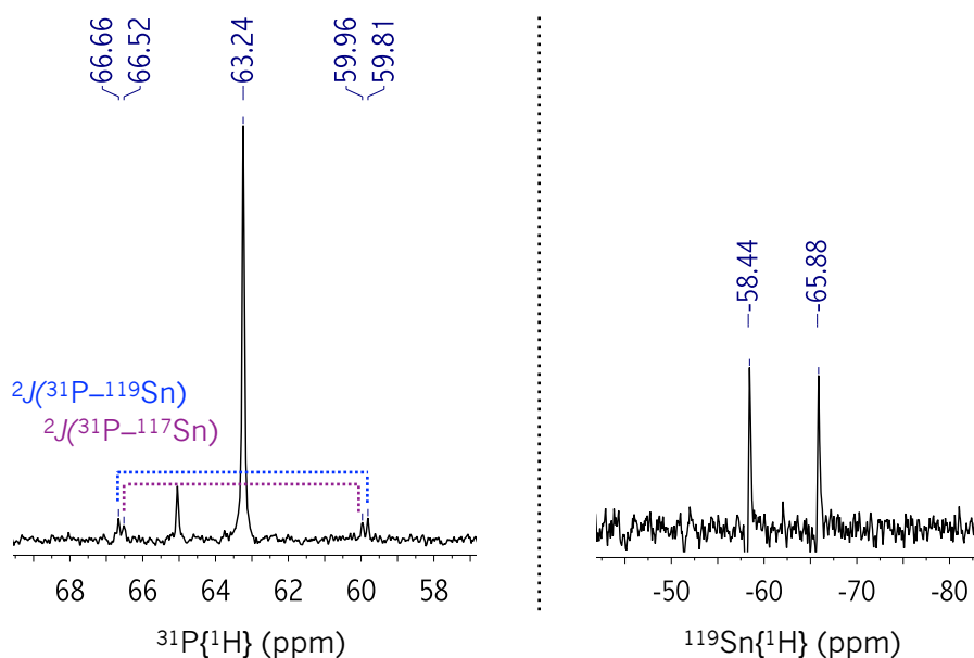
Figura 3.55 Espectros de RMN correspondientes al complejo 3-10 . Izquierda: {}^{31}\text{P}\{^1\text{H}\} (161.9 MHz, 298 K, \text{C}_6\text{D}_6 ). Derecha: {}^{119}\text{Sn}\{^1\text{H}\} (149 MHz, 298 K, \text{C}_6\text{D}_6 ).
