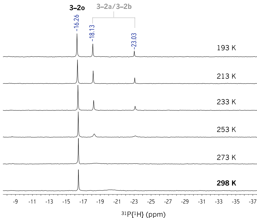
Figura 3.11 RMN de ^{31}\text{P}\{^1\text{H}\} (202.5 MHz, \text{tol-}d_8 ) a diferentes temperaturas correspondiente a la reacción “ in situ ” del complejo 3-1a frente a 1 atm de CO en disolución de \text{tol-}d_8 en un tubo de RMN de presión.
