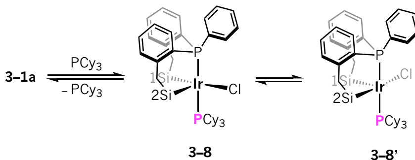
Esquema 3.27 Equilibrios propuestos para el complejo 3-8 y la disociación reversible de la fosfina \text{PCy}_3 que da lugar a 3-1a en disolución de \text{C}_6\text{D}_6 , \text{tol-}d_8 y \text{THF-}d_8 .
