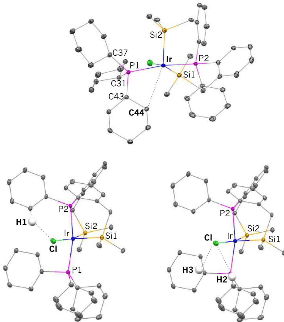
Figura 3.41 Diagramas ORTEP del complejo 3-8 · 2(CH 2 Cl 2 ) enfatizando la interacción agóstica \gamma\text{C-H}\cdots\text{Ir} (arriba) y las interacciones \text{Cl}\cdots\text{H1} , \text{Cl}\cdots\text{H2} y \text{Cl}\cdots\text{H3} (abajo). Elipsoides térmicos al 30 % de probabilidad. Los átomos de hidrógeno y los del disolvente han sido omitidos para mayor claridad excepto H1, H2 y H3.
