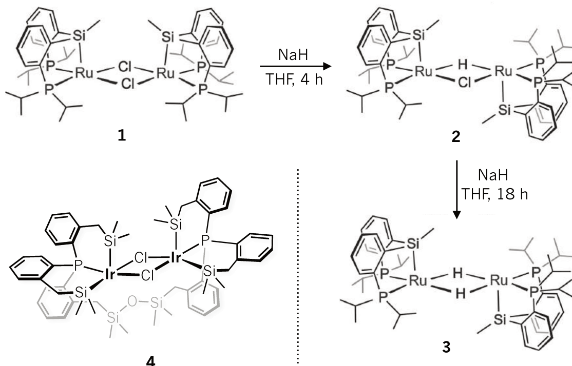
Esquema 3.3 Síntesis de estructuras dinucleares de Ru II enlazados al ligando [PSiP] con hidruros puente y estructura del complejo siloxano [Ir 2 (μ-Cl) 2 {P((o-C 6 H 4 )CH 2 SiMe 2 ) 3 ] 2 ] 2 O 4 con el ligando [PSi 3 ].
