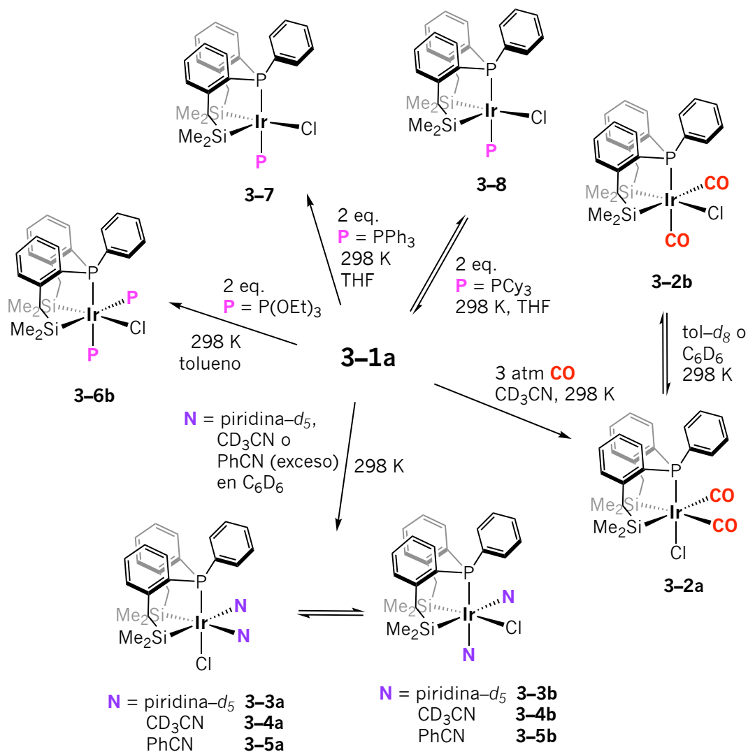
Esquema 3.5 Reactividad del complejo 3-1a frente a ligandos neutros donadores de 2 electrones.
