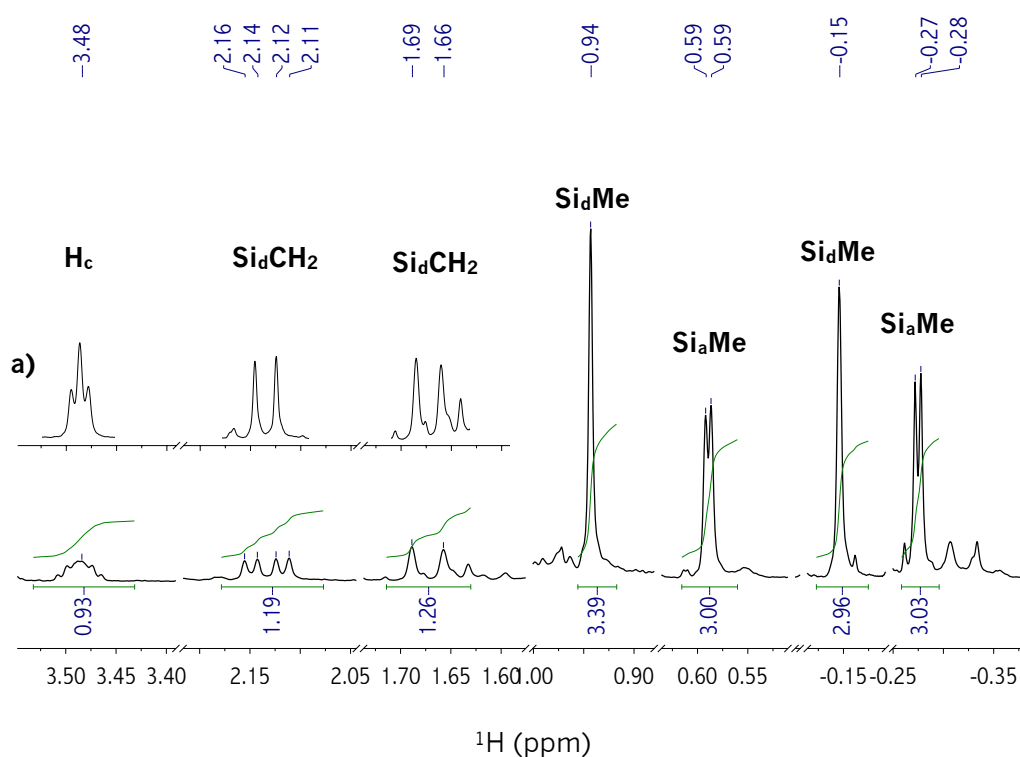
Figura 3.38 RMN de ^1H (400 MHz, 298 K, C_6D_6 ) correspondiente a la reacción del complejo 3-7 frente a 1 eq. de LiBEt_3H en disolución de C_6D_6 a 333 K. Detección espectroscópica del complejo 3-7c . a) RMN ^1H\{^{31}P\} (400 MHz, 298 K, C_6D_6 ).
