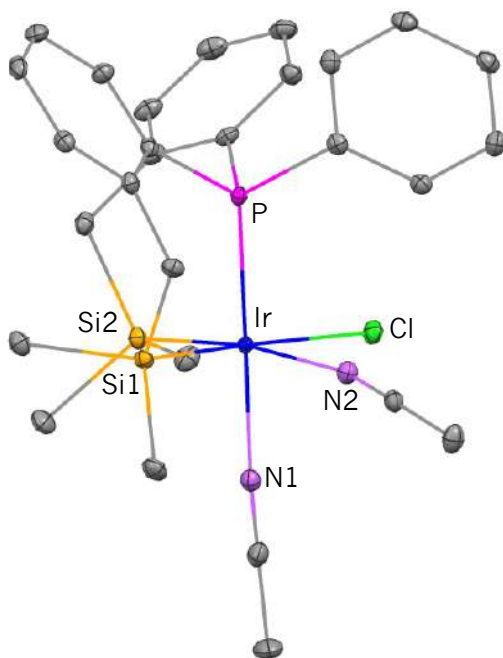
Figura 3.18 Diagramas ORTEP del complejo 3-4b · 2(CD 3 CN) . Elipsoides térmicas al 30 % de probabilidad. Los átomos de hidrógeno y los del disolvente han sido omitidos para mayor claridad.
