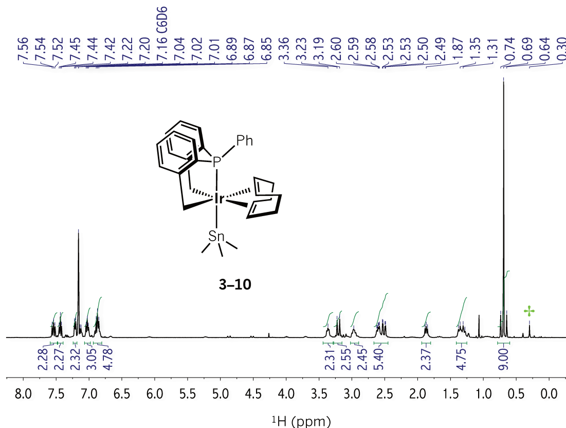
Figura 3.54 Espectro de RMN ^1\text{H} (400 MHz, 298 K, \text{C}_6\text{D}_6 ) del complejo 3-10 . \text{ClSnMe}_3 . 63
