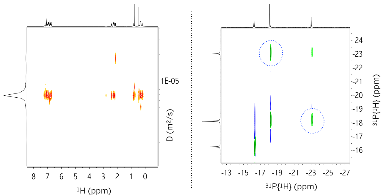
Figura 3.14 Espectros de RMN correspondientes a la reacción “ in situ ” del complejo 3-1a frente a 1 atm de CO en disolución de tol-d 8 en un tubo de RMN de presión. Izquierda: ^1\text{H} -DOSY (600 MHz, 298 K). Derecha: ^{31}\text{P} - ^{31}\text{P} EXSY ( t_m = 150 ms, 233 K).
