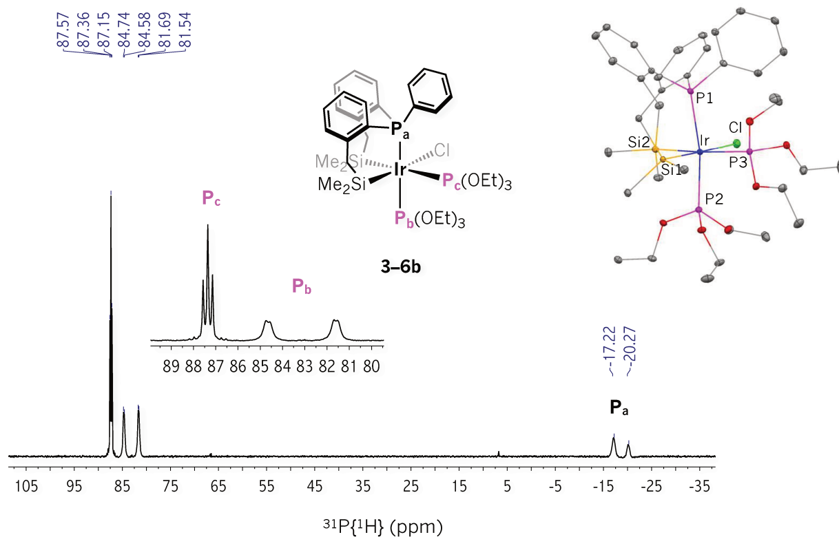
Spectre de RMN 31 P{ 1 H} et structure par diffraction des rayons X du complexe 3-6b.
