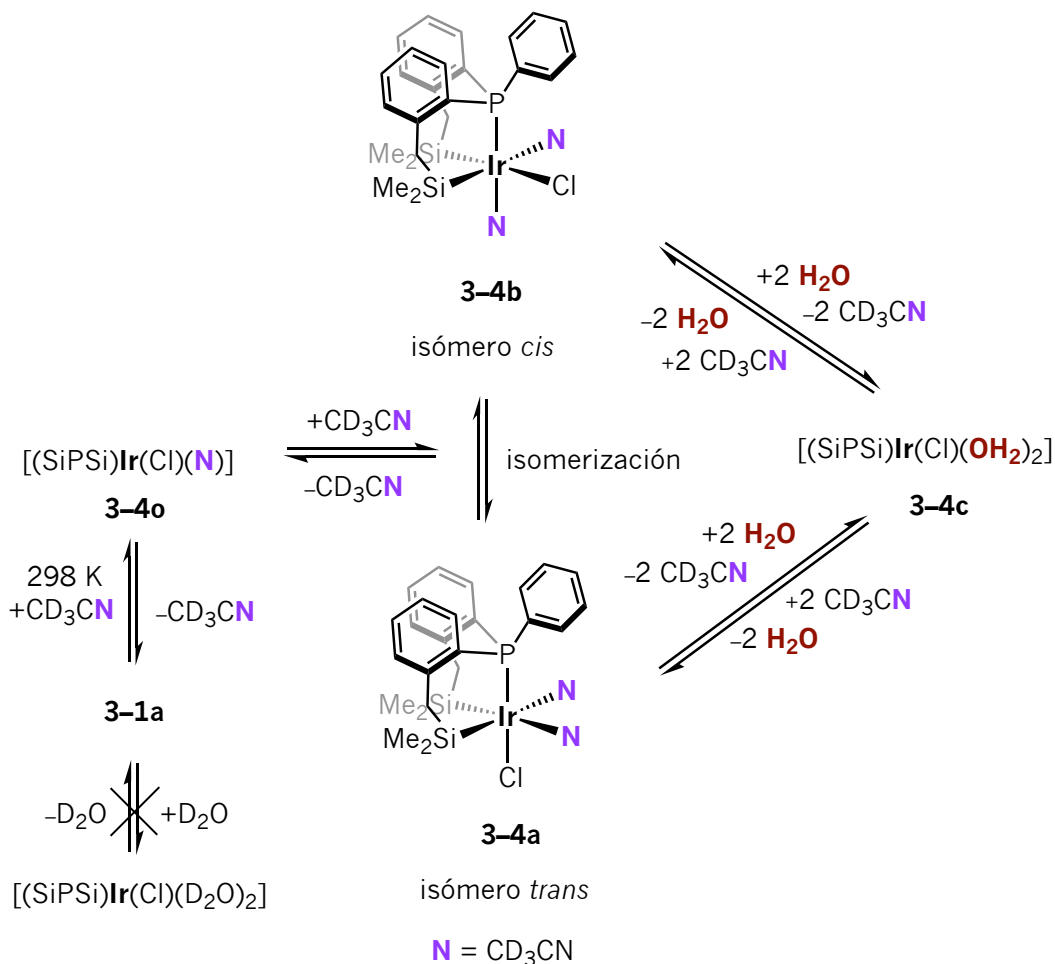
Esquema 3.15 Especies propuestas en equilibrio dinámico presentes en la reacción del complejo 3-1a en disolución de CD_3CN a 298 K.
