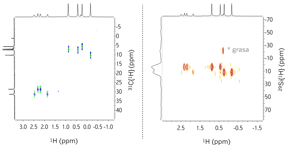
Figura 3.47 RMN de 2D correspondiente al complejo 3-9 . Izquierda: ^1\text{H}-^{13}\text{C}\{^1\text{H}\} HSQC (298 K, \text{C}_6\text{D}_6 ). Derecha: ^1\text{H}-^{29}\text{Si} HMQC (298 K, \text{C}_6\text{D}_6 ).
