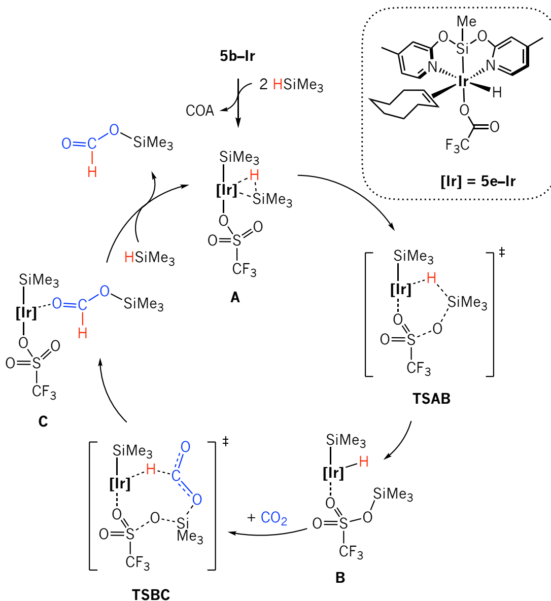
Esquema 1.9 Mecanismo propuesto para la hidrosilación de \text{CO}_2 catalizada por el complejo Ir-[SiNN] 5b-Ir (1 % mol) en ausencia de disolvente. 30
