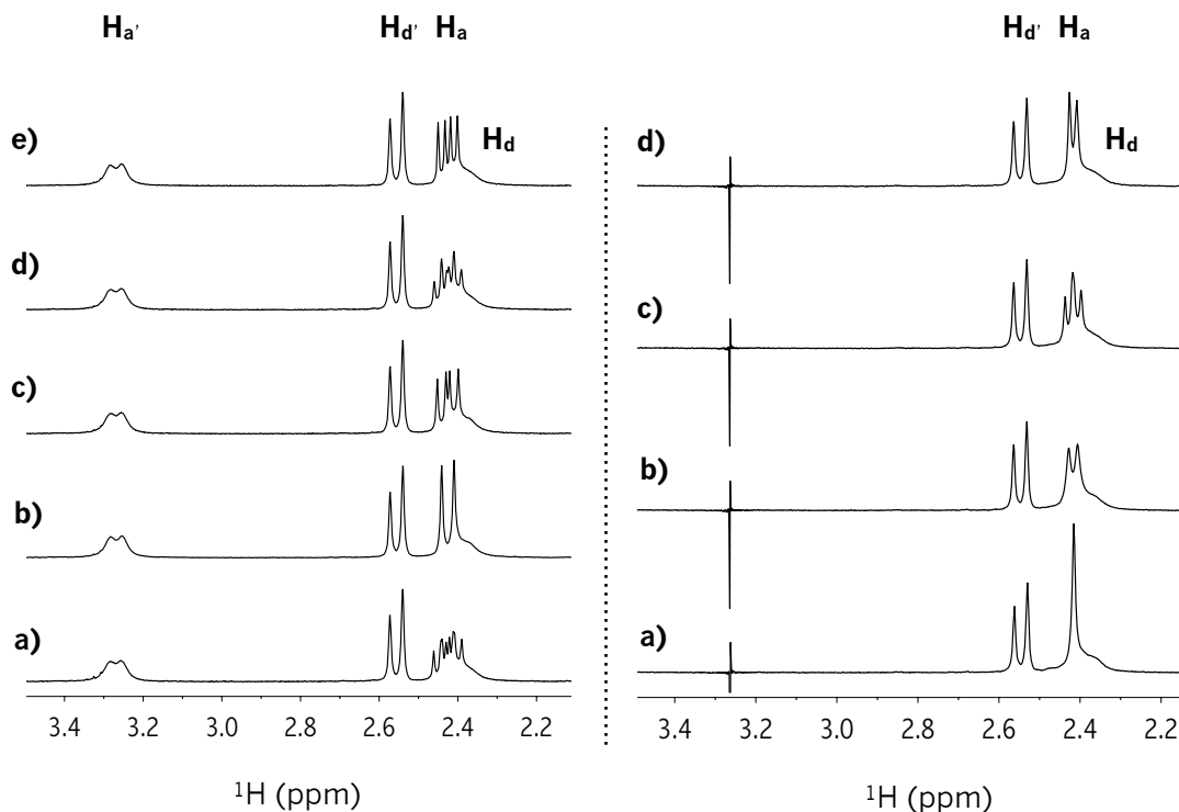
Figura 3.29 RMN (400 MHz, 298 K, \text{C}_6\text{D}_6 ) correspondiente al complejo 3-6b en la región de 2.2 a 3.4 ppm. Izquierda: a) ^1\text{H} b) ^1\text{H}\{^{31}\text{P}\} c) ^1\text{H}\{^{31}\text{P}\} sel: -18.5 \text{ ppm} , \text{P}_a d) ^1\text{H}\{^{31}\text{P}\} sel: 83.1 \text{ ppm} , \text{P}_b e) ^1\text{H}\{^{31}\text{P}\} sel: 87.3 \text{ ppm} , \text{P}_c . Derecha: Espectros irradiados en 3.27 \text{ ppm} : a) ^1\text{H}\{^{31}\text{P}\} b) ^1\text{H}\{^{31}\text{P}\} sel: -18.5 \text{ ppm} , \text{P}_a c) ^1\text{H}\{^{31}\text{P}\} sel: 83.1 \text{ ppm} , \text{P}_b d) ^1\text{H}\{^{31}\text{P}\} sel: 87.3 \text{ ppm} , \text{P}_c .
