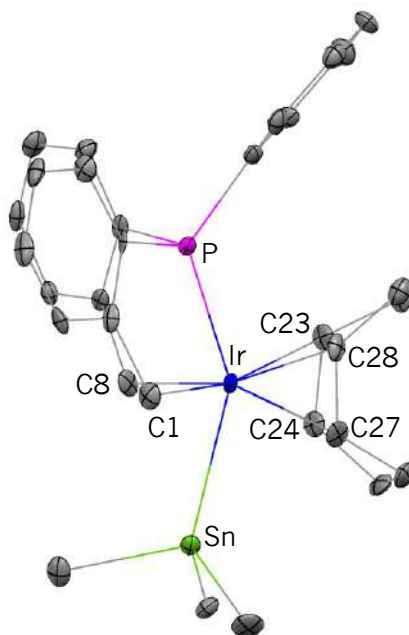
Figura 3.52 Diagrama ORTEP correspondiente al complejo 3-10 . Elipsoides térmicas al 50 % de probabilidad. Los átomos de hidrógeno han sido omitidos para mayor claridad.
