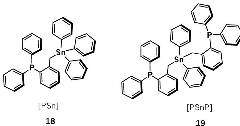
Figura 3.49 Ligandos estanilfosfinas bi- y tridentadas [PSn] 18 y [PSnP] 19 sintetizadas en nuestro grupo de investigación. 55
