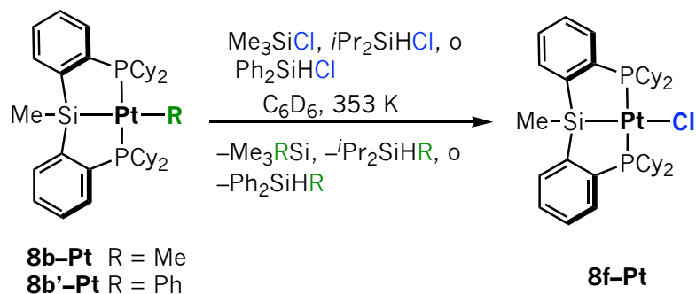
Esquema 1.18 Activación de enlaces Si-Cl de hidrosilanos por los complejos de Pt^{II} 8b-Pt y 8b'-Pt . 67
