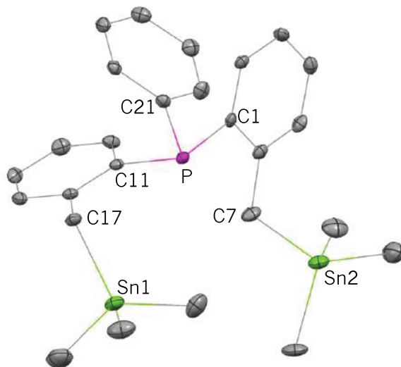
Figura 3.48 Diagrama ORTEP del ligando dibencilistanilfosfina [\text{SnPSn}] L2 . Elipsoides térmicos al 50 % de probabilidad. Los átomos de hidrógeno han sido omitidos para mayor claridad.
