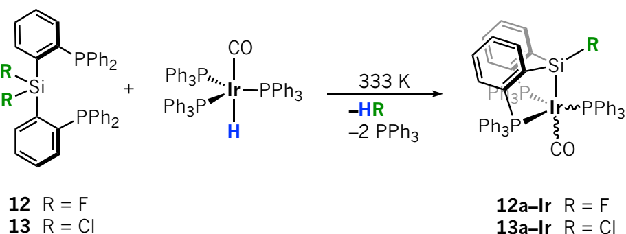
Esquema 1.16 Activación de enlaces Si-F y Si-Cl por el precursor [Ir(H)(CO)(PPh 3 ) 3 ]. 65, 66
