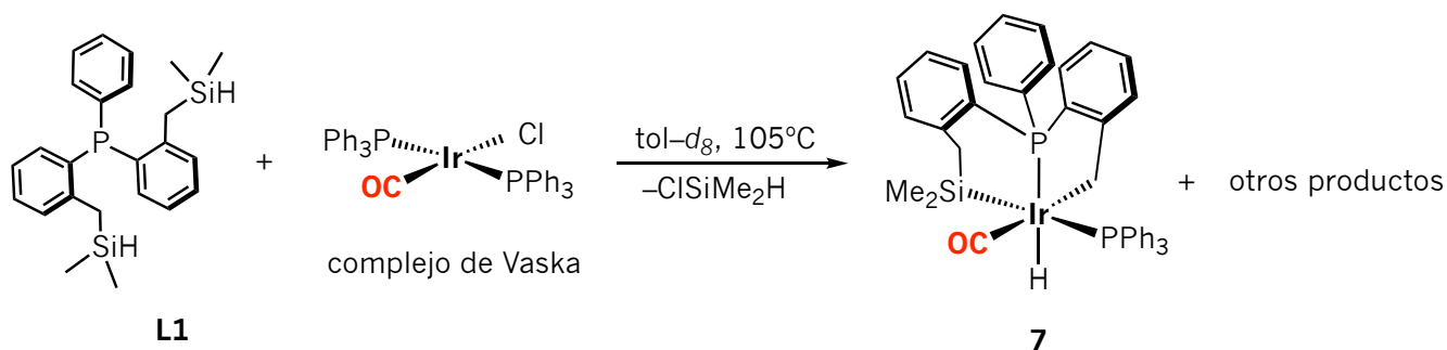
Esquema 3.11 Detección espectroscópica del complejo de Ir III [(CPSi)Ir(H)(CO)(PPh 3 )] 7 . 28
