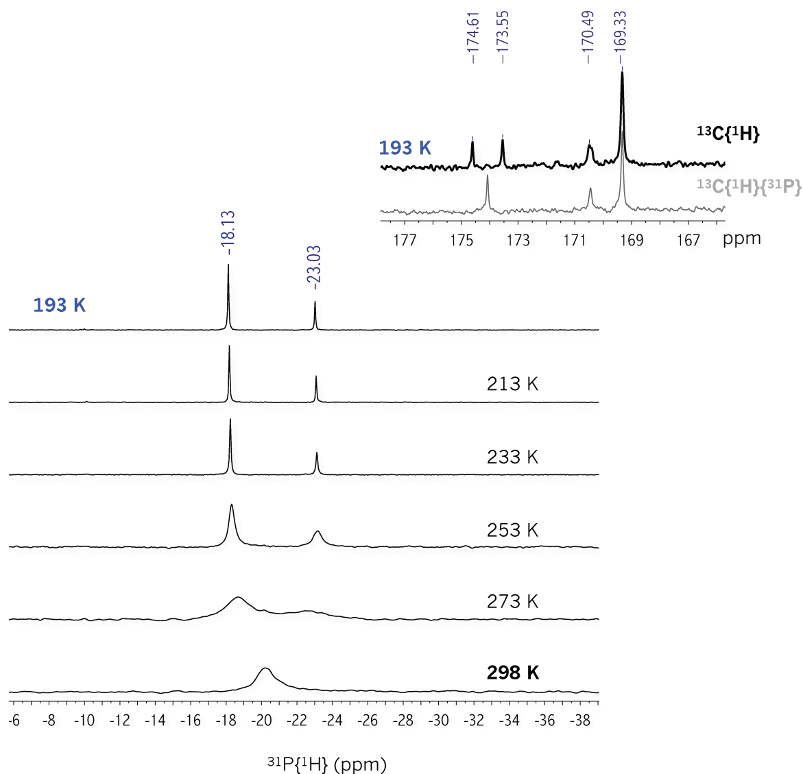
RMN du processus d'isomérisation du complexe 3-2a dans une solution de \text{tol-}d_8 .
