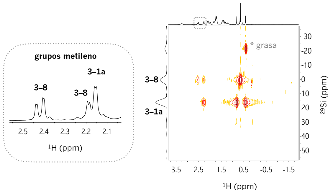
Figura 3.43 Derecha: RMN de 2D ^1\text{H} - ^{29}\text{Si} HMQC (298 K, \text{C}_6\text{D}_6 ) complejo 3-8 y la disociación reversible de la fosfina \text{PCy}_3 que da lugar a 3-1a en disolución de \text{C}_6\text{D}_6 . izquierda : Ampliación en la región de 2.1–2.5 ppm en ^1\text{H} .
