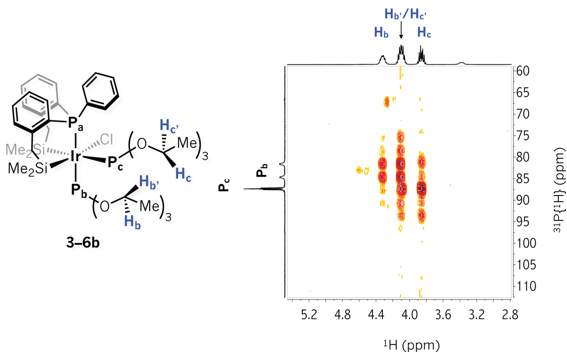
Figura 3A.17 RMN de 2D ^1\text{H} - ^{31}\text{P} HMQC (298 K, \text{C}_6\text{D}_6 ) correspondiente al complejo 3-6b . Correlaciones de los átomos de fósforo \text{P}_b y \text{P}_c con los protones de los grupos metileno de los fosfitos \text{P}(\text{OEt})_3 coordinados.
