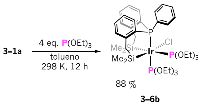
Esquema 3.18 Síntesis del complejo [(\text{PSi}_2)\text{Ir}(\text{Cl})(\text{P}(\text{OEt})_3)_2] cis 3-6b .
