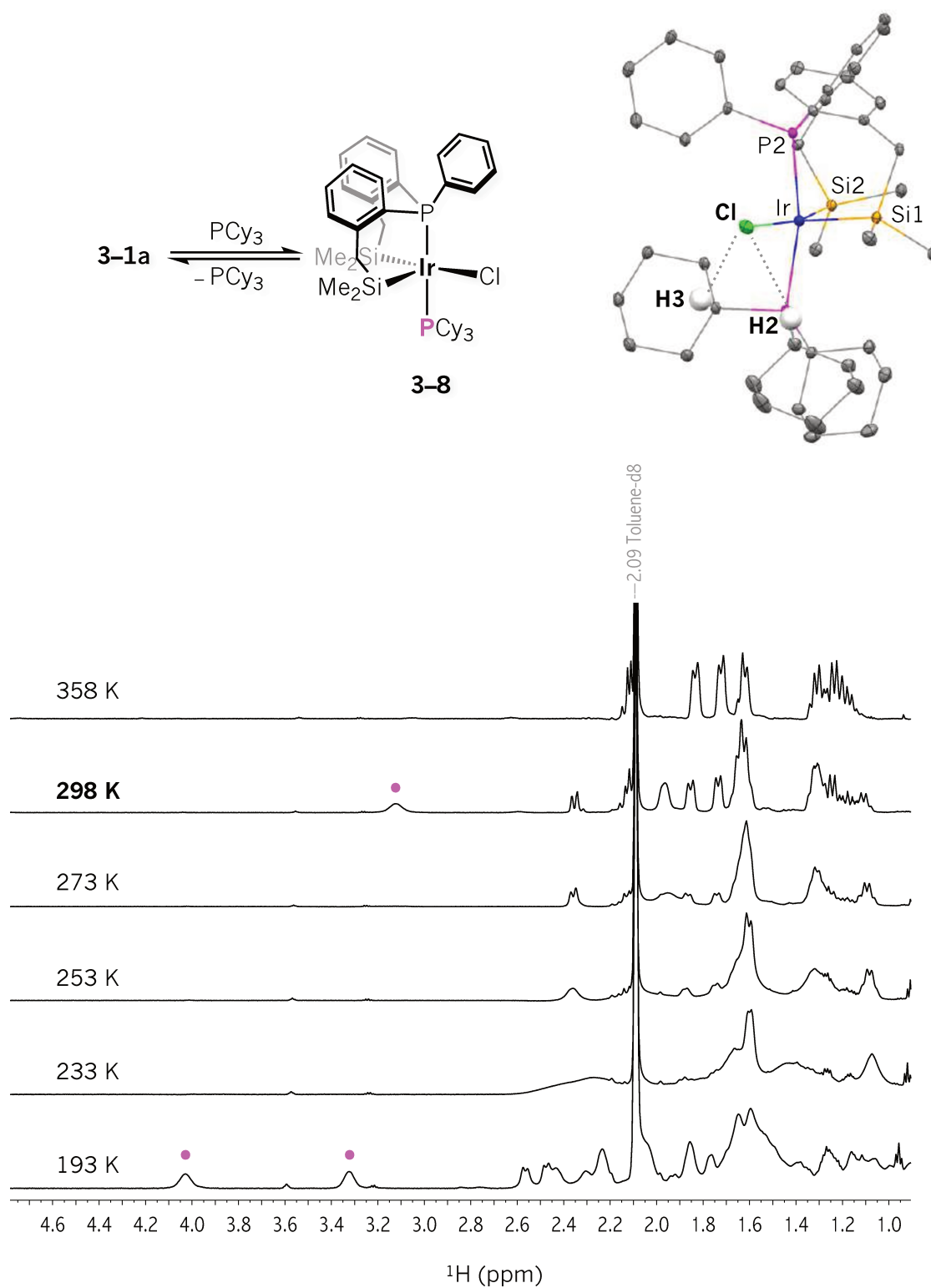
Figura 3A.30 RMN de 1 H (600 MHz, tol- d 8 ) en la región de 1.0–4.6 ppm a diferentes temperaturas correspondiente al complejo 3-8 en disolución de tol- d 8 . Detección espectroscópica de los complejos 3-8 , 3-1a y PCy 3 . ● H2 y H3 del complejo 3-8 .
