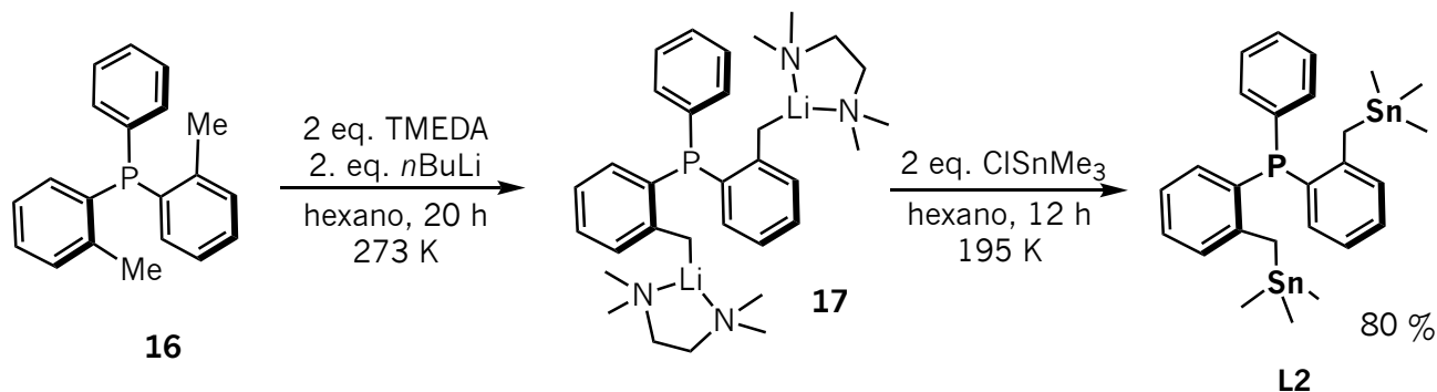
Esquema 3.29 Síntesis del ligando tridentado dibencilestanilfosfina [\text{SnPSn}] L2 .
