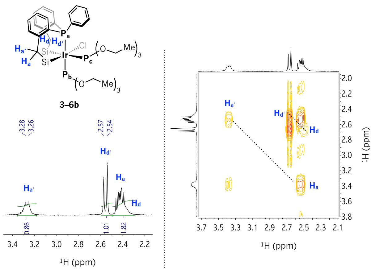
Figura 3.28 RMN correspondiente al complejo 3-6b . Izquierda: ^1H (400 MHz, 298 K, C_6D_6 ) en la región de 2.2 a 3.4 ppm. Derecha: ^1H - ^1H COSY (298 K, C_6D_6 ).
