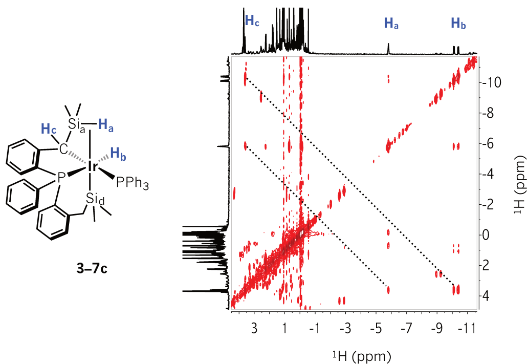
Figura 3A.24 RMN de 2D ^1\text{H} - ^1\text{H} COSY (298 K, C 6 D 6 ) correspondiente a la reacción del complejo 3-7 frente a 1 eq. de LiBEt 3 H en disolución de C 6 D 6 a 333 K. Detección espectroscópica del complejo 3-7c .
