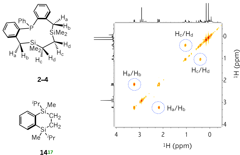
Figura 2.14 Estructuras de los compuestos cíclicos organosililados 2-4 y 1417 y espectro de RMN de 2D ^1\text{H} - ^1\text{H} COSY (298 K, \text{C}_6\text{D}_6 ) en la región de -0.5 a 4.0 ppm correspondiente a la reacción del complejo 2-1 en disolución de \text{C}_6\text{D}_6 frente a 3 atm de etileno en un tubo de RMN de presión. Detección espectroscópica del compuesto 2-4 . Se enfatiza la correlación de los protones \text{H}_a/\text{H}_b y \text{H}_c/\text{H}_d de este último.
