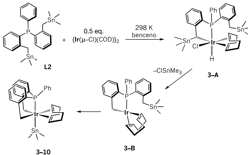
Esquema 3.31 Mecanismo propuesto para la formación del complejo heterobimetálico \text{Ir}^{\text{III}}\text{-Sn}^{\text{IV}} bisciclometalado [(\text{CPC})\text{Ir}(\text{SnMe}_3)(\text{COD})] 3-10 .
