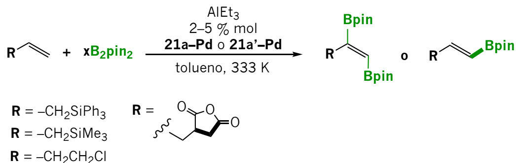
Esquema 1.29 Síntesis selectiva de monoborilalquenos y/o trans 1,2-diborilalquenos a través de la borilación deshidrogenante de alquenos y diboranos catalizada por los complejos 21a-Pd y 21a'-Pd . 80
