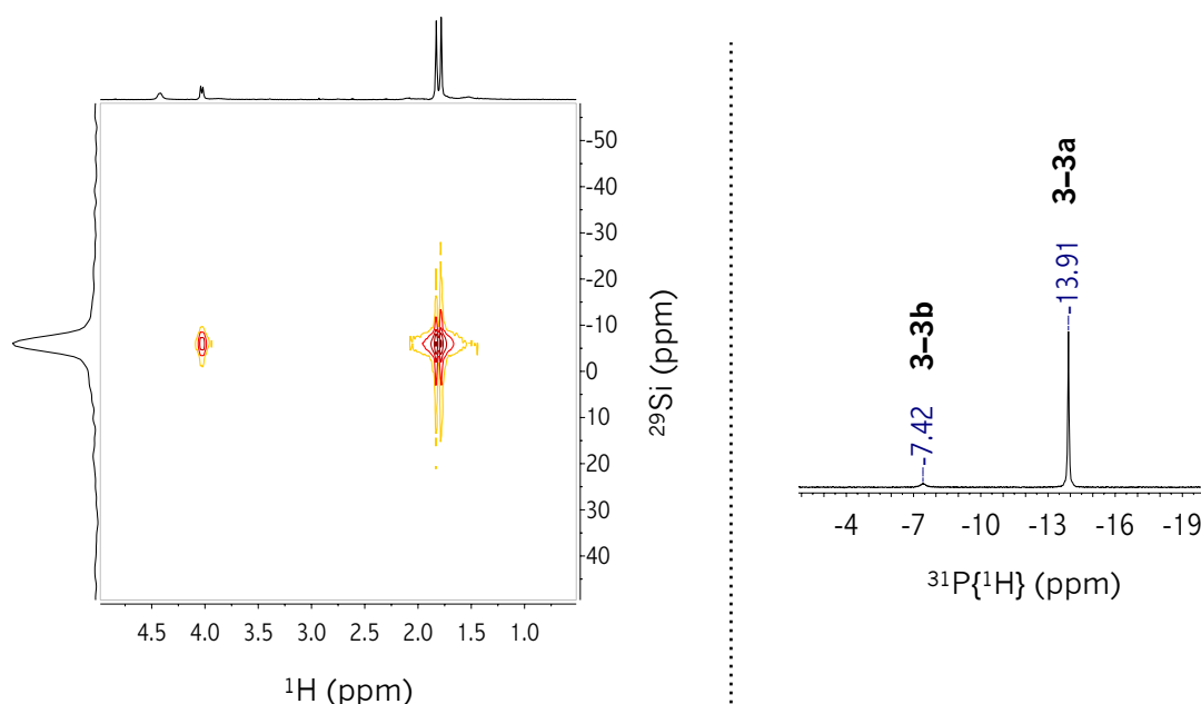
Figura 3.17 RMN correspondiente a la reacción del complejo 3-1a en disolución de piridina- d_5 . Derecha: ^1\text{H} - ^{29}\text{Si} HMQC (298 K, piridina- d_5 ) (Detección espectroscópica del complejo 3-3a ). Izquierda: ^{31}\text{P}\{^1\text{H}\} (161.9 MHz, 298 K, piridina- d_5 ) (Detección espectroscópica del complejo 3-3a y 3-3b ).
