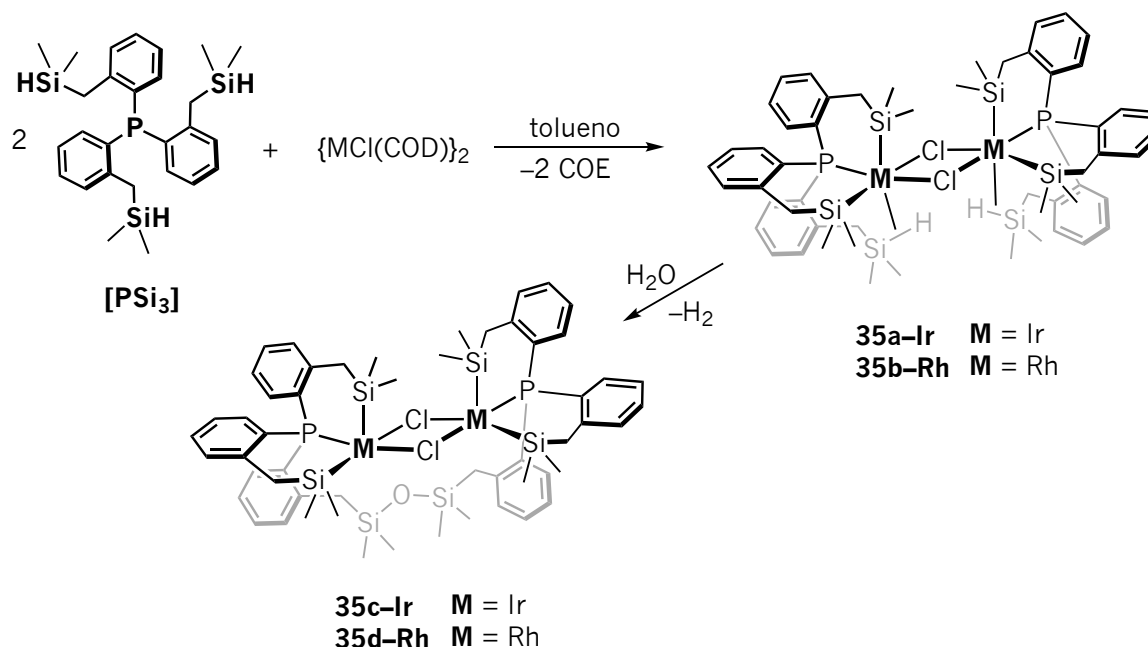
Esquema 1.44 Síntesis de complejos de Ir III y Rh III con enlaces agósticos M-η 2 -(SiH) 35a-Ir y 35b-Rh ; y siloxanos puente 35c-Ir y 35d-Rh a partir del ligando [PSi 3 ] frente a los precursores metálicos \{MCl(COD)\}_2 . 98
