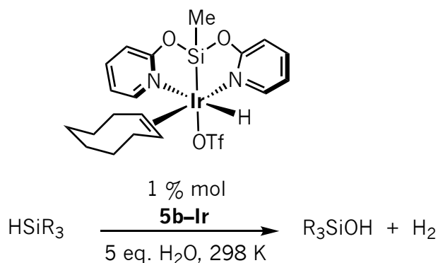
Esquema 1.8 Formación de silanoles y liberación de \text{H}_2 a través de la hidrólisis de silanos catalizada por el complejo \text{Ir}[\text{SiNN}] 5b-Ir . 42
