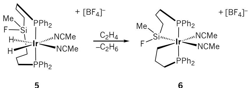
Esquema 3.10 Activación del enlace C–Si del carbono metilénico del ligando [bPSi F ] en el complejo 5 y formación del derivado 6 . 27
