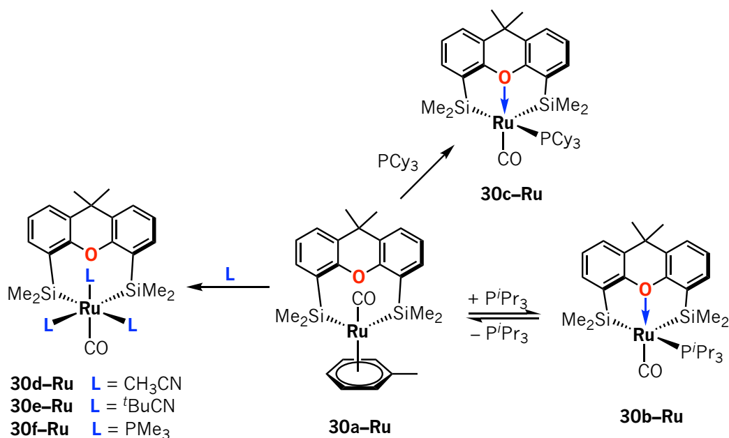
Esquema 1.35 Síntesis de complejos de Ru^{II} con el bis-silil ligando “xantsil”. 88,89
