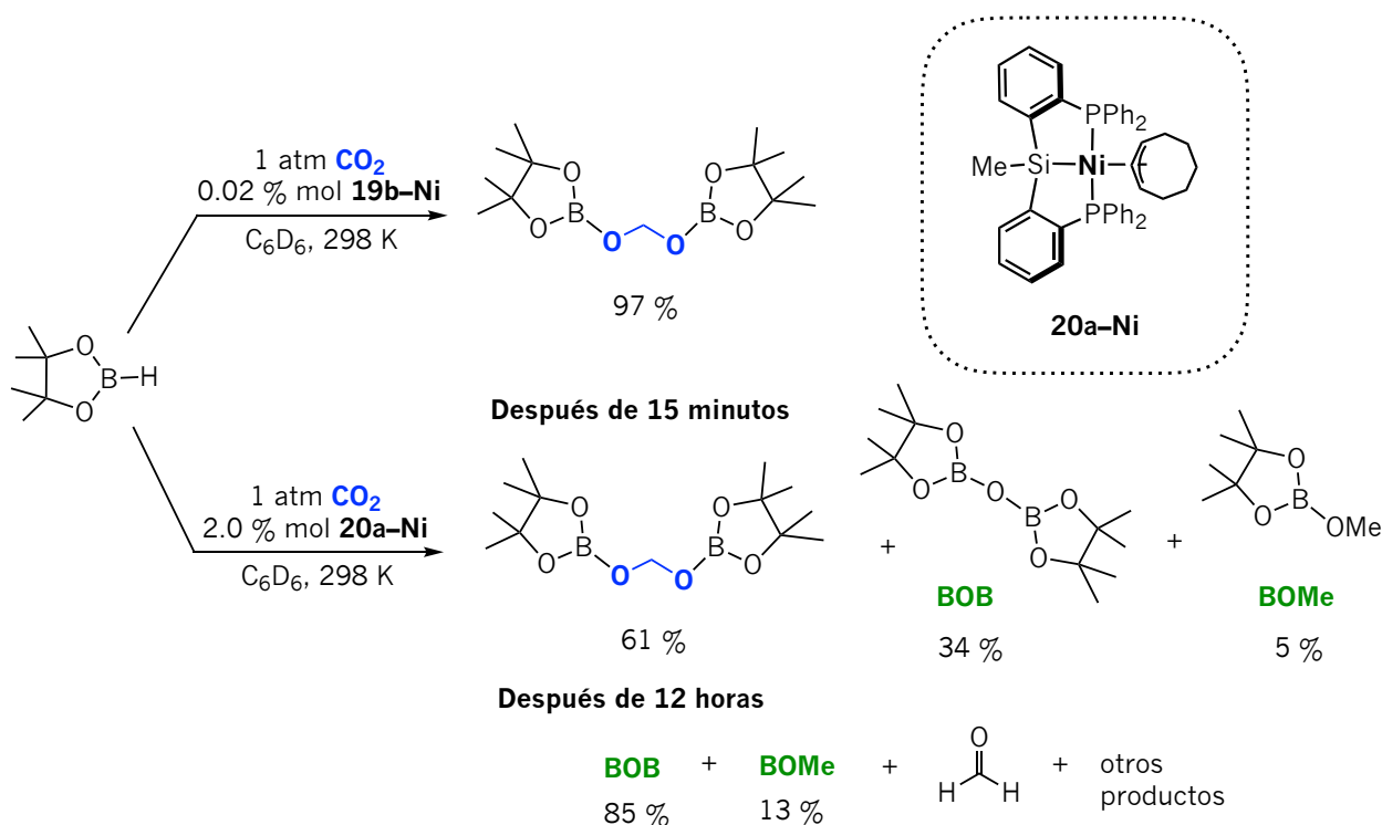
Esquema 1.27 Hidroboración de CO 2 con HBpin catalizada por los complejos 19b-Ni y 20a-Ni . 57a
