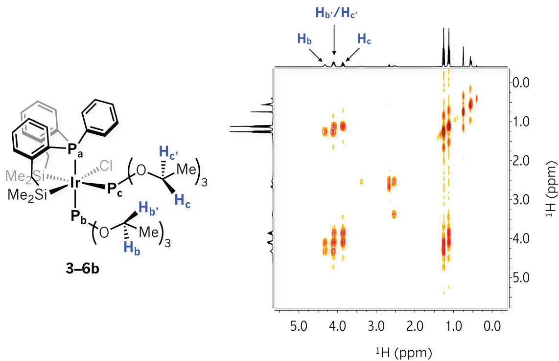
Figura 3A.18 RMN de 2D ^1\text{H} - ^1\text{H} COSY (298 K, \text{C}_6\text{D}_6 ) correspondiente al complejo 3-6b . Correlaciones entre los protones de los grupos metilenos y metilos de los fosfitos \text{P}(\text{OEt})_3 coordinados.
