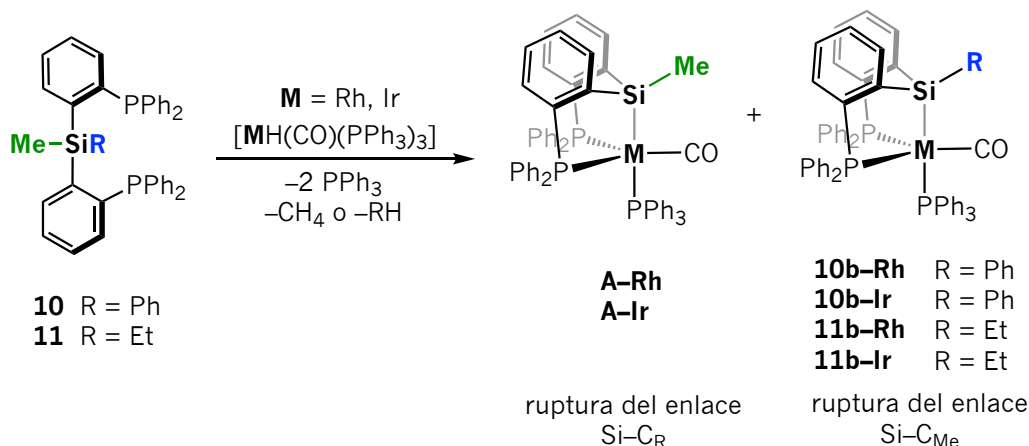
Esquema 1.15 Activación de enlaces Si-C(sp 2 ) y Si-C(sp 3 ) de los ligandos SiMePh{(o-C 6 H 4 )PPh 2 } 2 10 y SiMe(CH 2 CH 3 ){(o-C 6 H 4 )PPh 2 } 2 11 por precursores metálicos de Rh I e Ir I .
