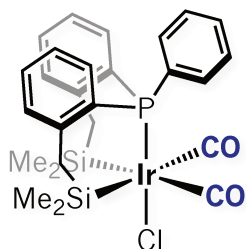
3-2a isómero trans
