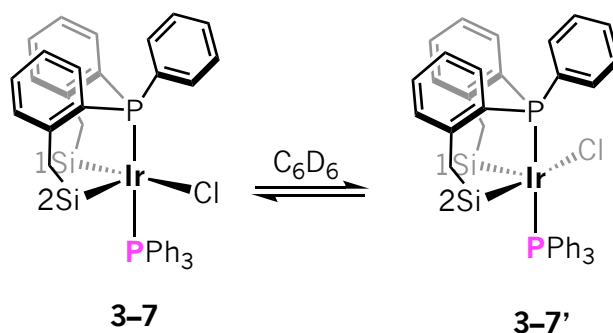
Esquema 3.20 Equilibrio dinámico propuesto para el complejo 3-7 en disolución de \text{C}_6\text{D}_6 .
