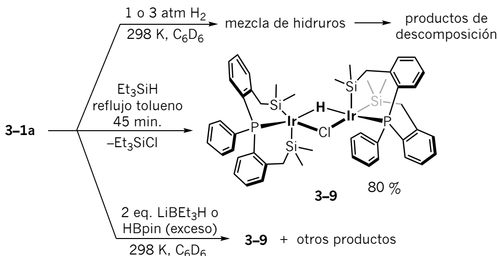
Esquema 3.28 Reactividad del complejo 3-1a frente a diferentes fuentes de hidrógeno.
