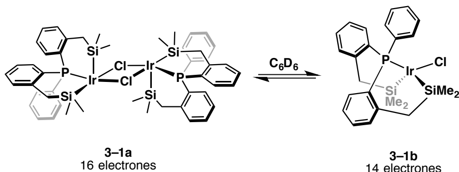
Esquema 3.4 Disociación en solución de C_6D_6 del complejo dinuclear 3-1a al complejo mononuclear 3-1b .
