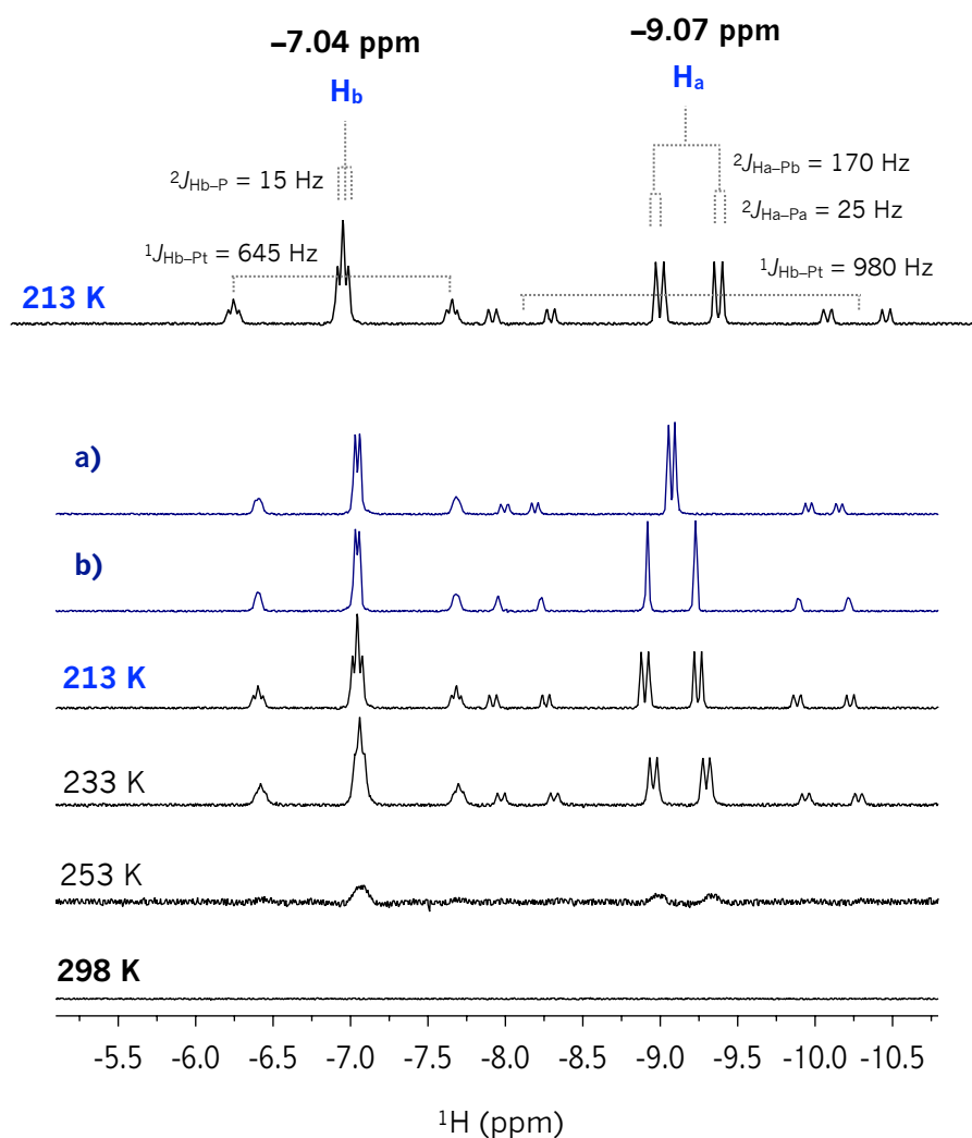
Figura 2.5 Espectros de RMN de ^1\text{H} (500 MHz, \text{tol-}d_8 ) en la región de hidruros metálicos a diferentes temperaturas correspondientes a la reacción del complejo 2-1 frente a 3 atm de \text{H}_2 en \text{tol-}d_8 en un tubo de RMN de presión y ampliación del espectro a 213 K. Detección espectroscópica del complejo 2-2 . a) ^1\text{H}\{^{31}\text{P}\}\text{sel} : -16.2 ppm y b) ^1\text{H}\{^{31}\text{P}\}\text{sel} : -3.5 ppm a 213 K.
