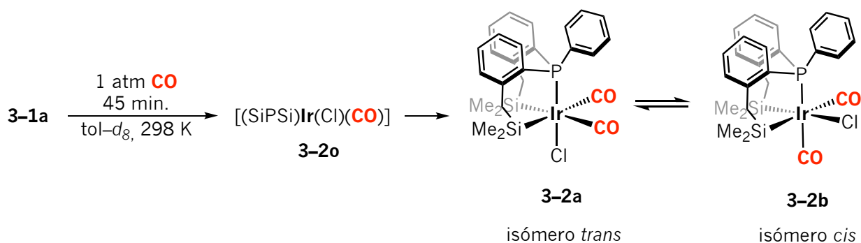
Esquema 3.8 Reacción “ in situ ” del complejo 3-1a frente a 1 atm de CO en disolución de tol-d 8 .
