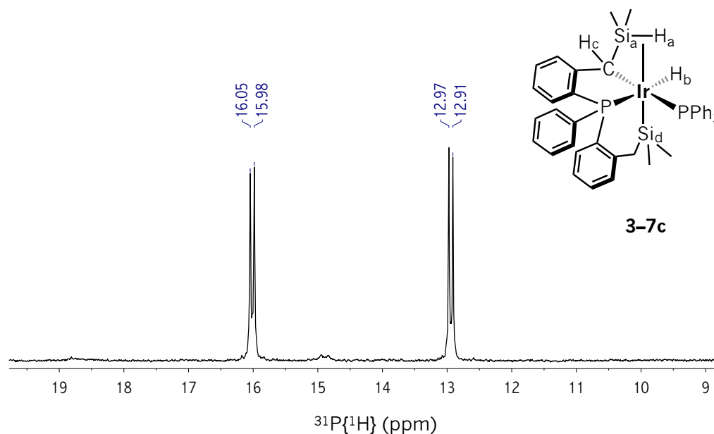
Figura 3.36 RMN de ^{31}\text{P}\{^1\text{H}\} (161.9 MHz, 298 K, \text{C}_6\text{D}_6 ) correspondiente a la reacción del complejo 3-7 frente a 1 eq. de \text{LiBEt}_3\text{H} en disolución de \text{C}_6\text{D}_6 a 333 K. Detección espectroscópica del complejo 3-7c .
