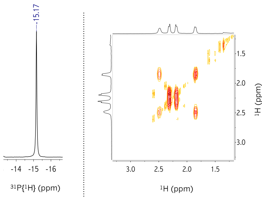
Figura 3.46 RMN correspondiente al complejo 3-9 . Izquierda: ^{31}\text{P}\{^1\text{H}\} (243.0 MHz, 298 K, \text{C}_6\text{D}_6 ). Derecha: ^1\text{H} - ^1\text{H} COSY en la región de 1.0–3.5 ppm.
