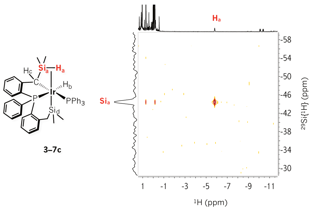
Figura 3A.25 RMN de 2D ^1\text{H} - ^{29}\text{Si} HMQC (298 K, C 6 D 6 ) correspondiente a la reacción del complejo 3-7 frente a 1 eq. de LiBEt 3 H en disolución de C 6 D 6 a 333 K. Detección espectroscópica del complejo 3-7c .
