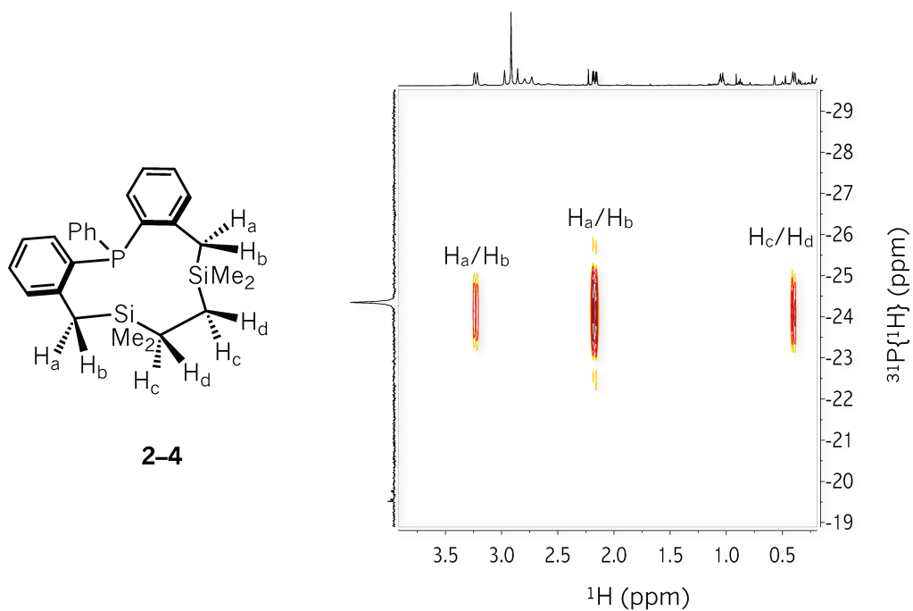
Figura 2A.9. Espectro de RMN de ^1\text{H} (500 MHz, 358 K , \text{tol-}d_8 ) correspondiente a la reacción del complejo 2-1 frente a 3 atm de CO en \text{tol-}d_8 llevada a cabo en un tubo de RMN de presión. Detección espectroscópica de la isomerización cis/trans 2-3b/2-3a .
