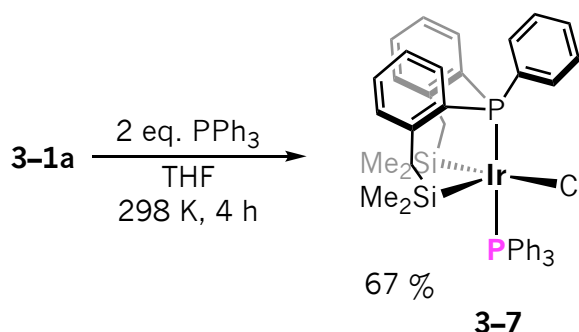
Esquema 3.19 Síntesis del complejo [(\text{SiPSi})\text{Ir}(\text{Cl})(\text{PPh}_3)] 3-7 .
