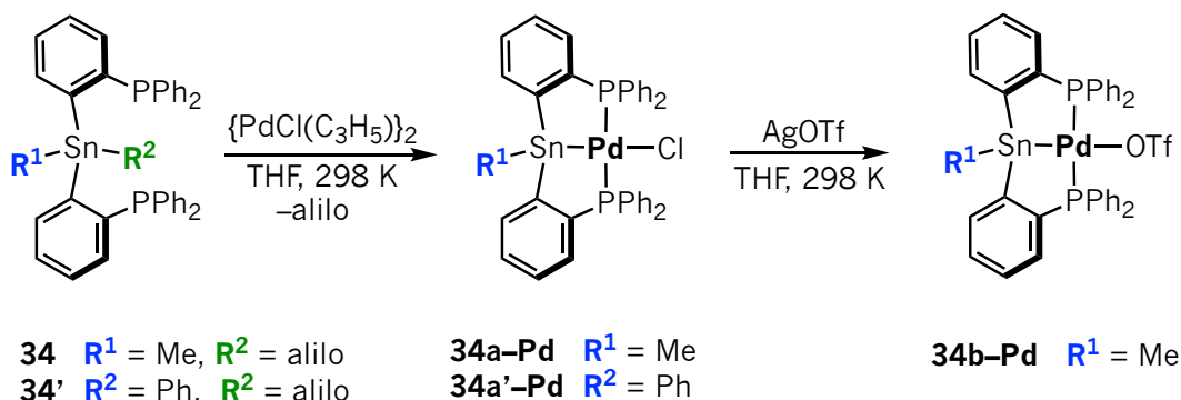
Esquema 1.41 Síntesis de complejos de \text{Pd}^{\text{II}} con ligandos estanilfosfinas [PSnP]. 96
