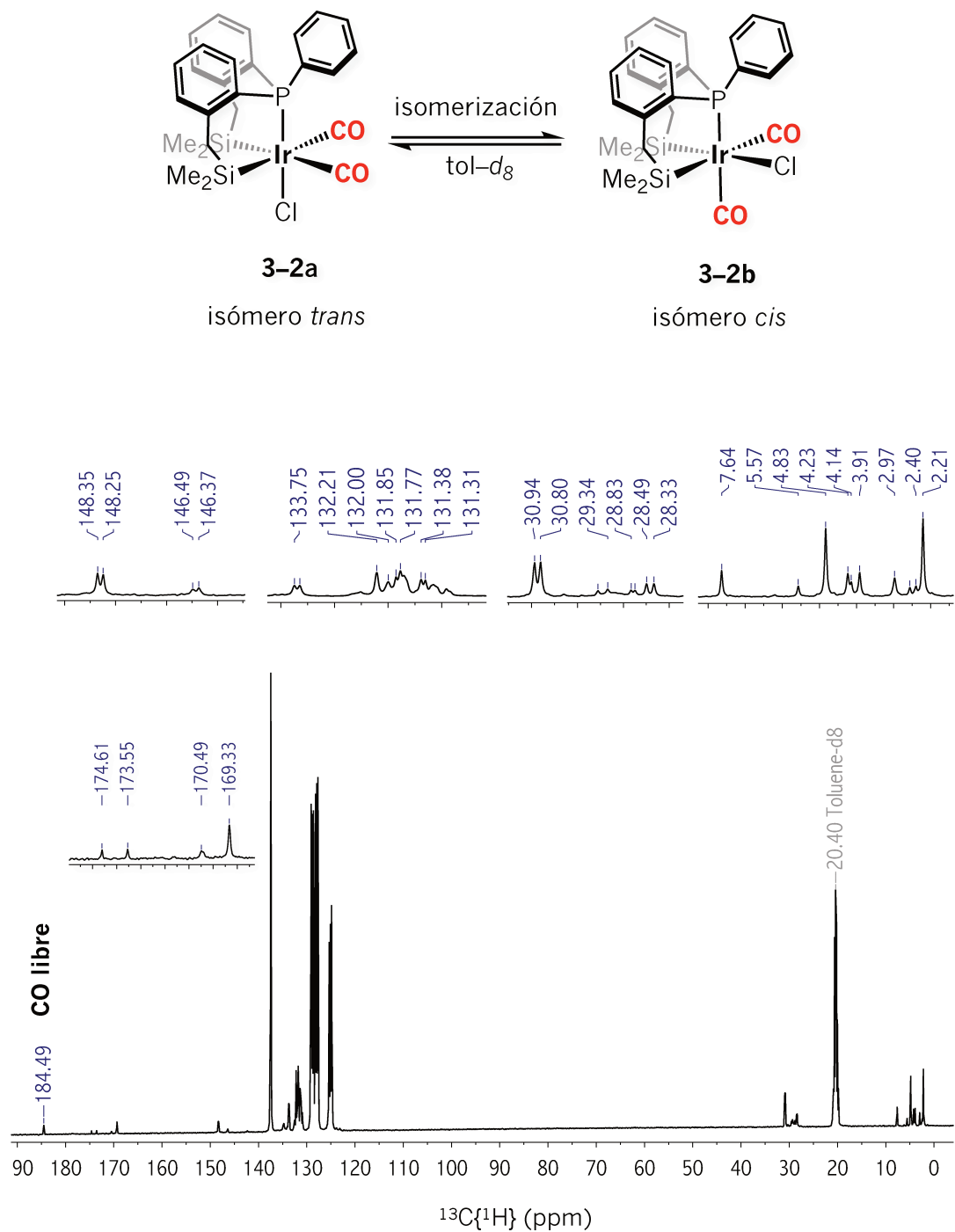
Figura 3A.7 RMN de ^{13}\text{C}\{^1\text{H}\} (100.6 MHz, 298 K, \text{tol-}d_8 ) correspondiente al proceso de isomerización cis/trans 3-2b/3-2a .
