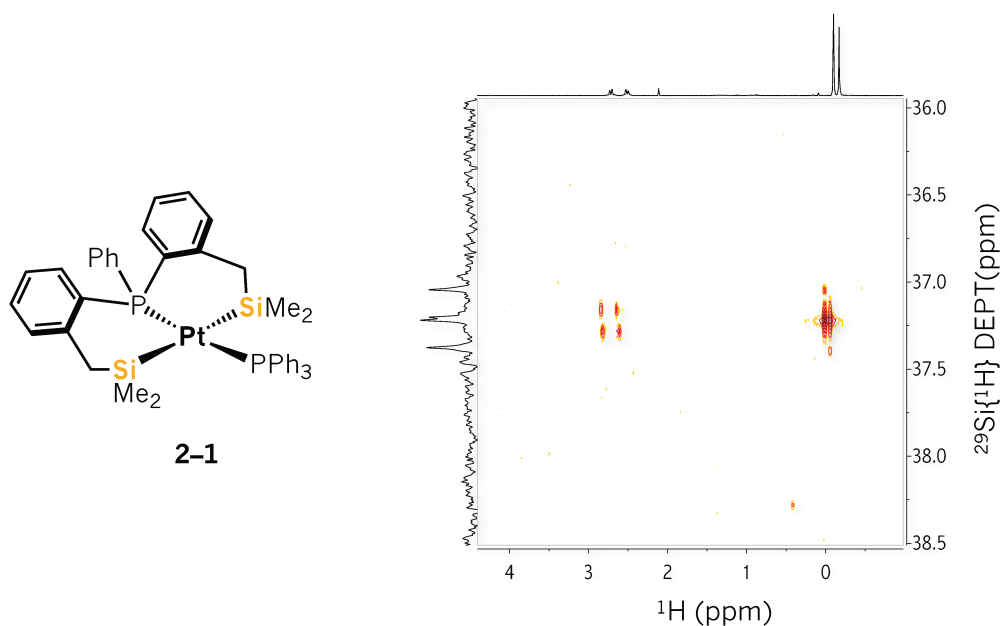
Figura 2A.1. Espectro de RMN de 2D ^1\text{H} - ^{29}\text{Si} HMQC ( \text{C}_6\text{D}_6 , 298 K) correspondiente al complejo 2-1 .
