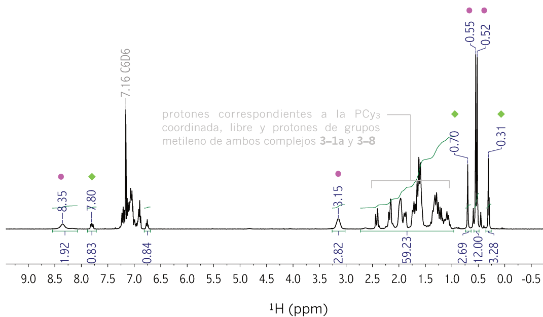
Figura 3A.27 RMN de ^1\text{H} (600 MHz, 298 K, \text{C}_6\text{D}_6 ) correspondiente al complejo 3-8 en disolución de \text{C}_6\text{D}_6 . Detección espectroscópica de los complejos 3-8 , 3-1a y \text{PCy}_3 . ● 3-8 ◆ 3-1a
