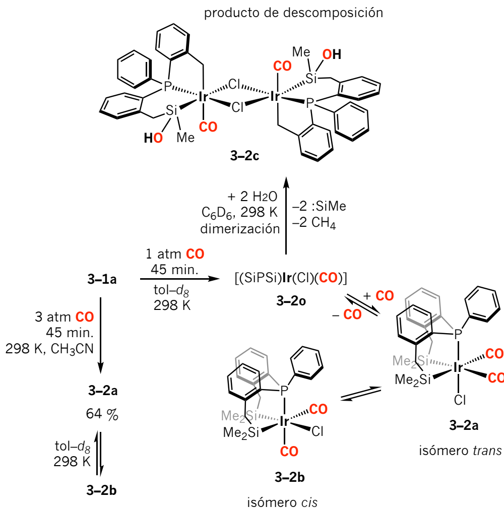
Esquema 3.12 Reactividad del complejo \{[\text{SiPSi}]\text{Ir}(\mu\text{-Cl})_2\} 3-1a frente a CO.
