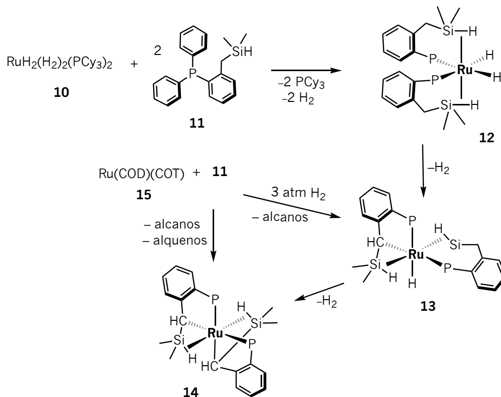
Esquema 3.23 Activación de enlaces C–H y Si–H en complejos de rutenio enlazados al ligando bidentado [PSi]. 44 Los grupos fenilo del átomo de fósforo han sido omitidos para mayor claridad.
