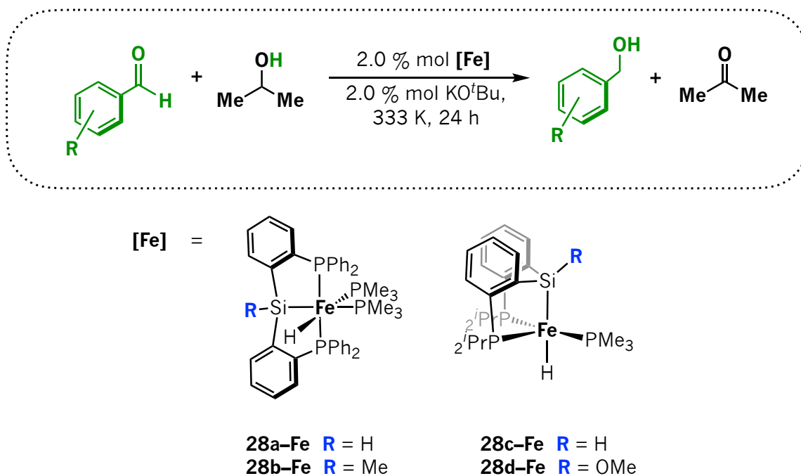
Esquema 1.33 Hidrogenación por transferencia de aldehídos catalizada por complejos de hierro 28a-Fe , 28b-Fe , 28c-Fe y 28d-Fe . 8c
