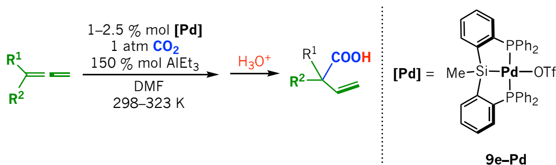
Esquema 1.23 Síntesis de ácidos carboxílicos \beta,\gamma -insaturados a partir de la carboxilación de alenos catalizada por el complejo Pd-[PSiP] 9e-Pd . 71
