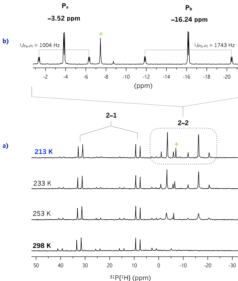
Figura 2.9 Espectros de RMN correspondientes a la reacción del complejo 2-1 frente a 3 atm de \text{H}_2 en \text{tol-}d_8 en un tubo de RMN de presión. Detección espectroscópica de los complejos 2-1 y 2-2 . a) ^{31}\text{P}\{^1\text{H}\} (202.4 MHz, \text{tol-}d_8 ) a diferentes temperaturas. + Denota \text{PPh}_3 libre que proviene del complejo 2-1 como una impureza. b) Ampliación del sistema de dobletes del complejo 2-2 a 213 K.
