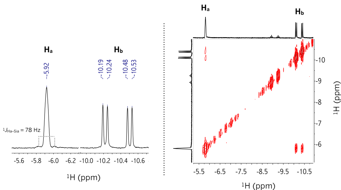
Figura 3.37 RMN correspondiente a la reacción del complejo 3-7 frente a 1 eq. de \text{LiEt}_3\text{H} en disolución de \text{C}_6\text{D}_6 a 333 K. Detección espectroscópica del complejo 3-7c . Izquierda: Señales de los átomos \text{H}_a y \text{H}_b en el espectro de ^1\text{H} (400 MHz, 298 K, \text{C}_6\text{D}_6 ). Derecha: ^1\text{H}\text{-}^1\text{H} COSY (298 K, \text{C}_6\text{D}_6 ) enfatizando la correlación entre dichos protones.
