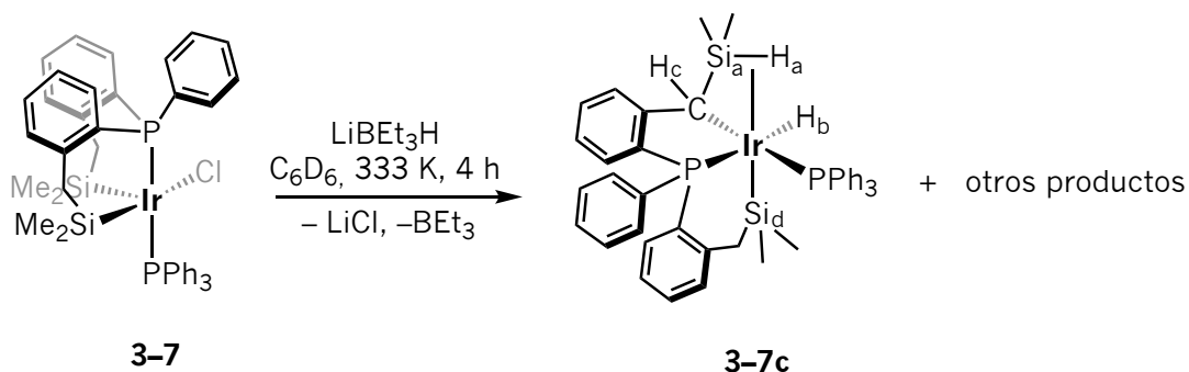
Esquema 3.22 Reacción del complejo 3-7 frente a 1 eq. de \text{LiBEt}_3\text{H} en disolución de \text{C}_6\text{D}_6 a 333 K.
