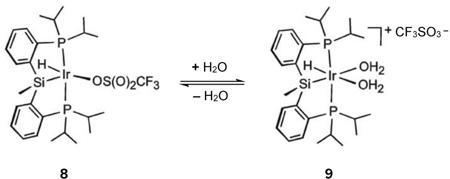
Esquema 3.16 Formación del aducto 9 en presencia de trazas de agua en equilibrio dinámico con el derivado 8 . 9p
