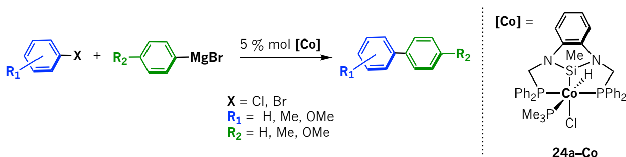
Esquema 1.31 Acoplamiento C-C o reacción de Kumada catalizada por el hidruro de Co^{III} 24a-Co . 7b
