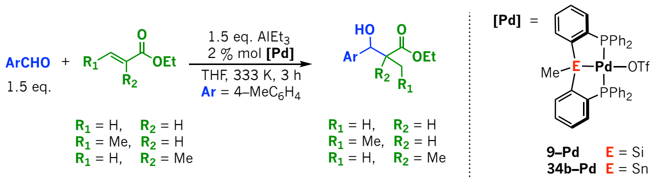
Esquema 1.42 Acoplamiento carbono-carbono de ésteres \alpha,\beta -insaturados y aldehídos a través de la reacción aldólica catalizada por complejos de \text{Pd}^{\text{II}} con ligandos [PEP] \text{E} = \text{Si}, \text{Sn} . 96
