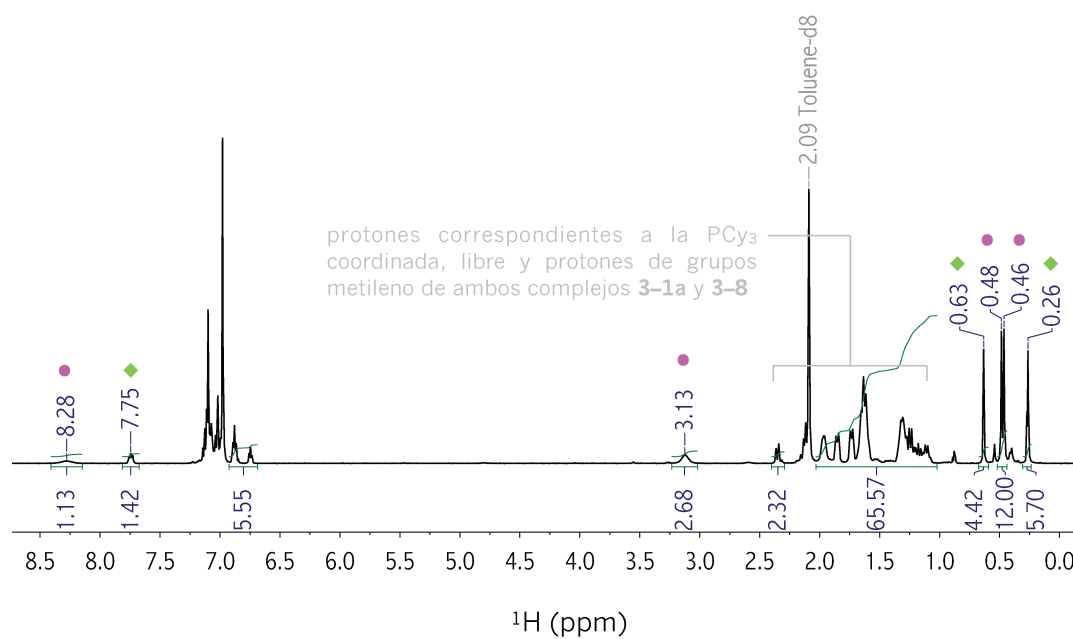
Figura 3A.28 RMN de 1 H (600 MHz, 298 K, tol- d 8 ) correspondiente al complejo 3-8 en disolución de tol- d 8 . Detección espectroscópica de los complejos 3-8 , 3-1a y PCy 3 . ● 3-8 ◆ 3-1a
