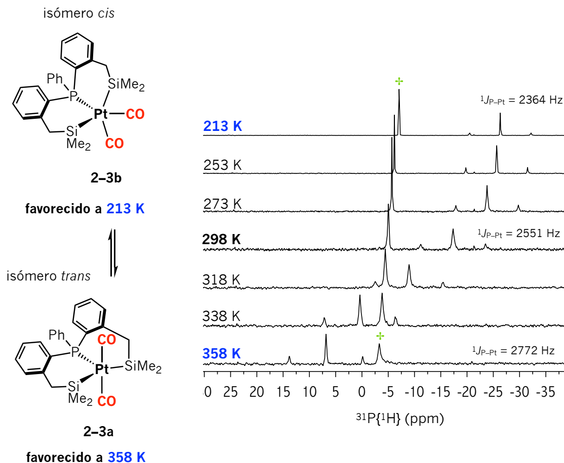
Figura 2.10 Espectros de RMN de ^{31}\text{P}\{^1\text{H}\} (202.4 MHz, \text{tol}-d_8 ) a diferentes temperaturas correspondientes a la reacción del complejo 2-1 frente a 3 atm de CO en \text{tol}-d_8 llevada a cabo en un tubo de RMN de presión. Detección espectroscópica de la isomerización cis/trans 2-3b/2-3a . + Fosfina \text{PPh}_3 libre.
