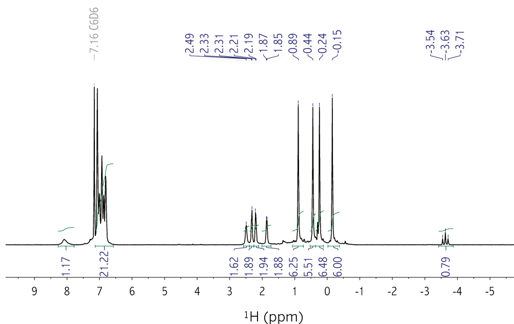
Figura 3.45 RMN de ^1\text{H} (600 MHz, 298 K, \text{C}_6\text{D}_6 ) correspondiente al complejo 3–19 .
