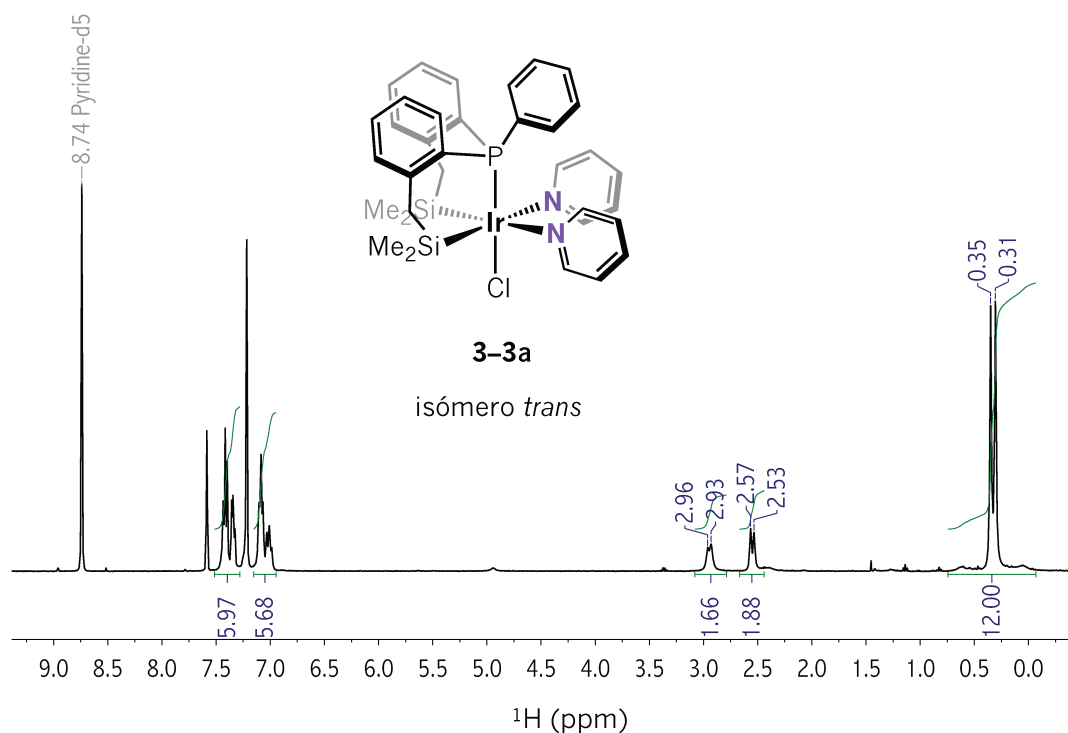
Figura 3.16 RMN de ^1\text{H} (400 MHz, 298 K, piridina- d_5 ) correspondiente a la reacción de 3-1a en disolución de piridina- d_5 a 298 K. Detección espectroscópica de 3-3a .
