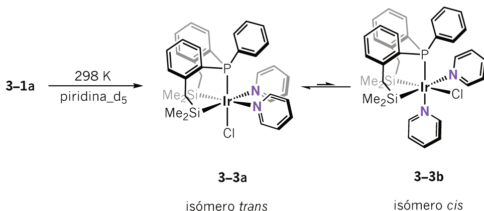
Esquema 3.13 Reacción del complejo 3-1a en disolución de piridina- d_5 a 298 K.
