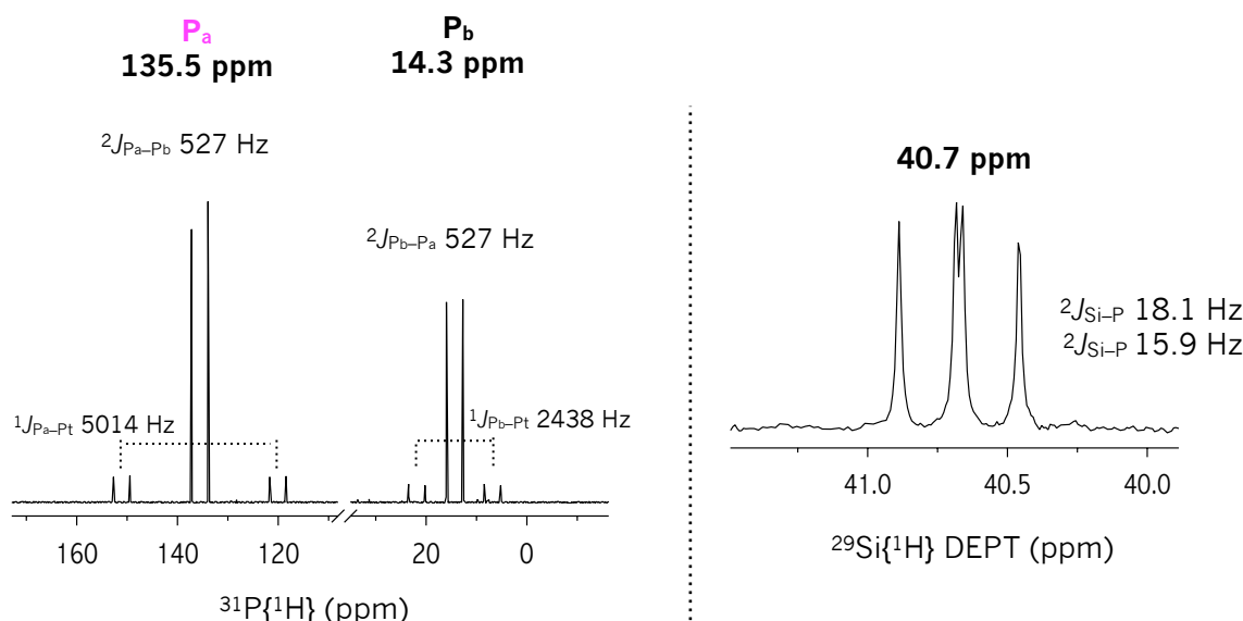
Figura 2.17 Espectros de RMN correspondientes al complejo 2-5 . Izquierda: ^{31}\text{P}\{^1\text{H}\} (161.9 MHz, 298 K, C 6 D 6 ). Derecha: ^{29}\text{Si}\{^1\text{H}\} DEPT (99.4 MHz, 298 K, C 6 D 6 ).
