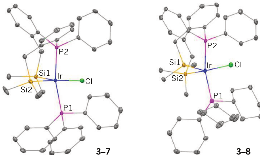
Structure par diffraction des rayons X des complexes 3-7 et 3-8
