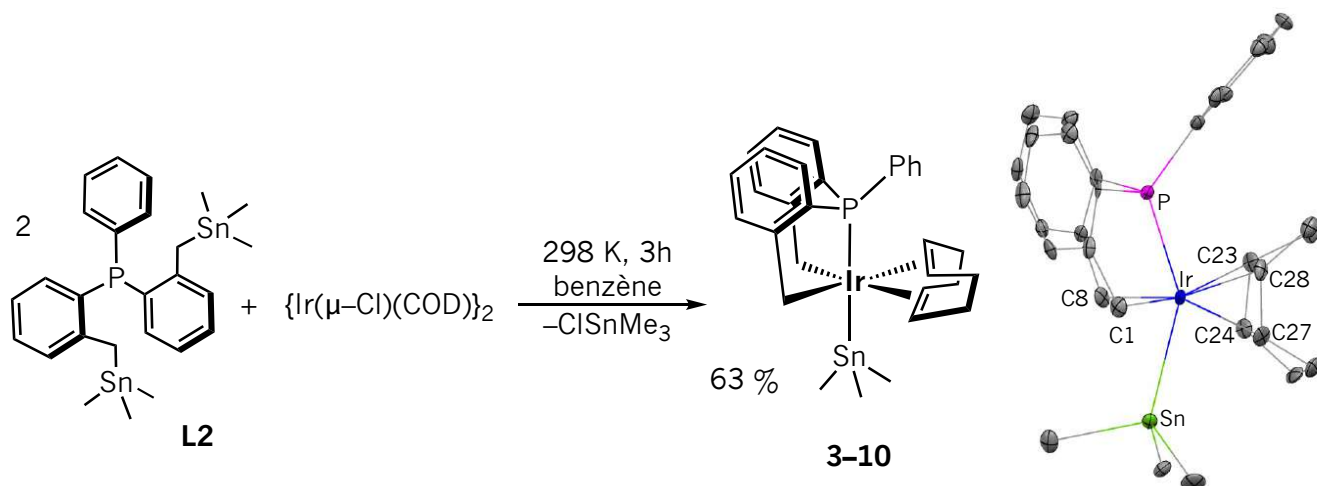
Préparation du composé 3-10 et structure par diffraction des rayons X.
