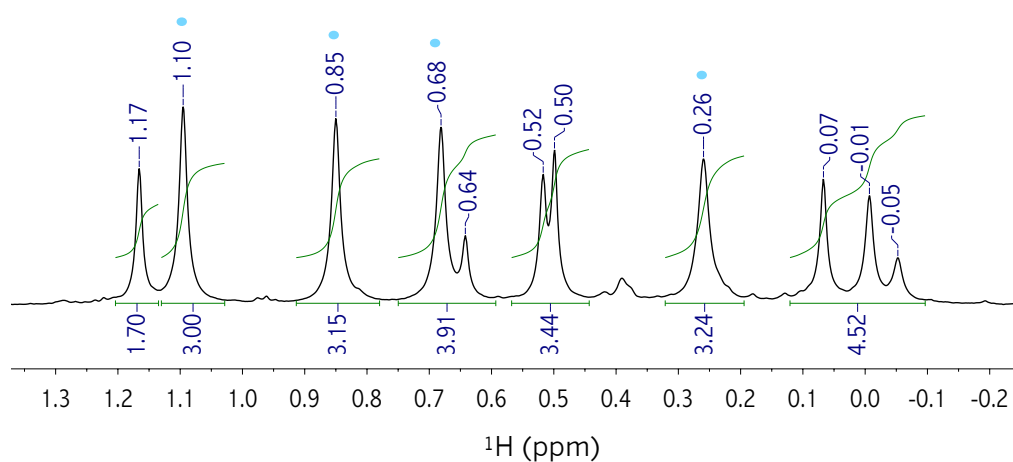
Figura 3.12 RMN de ^1\text{H} (500 MHz, 193 K, \text{tol-}d_8 ) en la región de los grupos metilo correspondiente a la reacción “ in situ ” del complejo 3-1a frente a 1 atm de CO en disolución de \text{tol-}d_8 en un tubo de RMN de presión. • Señales correspondientes al complejo [(\text{SiPSi})\text{Ir}(\text{Cl})(\text{CO})] 3-2o .
