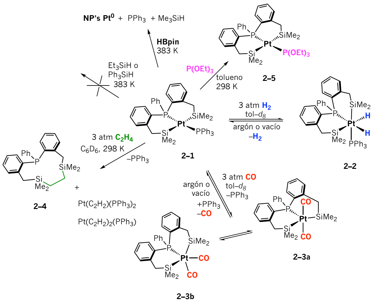
Esquema 2.3 Reactividad del complejo trans - [\text{Pt}(\text{SiP}(\text{SiMe}_2)\text{Ph})(\text{PPh}_3)] 2-1 frente a \text{H}_2 , \text{CO} , \text{C}_2\text{H}_4 , \text{Et}_3\text{SiH} , \text{Ph}_3\text{SiH} , HBpin y \text{P}(\text{OEt})_3 .
