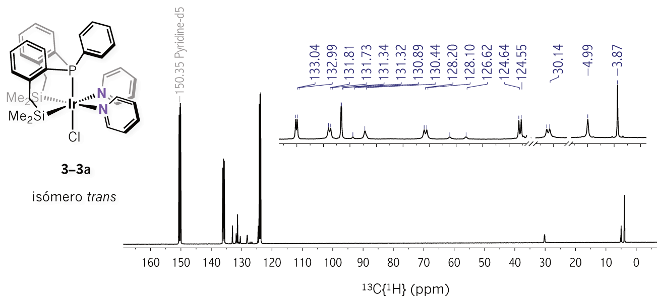
Figura 3A.13 RMN de ^{13}\text{C}\{^1\text{H}\} (100.6 MHz, 298 K, piridina- \text{d}_5 ) correspondiente a la reacción de 3-1a en disolución de piridina- \text{d}_5 a 298 K. Detección espectroscópica de 3-3a .
