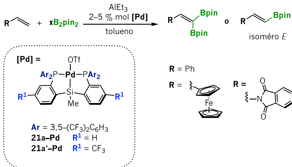
Esquema 1.28 Síntesis selectiva de ( E )-monoborilalquenos y/o 1,1-diborilalquenos a través de la borilación deshidrogenante de alquenos y diboranos catalizada por los complejos 21a-Pd y 21a'-Pd . 80
