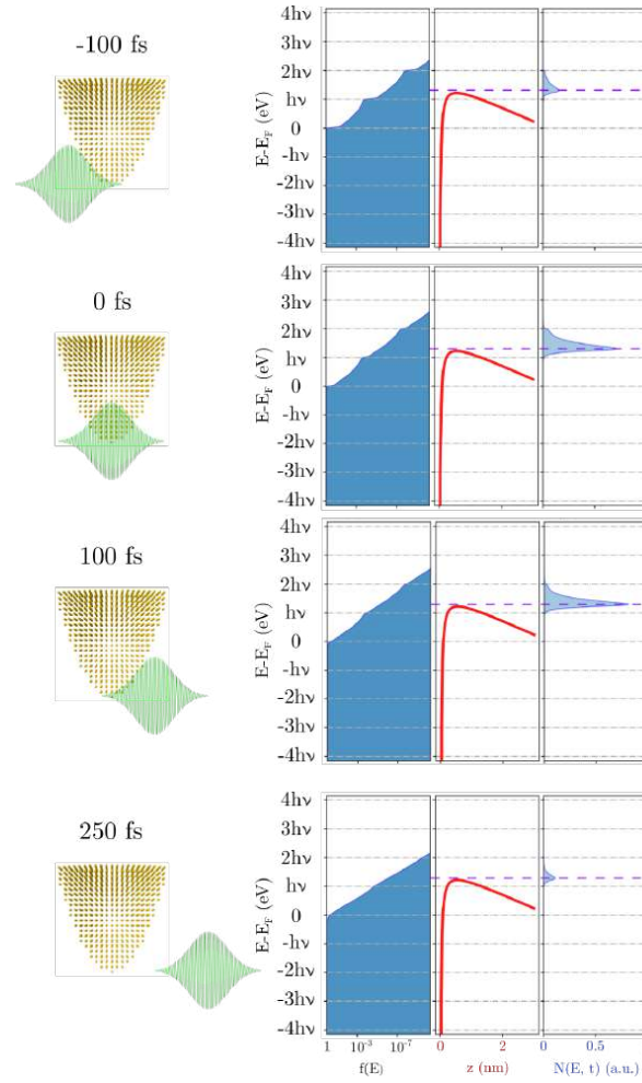
Figure V: Excitation optique ultra-rapide d'un gaz d'électrons. Le nanoémetteur de tungstène est esquissé avec une forme parabolique. Les trois graphiques représentent (de gauche à droite) : le numéro d'occupation des électrons f(E;t) (courbe bleu foncé), la barrière de potentiel (courbe rouge) et le nombre d'électrons émis N(E;t) (courbe bleu clair). Nous avons considéré une impulsion laser de \lambda = 515 nm et une durée d'impulsion FWHM de 250 fs. Le temps de thermalisation électron-phonon est de 400 fs. Le champ électrique CC appliqué est F_{loc} = 1,19 V/nm.
