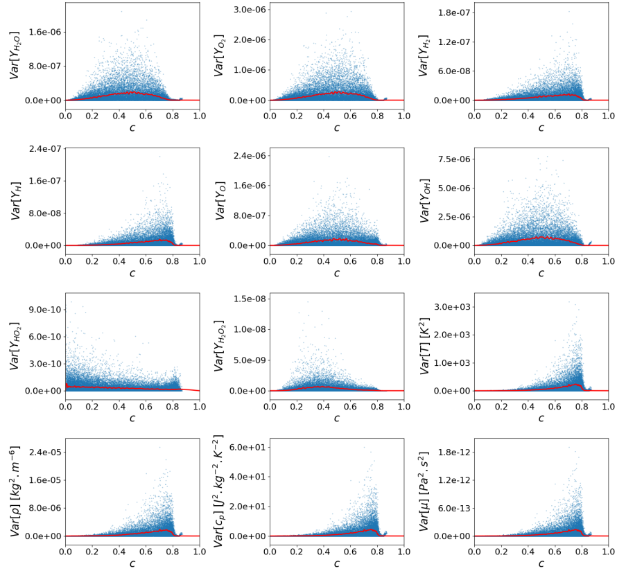
FIGURE 6.18 – Nuages de points de réalisations des couple de variables aléatoires (C_t, (X_t - E[X_t|C_t])^2) et fonctions \eta_X^{(t)} (lignes pleines rouges) calculés à l'aide d'une chimie détaillée pour un réacteur homogène adiabatique à pression constante et atmosphérique d'un mélange stœchiométrique air-hydrogène initialement à T = 1200 K, et pour l'instant t = 40\mu s .
