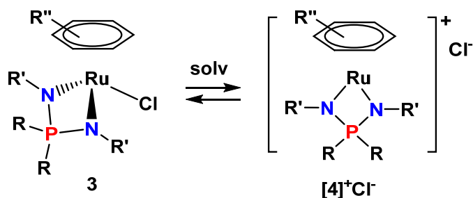
Schéma 5. Dissociation du chlorure dans les complexes 3 .
