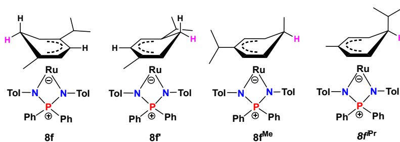
Scheme 10. Isomères possibles du complexe cyclohexadiényle 8f .
