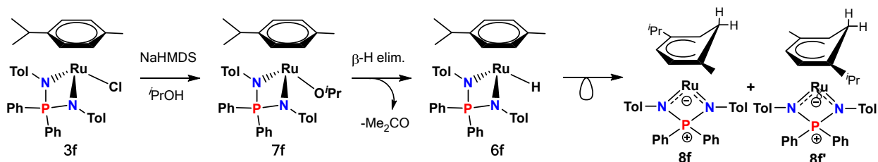
Scheme 9. Réarrangement du complexe hydrure 6f en complexes cyclohexadiényles 8f et 8f' pendant les tentatives d'isolation de 6f .
