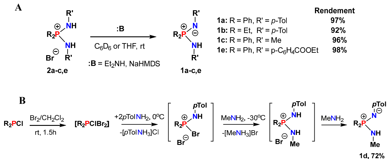
Schéma 2. (A) Synthèse des aminoiminophosphoranes 1a-c,e et (B) aminoiminophosphorane 1d .
