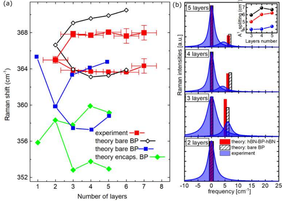
Figure B.11: (a) Énergies des branches intérieures et surface de la vibration A_g^1 en fonction du nombre de couches : de nos données (rouge) et des prévisions théoriques [Hu 2016] (noir) et [Birowska 2019] (bleu - BP nu et vert - BP encapsulé avec h-BN). (b) Intensité relative et division du mode A_g^1 en fonction du nombre de couches sur la base de nos données expérimentales (pics Lorentziens, les intensités sont normalisées à la composante principale A_g^1 , les largeurs correspondent au moyen FWHM du pic Raman, la fréquence de la composante principale est fixée à 0) et les calculs pour BP nu (barres noires) et encapsulé (barres rouges). L'encadré montre la différence d'énergie entre les pics intérieurs et de surface en fonction du nombre de couches. D'après [Birowska 2019].
