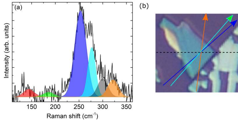
Figure B.25: (a) Exemple d'ajustement d'un spectre pour un angle d'excitation de 0^\circ avec des pics lorentziens; (b) Micrographie optique du flocon. La direction 0^\circ est marquée avec la ligne pointillée et les directions d'intensité maximale dérivées des diagrammes polaires pour les modes 186\text{ cm}^{-1} (vert), 253\text{ cm}^{-1} (bleu foncé) et 322\text{ cm}^{-1} (orange) sont indiquées par les flèches.
