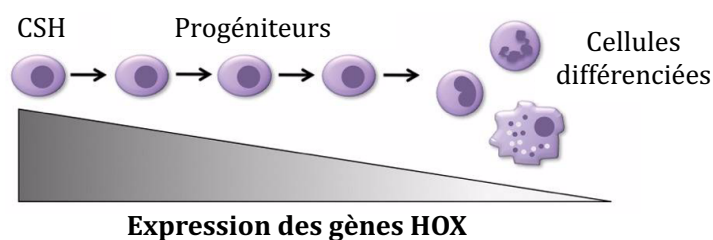
Figure 17 : Expression des gènes HOX au cours de l'hématopoïèse normale. Tiré de Collins and Hess, 2016a.
