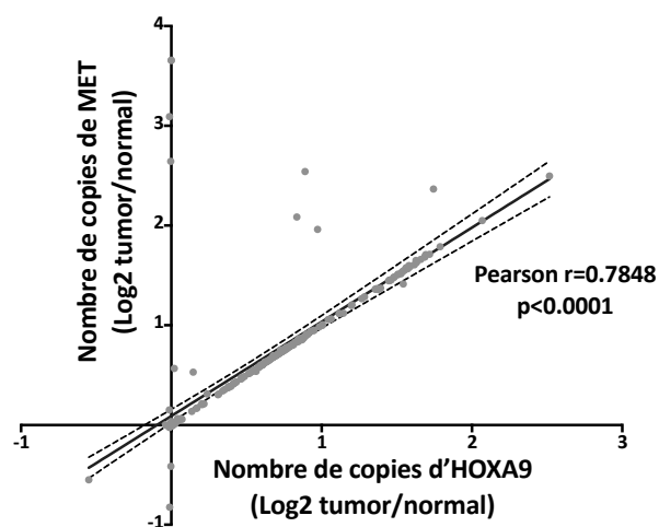
Figure 35 : Corrélation entre le nombre de copies d' HOXA9 et de MET . La droite représente la droite de régression linéaire avec intervalle de confiance à 95% (traits pointillés). Le coefficient de corrélation est calculé par test de Pearson.
