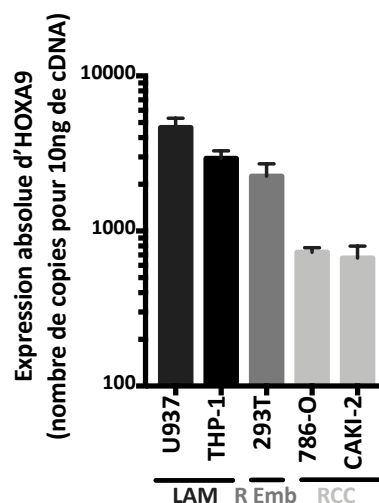
Figure 40 : Expression absolue d'HOXA9 dans différentes lignées de LAM, de rein embryonnaire et de RCC. L'expression a été déterminée par qPCR et est exprimée en nombre de copies d'ARNm pour 10ng d'ADN complémentaire. LAM : leucémie aiguë myéloïde, R Emb : rein embryonnaire, RCC : carcinome à cellules rénales. n=3 à 4, moyenne +/- sem.
