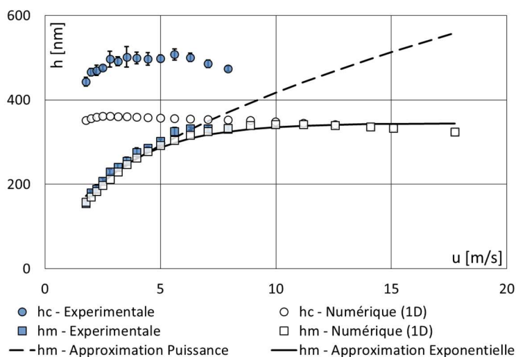
Figure i-13 – Variation de l'épaisseur centrale et minimale de film avec la vitesse, w^{1D} = 5,82 \times 10^4 \text{ N} \cdot \text{m}^{-1} et T_0 = 293,15 \text{ K} . Trois fois l'écart type est indiqué en noir pour les résultats expérimentaux.
