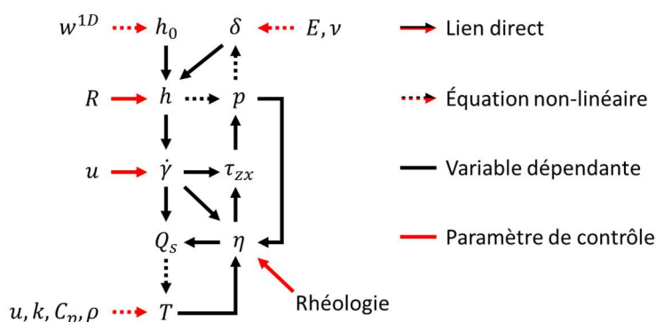
Figure i-12 – Différents liens entre les paramètres de contrôle et les variables dépendantes dans les contacts à vitesse d’entrainement nulle.
