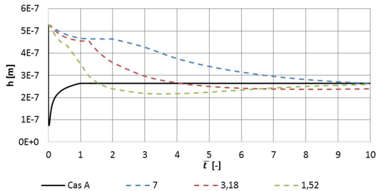
Figure i-24 – Variation de l'épaisseur minimale de film dans les cas A et C, pour \bar{t}_T = \{1,52; 3,18; 7\} , en fonction de \bar{t} .
