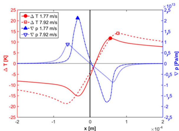
Figure i-14 – Différences de température (en rouge, axe de gauche) entre les deux interfaces et gradient de pression (en bleu, axe de droite) dans le fluide à w^{1D} = 5,82 \times 10^4 \text{ N} \cdot \text{m}^{-1} et T_0 = 293,15 \text{ K} , pour deux vitesses différentes.
