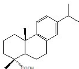
Figure 22: Acide déhydroabiétique.
