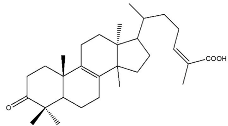
Figure 39: Acide isomasticadiénonique.
