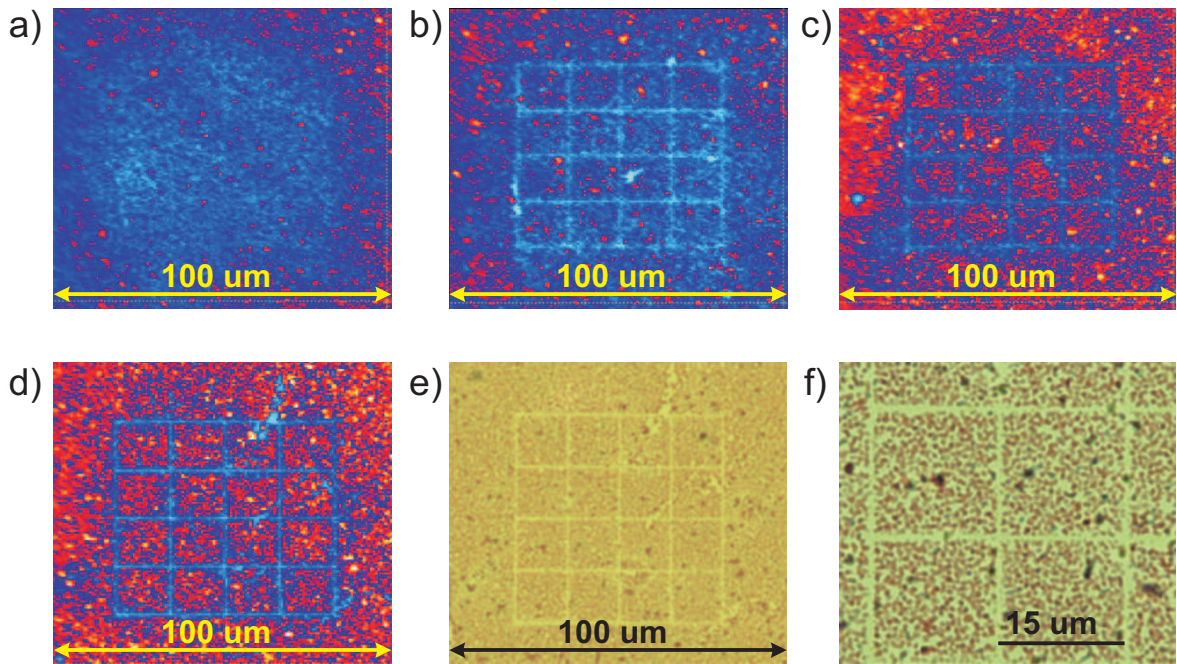
Figure 3.22: Images de fluorescence d'échantillons de DAST après photoblanchiment avec différentes combinaisons de paramètres d'écriture, qui peuvent être présentés comme un couple "puissance-vitesse": a) 1 mW-5 \mu\text{m} / s b) 5 mW-5 \mu\text{m} / s c) 5 mW-10 \mu\text{m} / s d) 10 mW-35 \mu\text{m} / s. e) - f) Image optiques de l'échantillon enregistrées avec une puissance de 10 mW et une vitesse de 35 \mu\text{m} / s et prises par un microscope optique.
