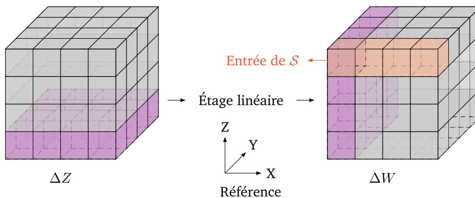
Figure 3.8.: Diffusion d'une faute obtenue lors de l'exécution d'une structure CUBE.
