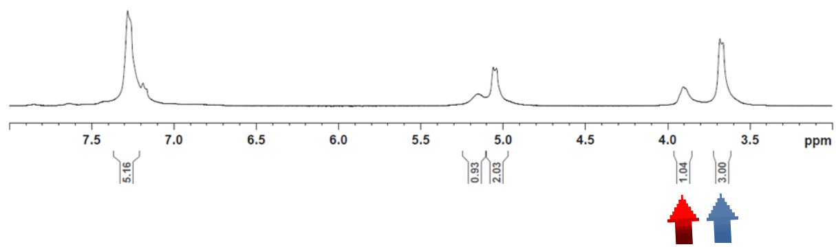
1 H-NMR Reference 18c
