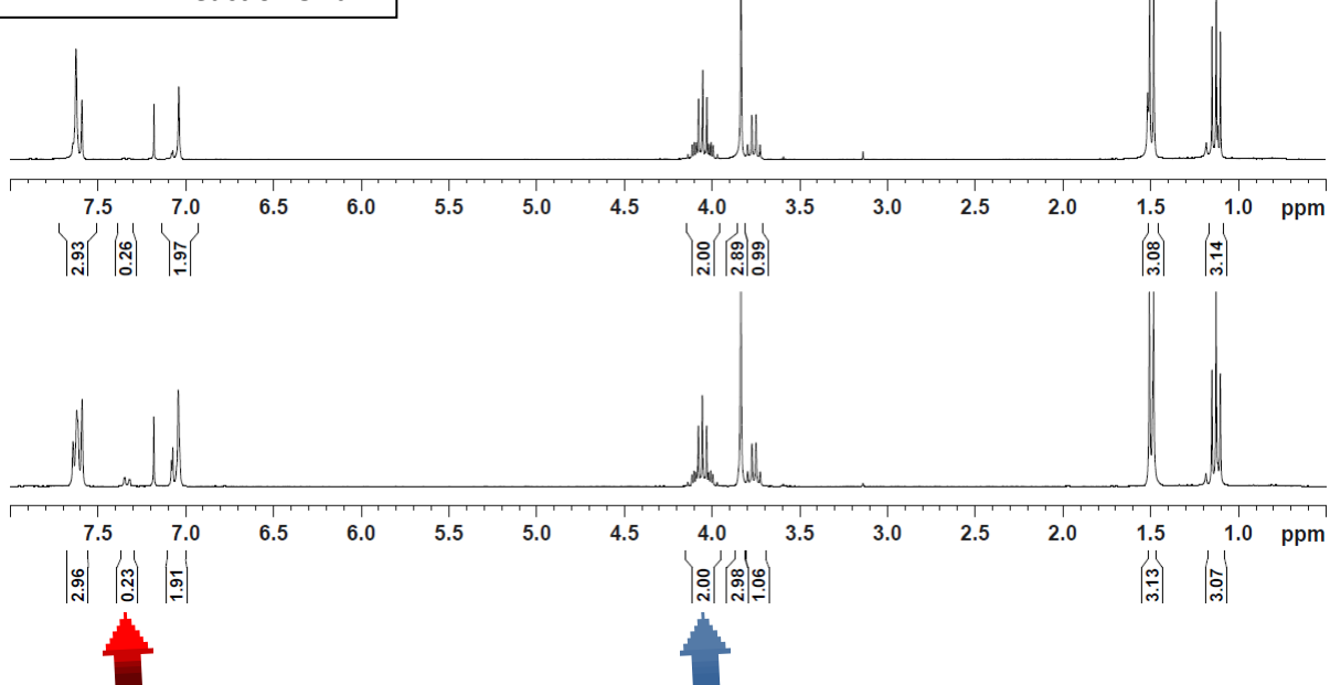
1 H-NMR HIE reaction 52b
