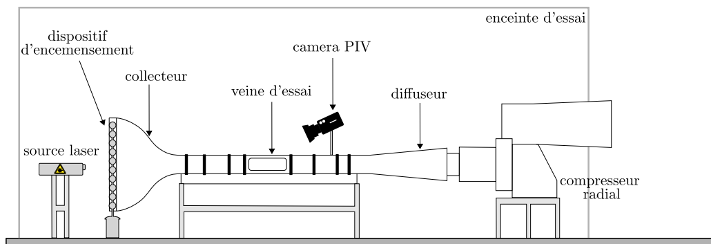
FIGURE 2.3 – Installation soufflerie de couche limite Vélocimétrie par Images de Particules de l'ONERA Lille
