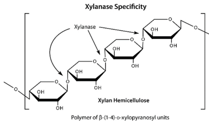
Figure 7 : Hémicellulose
