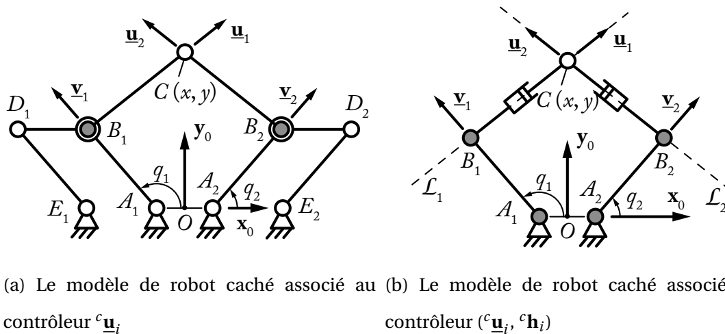
FIGURE 3.4 – Robots cachés associés au mécanisme à cinq barres.
