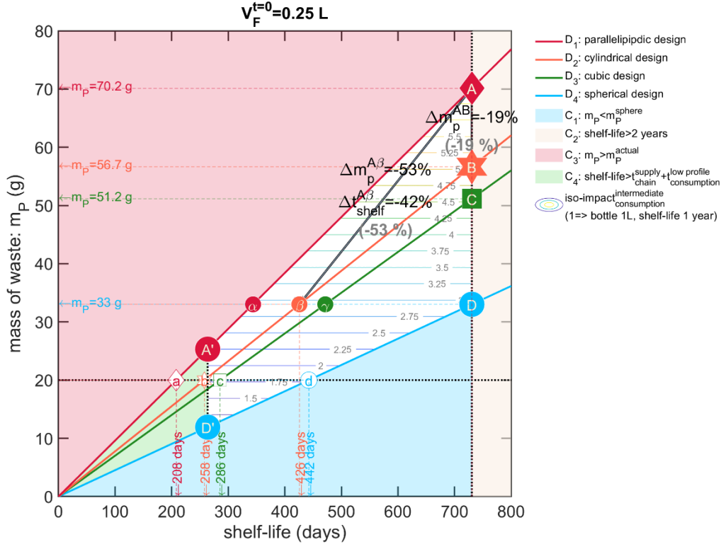
Figure VII-2. Représentation géométrique des équations (VII.1) et (VII.3)-(VII.4) pour une bouteille de 0.25 L. Les isocontours représentent les valeurs du rapport \frac{M_p(V_F^{t=0}=0.25 L)}{M_p(V_F^{t=0}=1 L)} .
