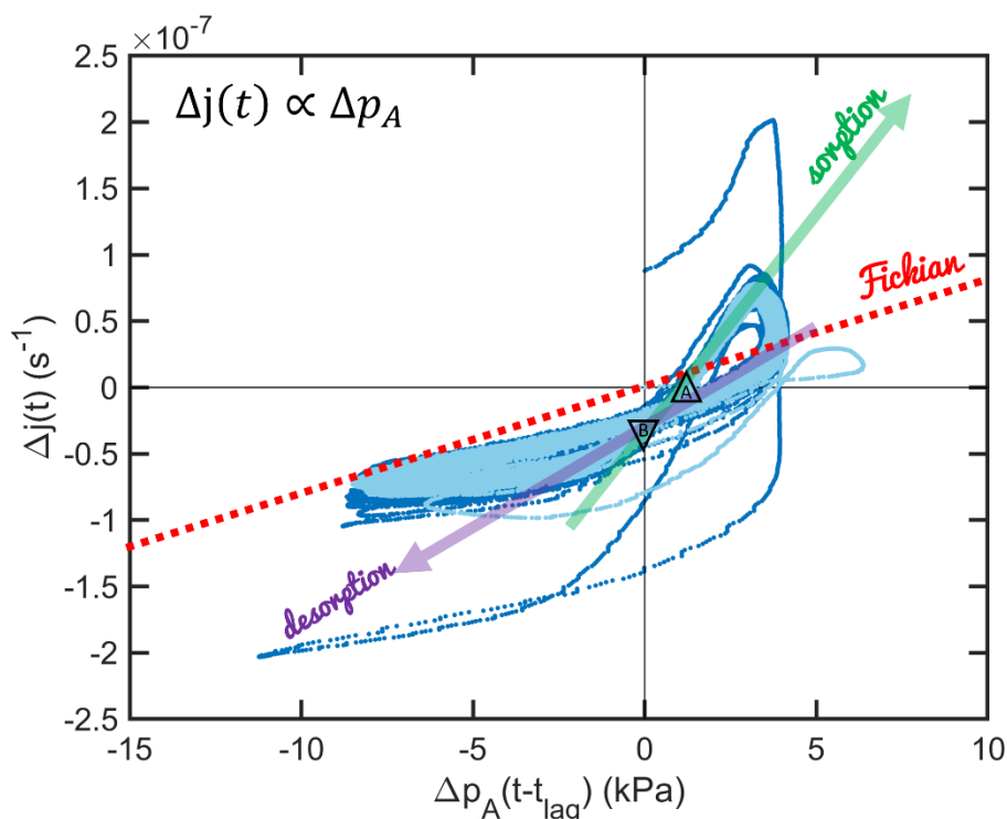
Figure VII-9. Analyse des fluctuations du flux de matière en fonction de la fluctuation périodique (période de 240 s) de la pression partielle en vapeur d'eau à 50°C pour un échantillon de 630 μm d'épaisseur.
