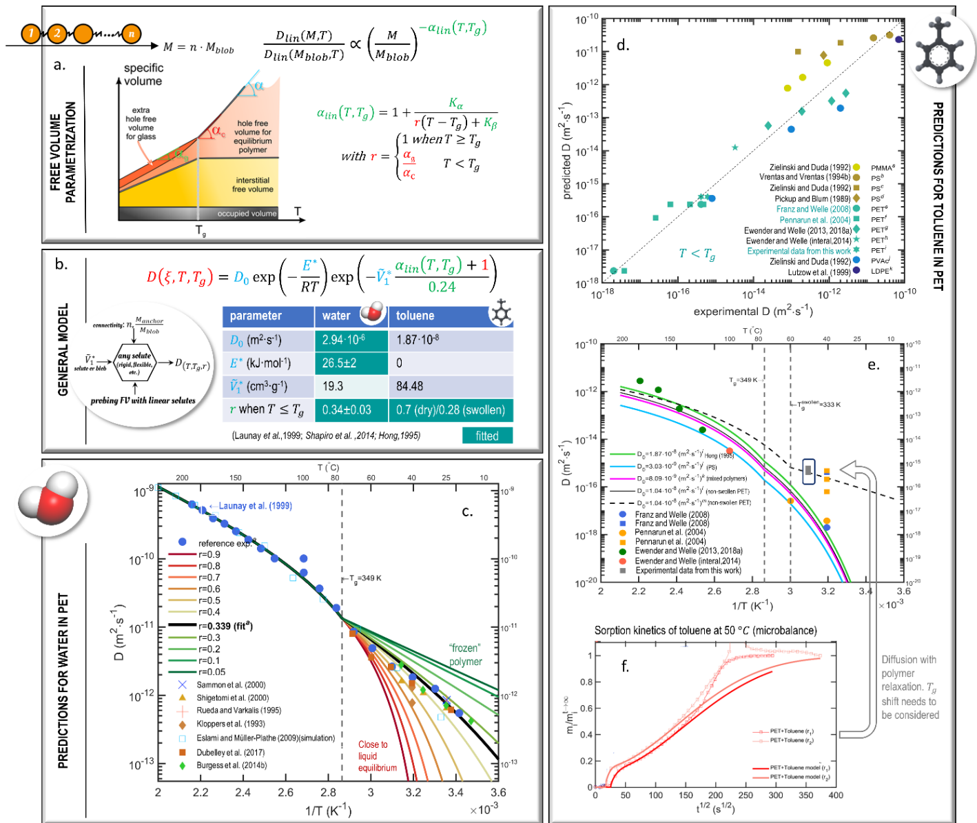
Figure VII-8. Paramétrisation et prédictions des coefficients de diffusion de l'eau et de l'éthanol dans le PET à l'état caoutchoutique et vitreux : (a) lois d'échelle à l'état caoutchoutique et vitreux pour des molécules sondes linéaires ; (b) modèle générique de coefficients de diffusion et paramétrage du modèle pour l'eau et le toluène ; (c) validation pour l'eau sur la base d'une identification de r à partir des données de Launay et al. (1999) ; (d) validation pour le toluène dans cinq polymères ; (e) dépendance des coefficients de diffusion du toluène à la température ; (f) cinétiques de sorption à 50°C mettant en évidence la relaxation du polymère.
