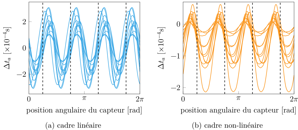
Figure 6.6 Évolution de \Delta t_a sur le dernier tour pour le modèle désaccordé, en fonction de la position angulaire du capteur, avec les positions des extremums d'excitation indiquées (---).
