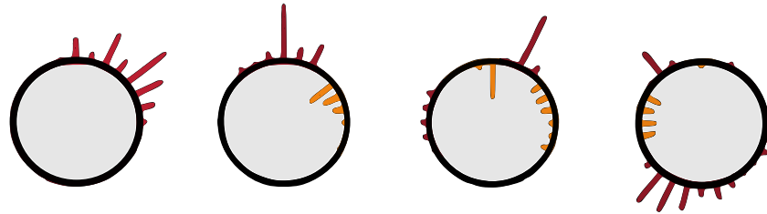
Figure 2.7 Représentation schématisée des modes d'une roue aubagée désaccordée : l'énergie est localisée, seules certaines aubes sont déformées suivant de grandes amplitudes. Adapté de [5].
