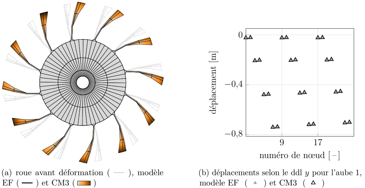
Figure 4.7 Comparaison du mode propre à plus basse fréquence entre le modèle désaccordé EF, calculé avec Samcef, et le modèle désaccordé construit par la CM3.
