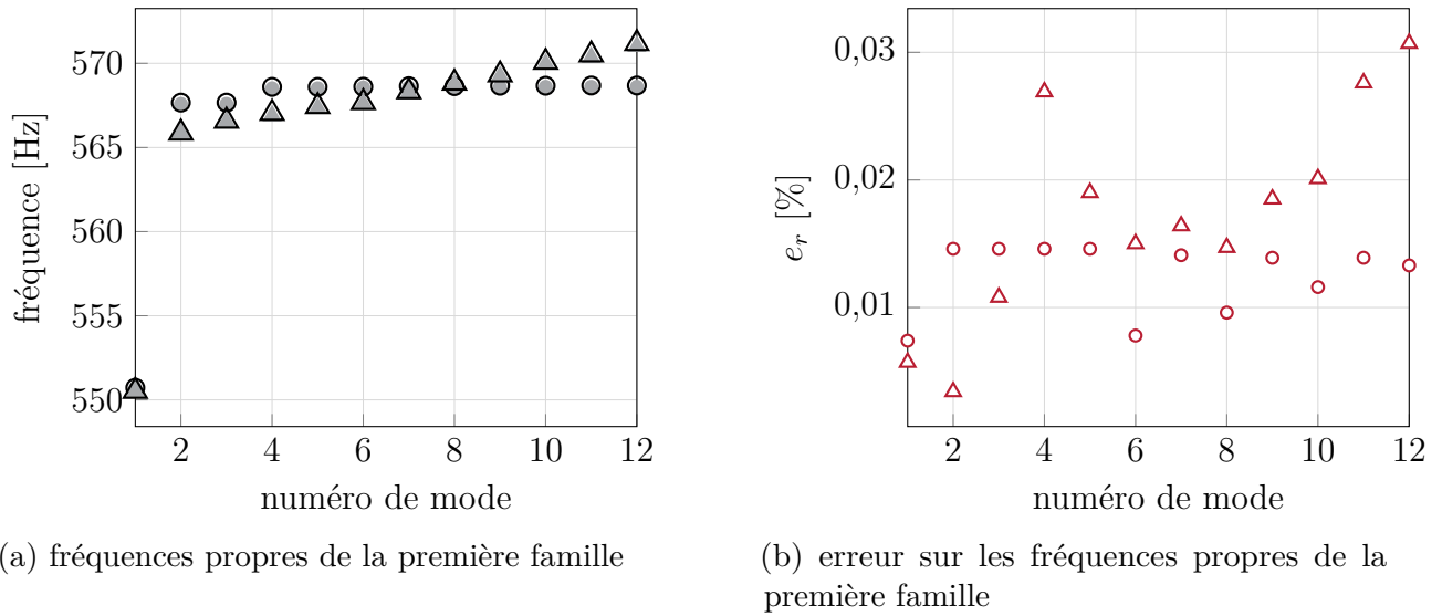
Figure 4.6 Fréquences propres, Samcef/CM3/erreurs associées, sur la première famille modale pour les modèles accordés ( \circ ) / ( \bullet ) / ( \circ ) et désaccordés ( \Delta ) / ( \blacktriangle ) / ( \triangle ).
