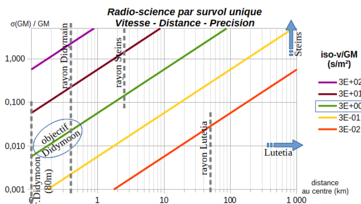
FIGURE 2.7 – Précisions atteintes par radio-science lors d'un survol unique ( \sigma_v = 0.02 mm/s, quelques iso- (v/GM) donnés en table 2.4).
