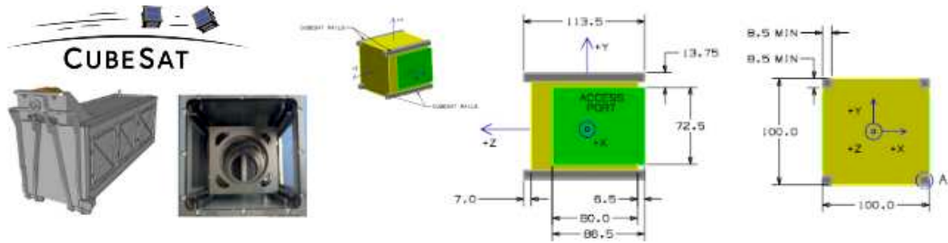
FIGURE 2.1 – Extractions du CubeSat Design Specification, Rev.13 : à gauche le déployeur (design extérieur et photo de l'intérieur), à droite les dimensions pour 1U
