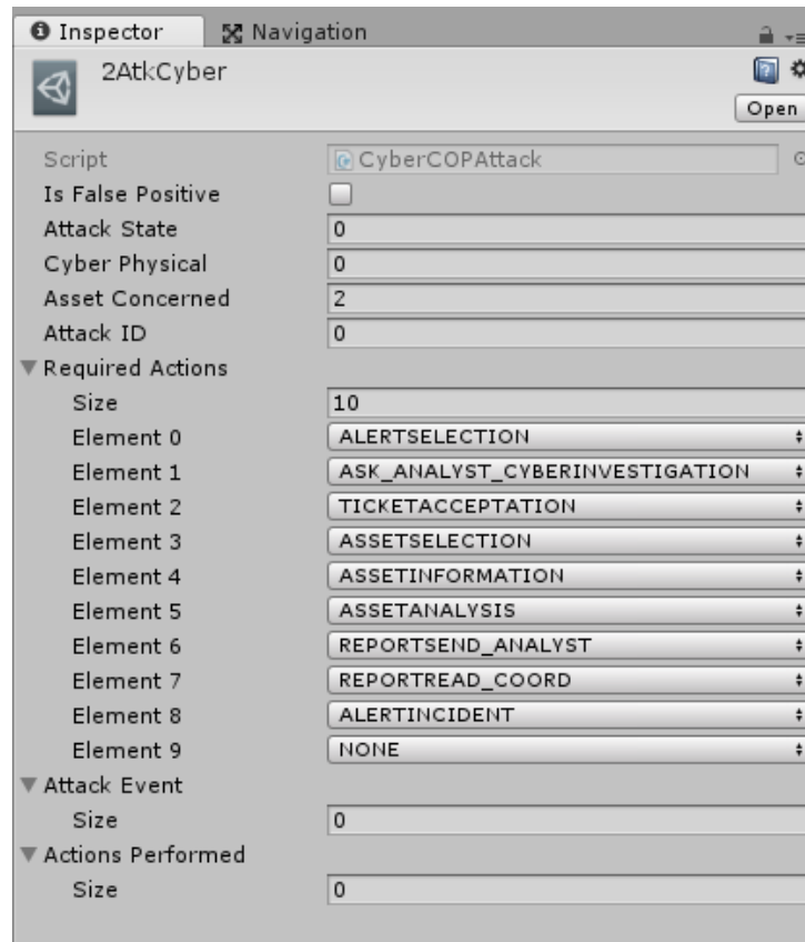
FIGURE 4.11 – Vue éditeur du Scriptable Object de l'attaque 2AtkCyber. C'est dans cette vue que le créateur du scénario peut modifier les propriétés d'une attaque sur un asset, en paramétrant le numéro de l'asset concerné, la vue concernée (IT ou Cyber), la nature de l'attaque (véritable attaque ou faux positif) et la procédure des actions à effectuer pour réussir l'analyse de l'alerte liée à cette attaque.
