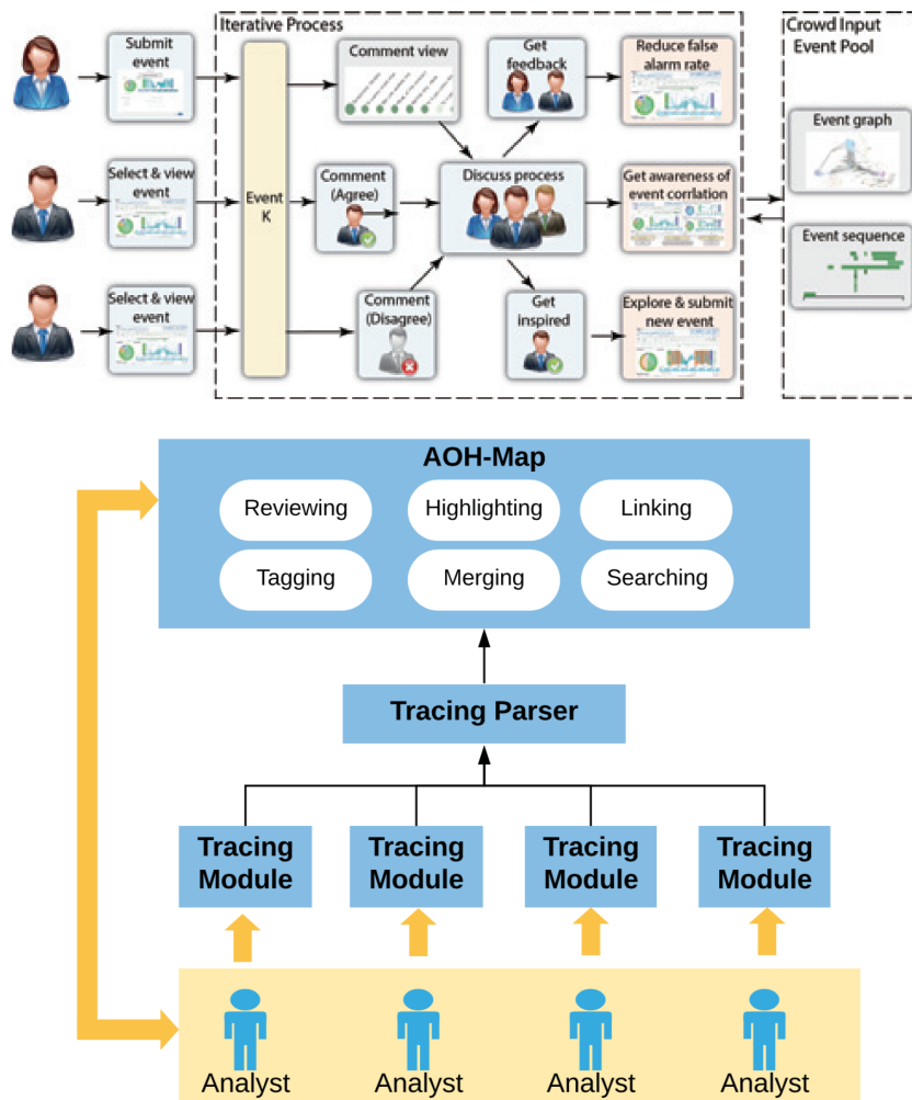
FIGURE 1.20 – Architecture collaborative des outils d'analyse d'événements OCEANS (extrait de [19], en haut) et AOH-Map (extrait de [133], en bas) (© 2019, IEEE). Ces outils permettent à plusieurs utilisateurs d'échanger des informations et de visualiser leurs traces d'interaction et leurs raisonnements. L'échange d'information est un vecteur de risque de fuite de données.
