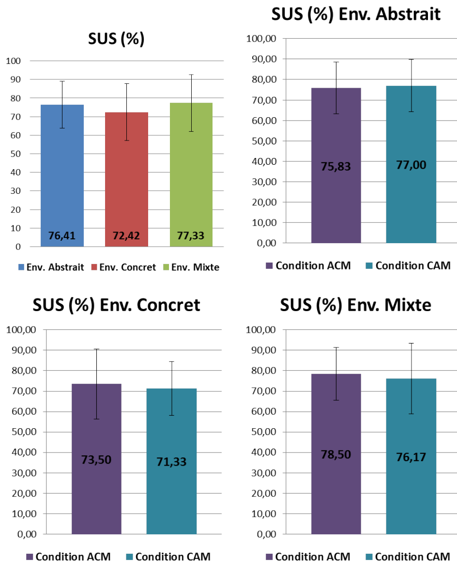
FIGURE 5.15 – Scores SUS pour les différents types d'environnements en moyenne et en fonction des conditions. Les scores sont supérieurs à 70/100 et il n'y a pas d'effets liés à la condition.
