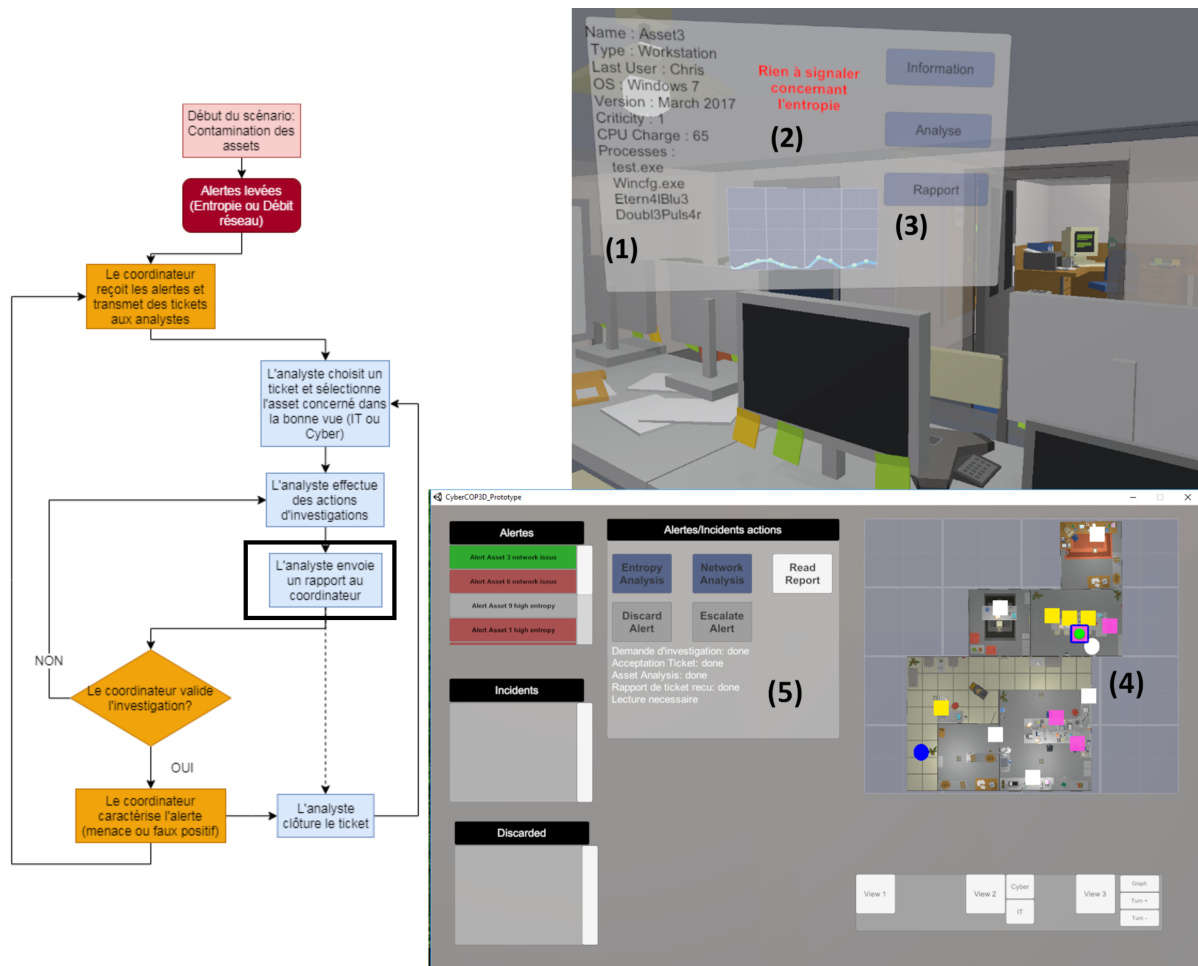
FIGURE 5.7 – (1) Récupération des informations, du (2) résultat d'analyse et (3) envoi du rapport par l'analyste. Réception du rapport par le coordinateur : (4) mise à jour de la minicarte (l'asset concerné change de couleur) et (5) des actions utilisateur (action de lecture de rapport activée).
