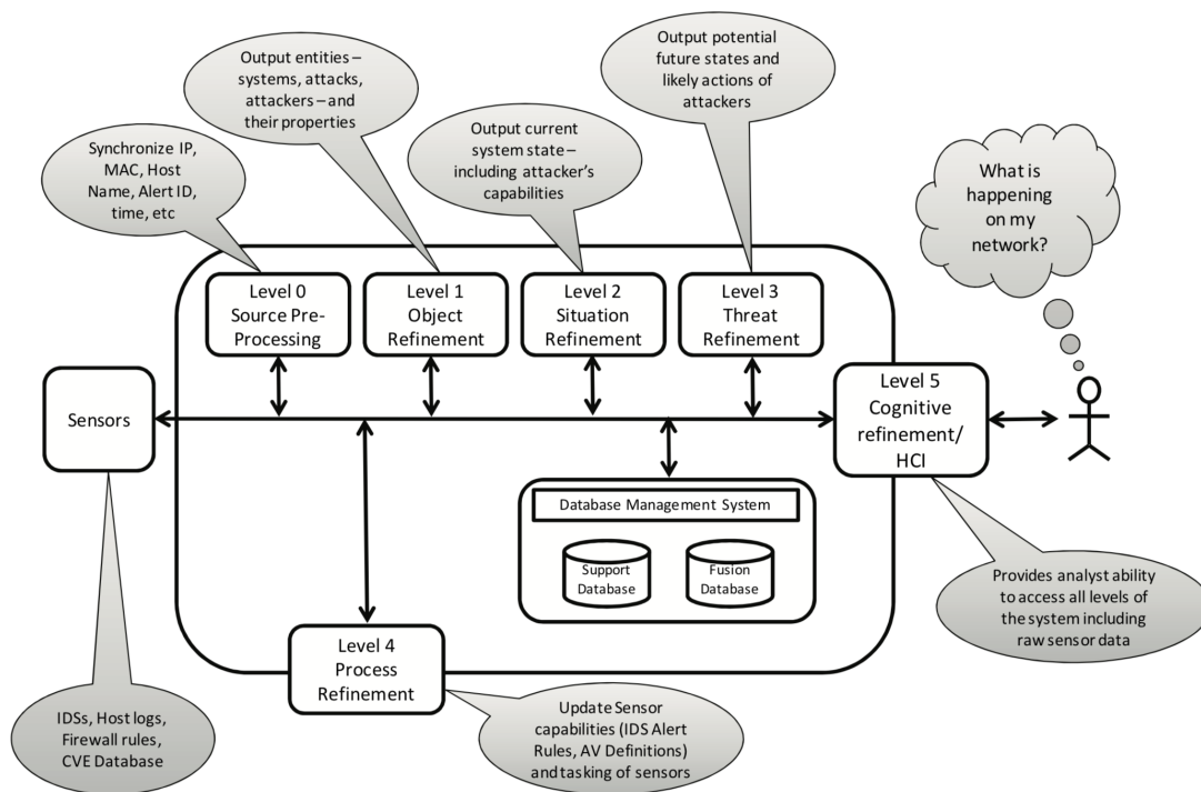
FIGURE 1.6 – Modèle Joint Director of Laboratories (JDL) adapté à la cybersécurité, proposé par Giacobe [49] (© 2010, SPIE). Dans ce modèle, les données sont fusionnées dans une vue agrégée de la situation.
