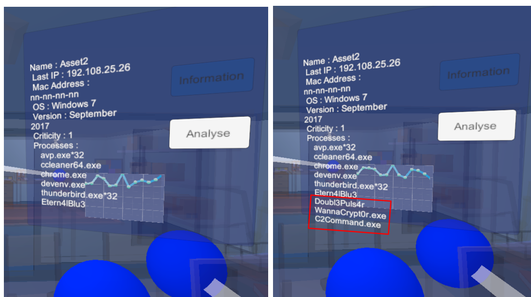
FIGURE 5.21 – Liste incomplète des processus tournant sur un asset (à gauche) et liste complète (à droite).
