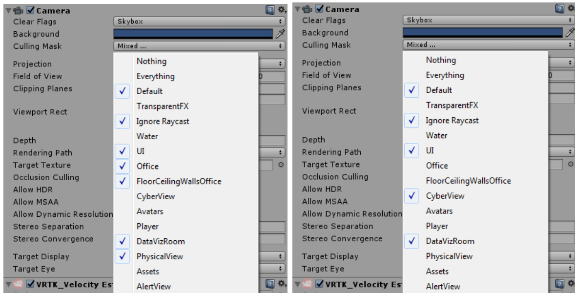
FIGURE 4.19 – Couches d’affichage des caméras en vue IT et Cyber. On peut remarquer que les couches de rendu Office et CyberView vues dans la Figure 4.18 sont activées ou désactivées en fonction de la vue.
