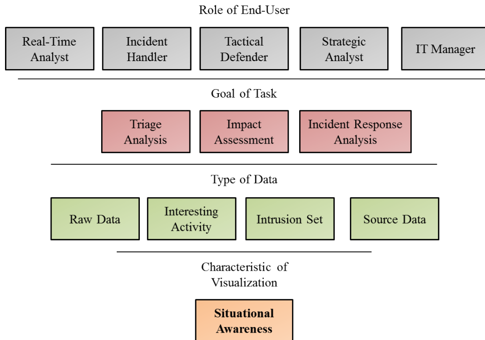
FIGURE 1.15 – Représentation dans le framework EEVi des liens entre visualisation de données pour la CSA, rôles et tâches des analystes et les sources de données requises, adapté de [108]. On peut remarquer que la CSA concerne beaucoup de rôles différents d'utilisateurs ainsi que des sources de données hétérogènes.
