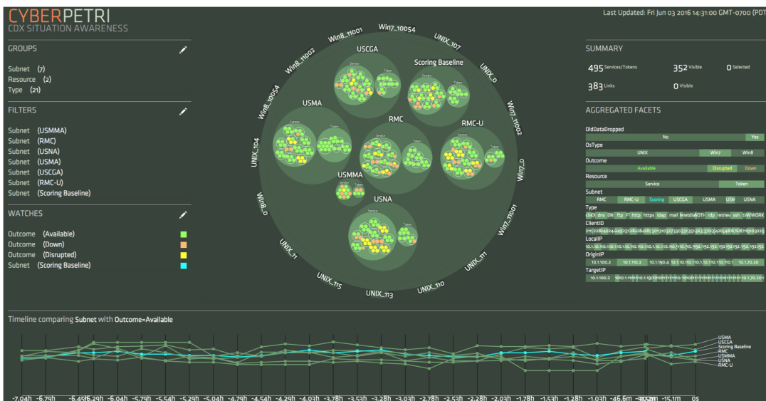
FIGURE 1.19 – En haut, EntVis, Outil de Visual Analytics pour les détections d'anomalies du trafic réseau, extrait de [136] (© 2015, IEEE). En bas, Outil CyberPetri, pour l'étude de l'évolution de l'état d'un challenge de cybersécurité, extrait de [2] (© 2016, IEEE).
