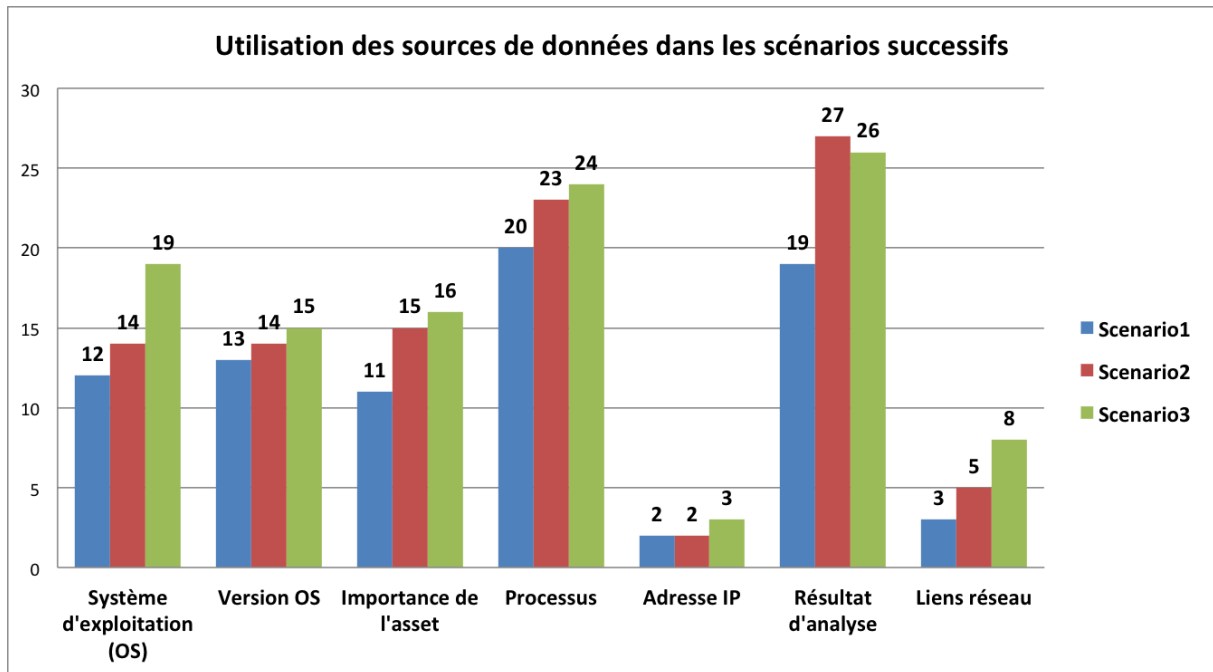
FIGURE 5.19 – Utilisation des données par les utilisateurs au fur et à mesure des expérimentations. Les utilisateurs ont de plus en plus utilisé les données à leur disposition (progression du nombre d'utilisations entre les scénarios 1 et 3) et ont utilisé en majorité les résultats d'analyse et la liste des processus pour caractériser les alertes.
