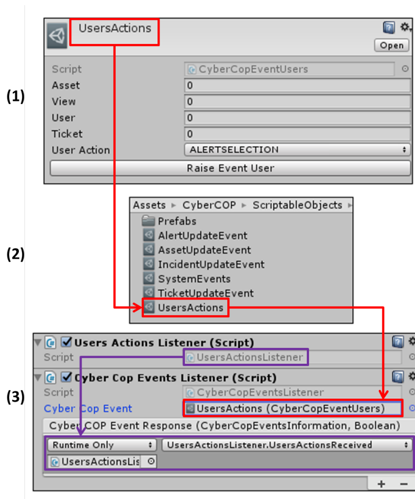
FIGURE 4.2 – Scriptable Object UsersActions d'événements. (1) Modification des attributs via un éditeur fourni par Unity. (2) UsersActions s'instancie directement via un menu de l'explorateur de fichiers. (3) Il s'utilise en le glissant-déposant dans un script d'objet de Unity et en y faisant référence dans le script.
