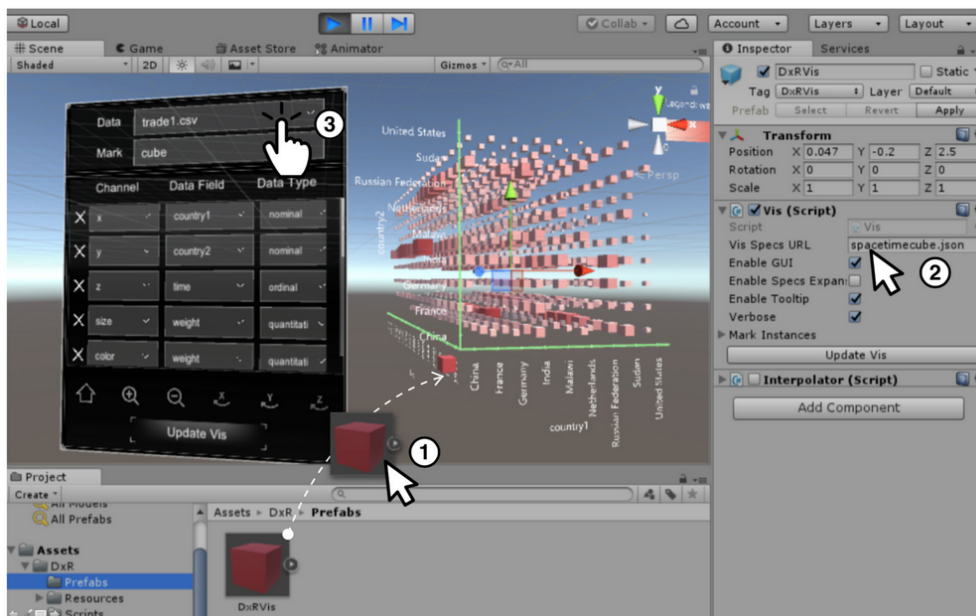
FIGURE 2.11 – Outil DXR de développement de visualisations de données immersives, extrait de [112] (© 2019, IEEE).
