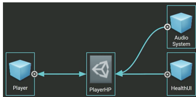
FIGURE 4.1 – Exemple de découplage entre émission et réception d'événements proposé par l'utilisation des Scriptable Objects, extrait de https://blogs.unity3d.com/2017/11/20/making-cool-stuff-with-scriptableobjects/ .
