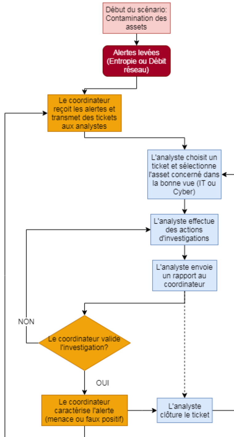
FIGURE 3.14 – Scénario collaboratif d’analyse de WannaCry proposé pour une instantiation du modèle CyberCOP 3D dans un EVC. Le coordinateur reçoit les alertes et transmet des tickets aux analystes. Ces derniers sélectionnent l’asset concerné dans la vue requise par l’analyse (Cyber ou IT), puis effectuent des actions d’investigation. Enfin, ils transmettent un rapport au coordinateur qui caractérise l’alerte, ce qui permet aux analystes de clôturer le ticket.
