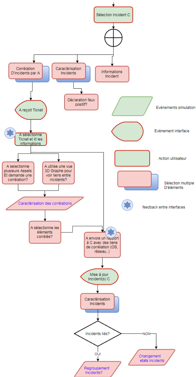
FIGURE 5.10 – Déroulement de la phase de corrélation d’alertes de notre scénario. L’objectif est de croiser les informations entre les alertes afin de déterminer si elles proviennent d’une même cause.
