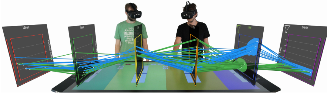
FIGURE 2.13 – Exemple d’un environnement de Collaborative Immersif Analytics permettant l’analyse collaborative de données multidimensionnelles, extrait de [15] (© 2018, ACM). Les utilisateurs munis de casques de Réalité Virtuelle interagissent sur des données via des gestes et via l’utilisation d’une table tactile.
