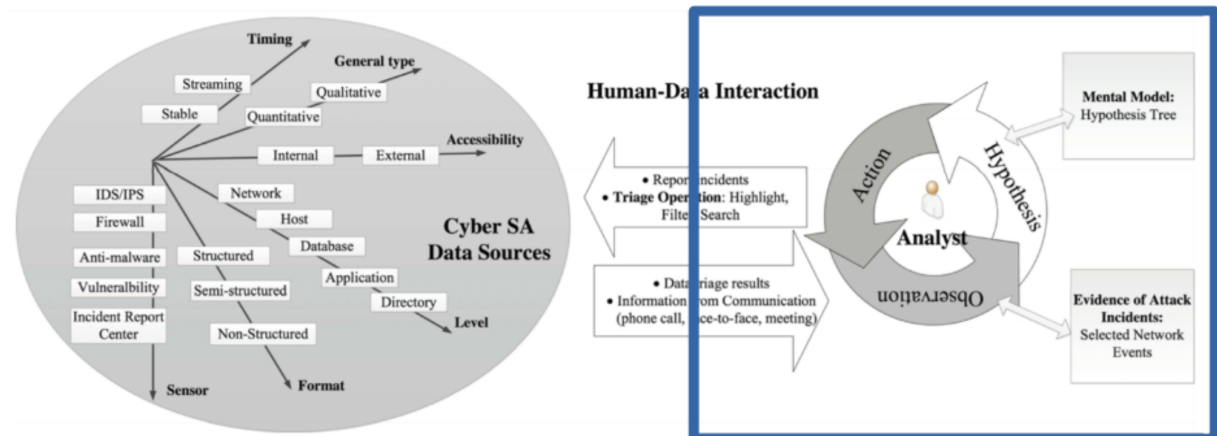
FIGURE 1.7 – Traitement humano-centré (partie encadrée, à droite) des données en cybersécurité, extrait de [134] (© 2017, Springer). Les modèles cognitifs de la CSA concernent la prise d'informations par un opérateur humain.
