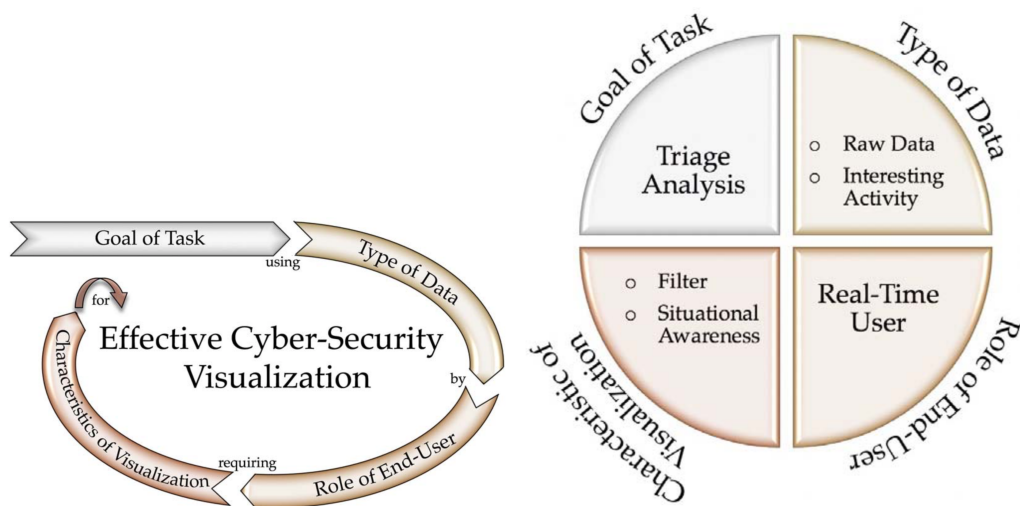
FIGURE 1.14 – Framework EEVi pour le développement de visualisations adaptées aux utilisateurs, extrait de [108] (© 2017, IEEE). L'image de gauche décrit le processus de développement d'un outil de visualisation tandis que l'image de droite présente un exemple de relations entre une tâche de triage de données, les données à utiliser, les rôles dédiés à cette tâche ainsi que les caractéristiques de l'outil.
