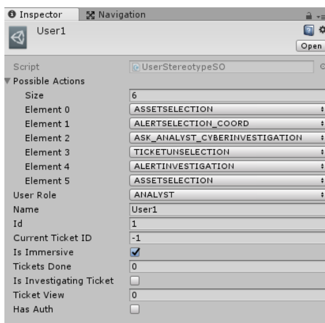
FIGURE 4.12 – Vue éditeur du Scriptable Object User1 contenant les informations d'un utilisateur. Ces informations sont modifiables directement dans l'éditeur de Unity et seront ensuite utilisées dans le Scriptable Object de scénario présenté précédemment.
