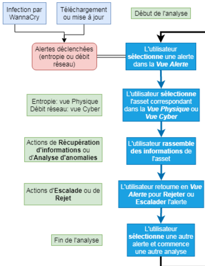
FIGURE 5.13 – Scénario simplifié pour notre étude de l'utilisabilité d'un environnement virtuel pour l'analyse d'alertes. Dans ce scénario, l'analyste agit seul pour étudier les alertes et les caractériser.
