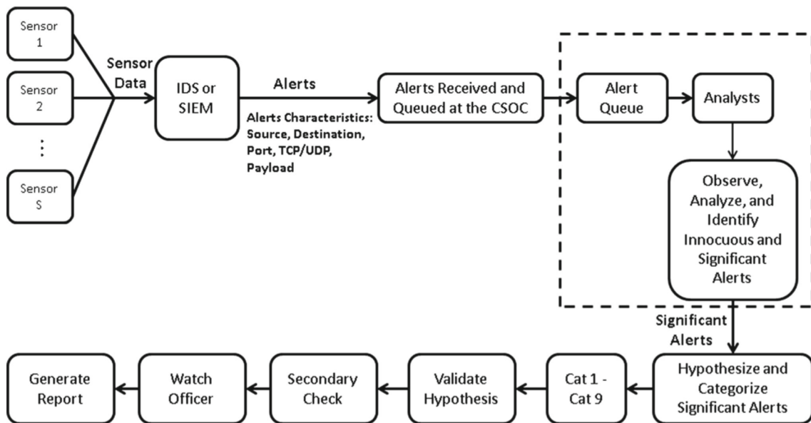
FIGURE 3.6 – Procédure d’analyse de traitement d’alertes, extrait de [110] (© 2018, Springer). Ces dernières sont centralisées par le SIEM et transmises aux analystes qui les traitent individuellement. Si une alerte est jugée pertinente, elle est alors vérifiée une seconde fois et à l’issue de la vérification un rapport est produit.
