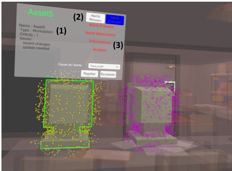
FIGURE 5.11 – Vue alerte qui remplace le système de ticketing . Cette vue contient (1) des informations sur l'asset et sur (2) les alertes le concernant. Le texte rouge (3) correspond à l'historique d'actions déjà effectuées sur l'alerte sélectionnée, en l'occurrence l'alerte entropie.
