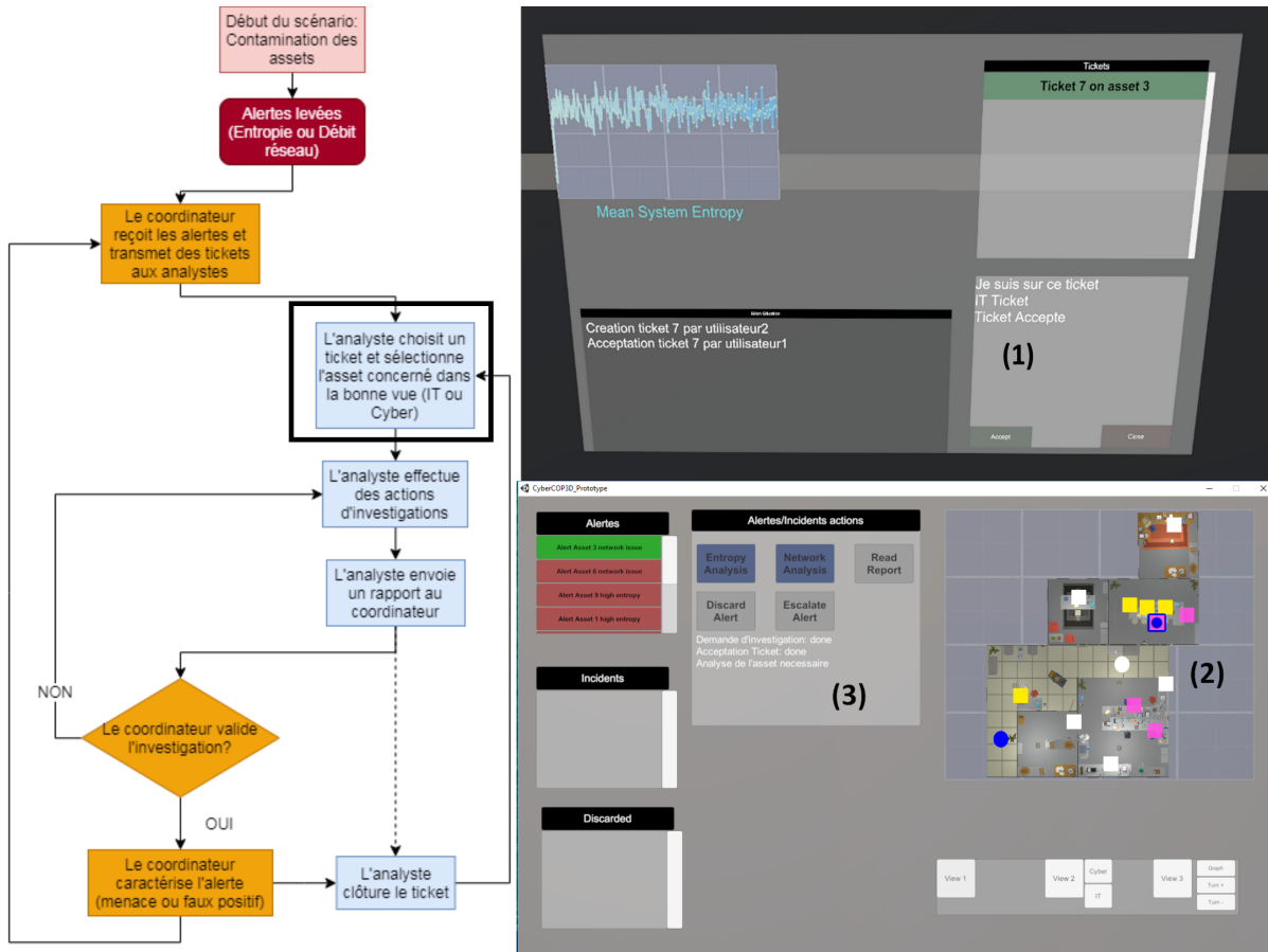
FIGURE 5.3 – (1) Acceptation du ticket par l'analyste et mise à jour de l'interface du coordinateur ((2) changement de couleur de l'asset concerné et (3) mise à jour des informations sur l'alerte).
