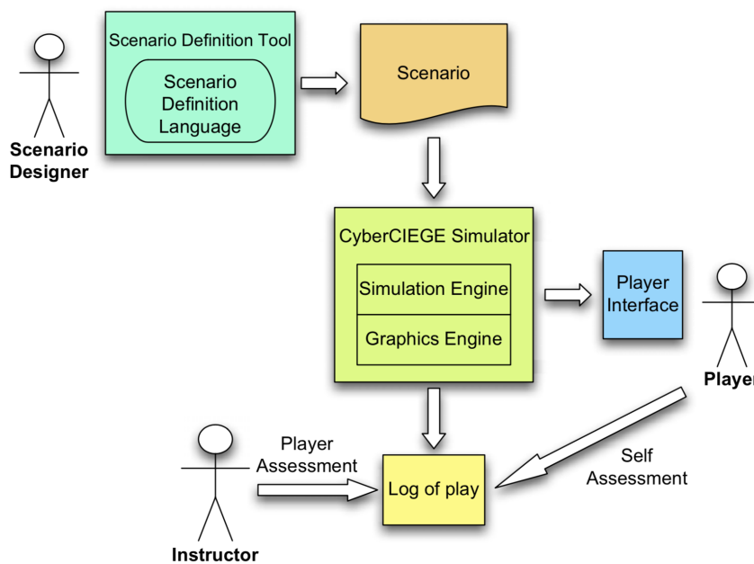
FIGURE 1.30 – Architecture du serious game CyberCIEGE [23] (© 2007, Elsevier), composée d'un moteur de scénarios qui permet de définir et d'implémenter des scénarios dans le simulateur, du simulateur à proprement parler qui gère la progression de l'utilisateur dans le scénario et qui lui propose une interface immersive adaptée, ainsi que d'un outil de visualisation des traces utilisateurs permettant à un instructeur d'évaluer la pratique de l'utilisateur.
