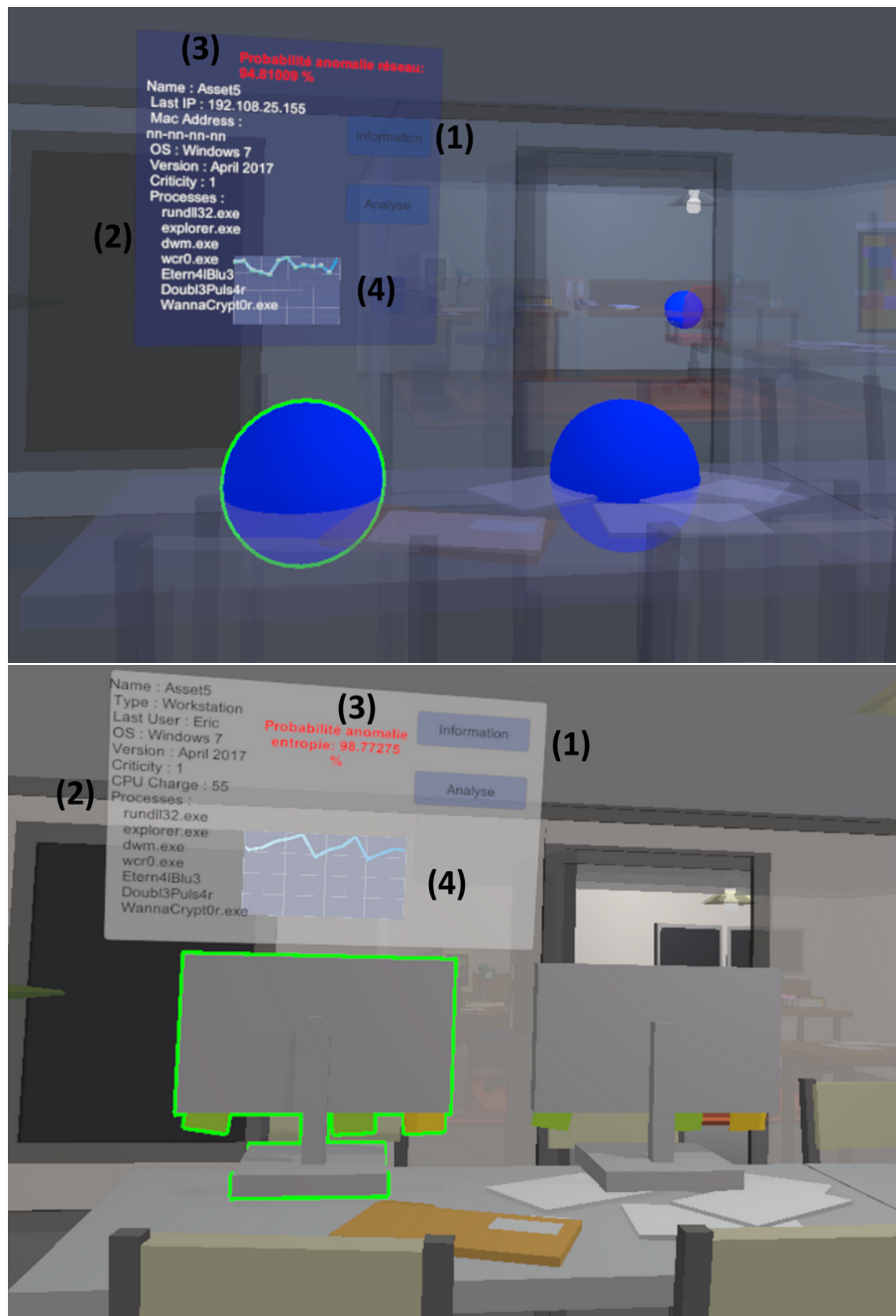
FIGURE 5.12 – Vue Cyber (en haut) et vue IT (en bas). Ces vues contiennent (1) les actions d'analyse, (2) des informations relatives à l'asset, (3) le résultat de l'analyse d'anomalies et (4) une visualisation des métriques d'entropie et de débit réseau, en fonction des vues.
