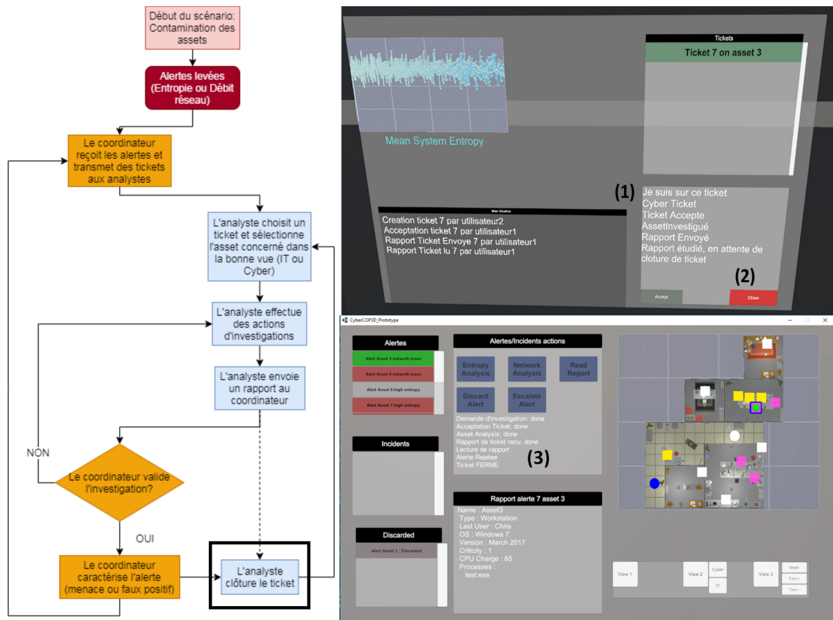
FIGURE 5.9 – (1) Mise à jour des informations du ticket sur le tableau de bord. L'analyste peut alors (2) fermer le ticket, ce qui (3) met à jour l'affichage du coordinateur.
