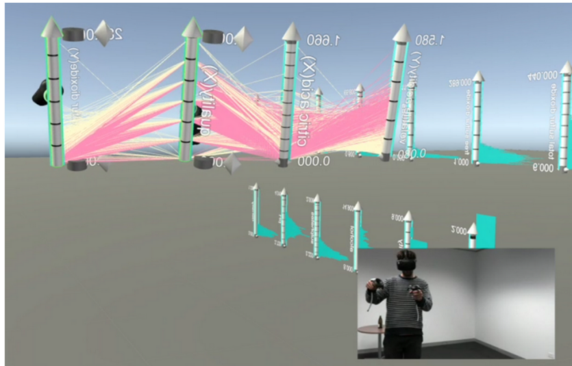
FIGURE 2.12 – ImAxes, extrait de [25] (© 2017, ACM). Cette métaphore d'interaction permet de croiser des graphes 2D afin de voir directement les corrélations entre les données.
