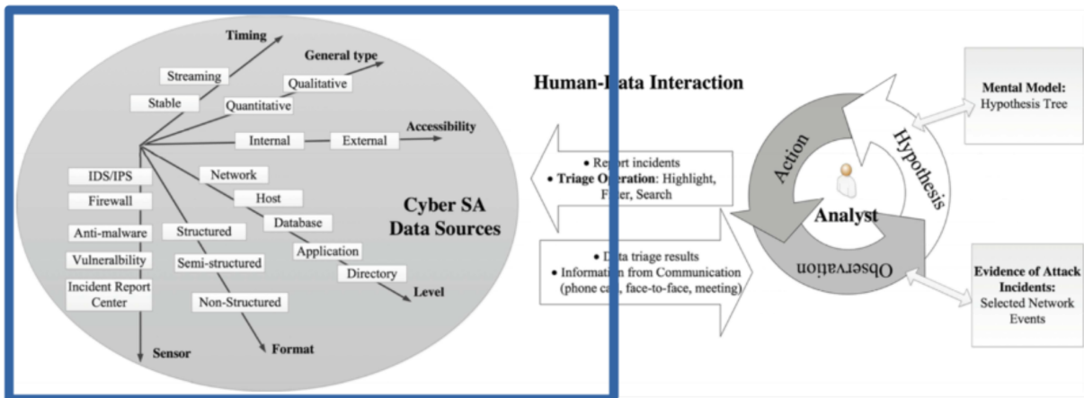
FIGURE 1.4 – Traitement techno-centré (partie encadrée, à gauche) des données en cybersécurité, extrait de [134] (© 2017, Springer). Les modèles de fusion et de corrélation de données pour la CSA ne concernent que l'aspect technique du traitement de l'information.
