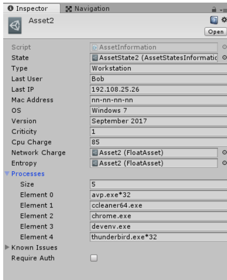
FIGURE 4.10 – Vue éditeur du Scriptable Object Asset2 contenant les informations d'un asset de la simulation. Ces informations sont modifiables directement dans l'éditeur de Unity et seront ensuite utilisées dans le Scriptable Object de scénario présenté précédemment.
