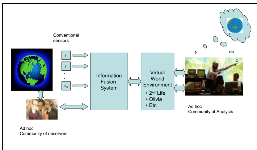
FIGURE 1.23 – Architecture de solution pour l'analyse collaborative immersive de données pour la cybersécurité, extrait de [56] (© 2008, IEEE). L'EV reçoit des données fusionnées et transmet des commandes de filtrage à la base de données.
