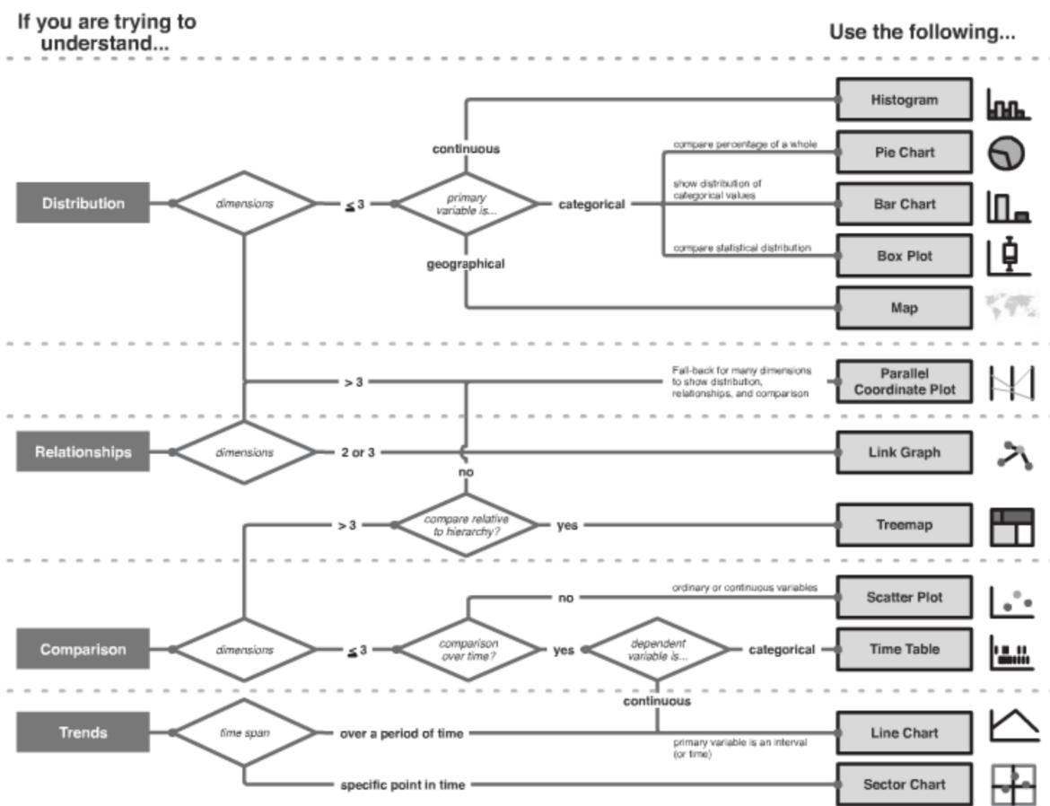
FIGURE 1.16 – Arbre de décision des représentations 2D de données utilisables en cybersécurité, en fonction du type de questions que l'on se pose sur les données, extrait de [88] (© 2009, Raffael Marty). Les représentations proposées sont uniquement en 2D.
