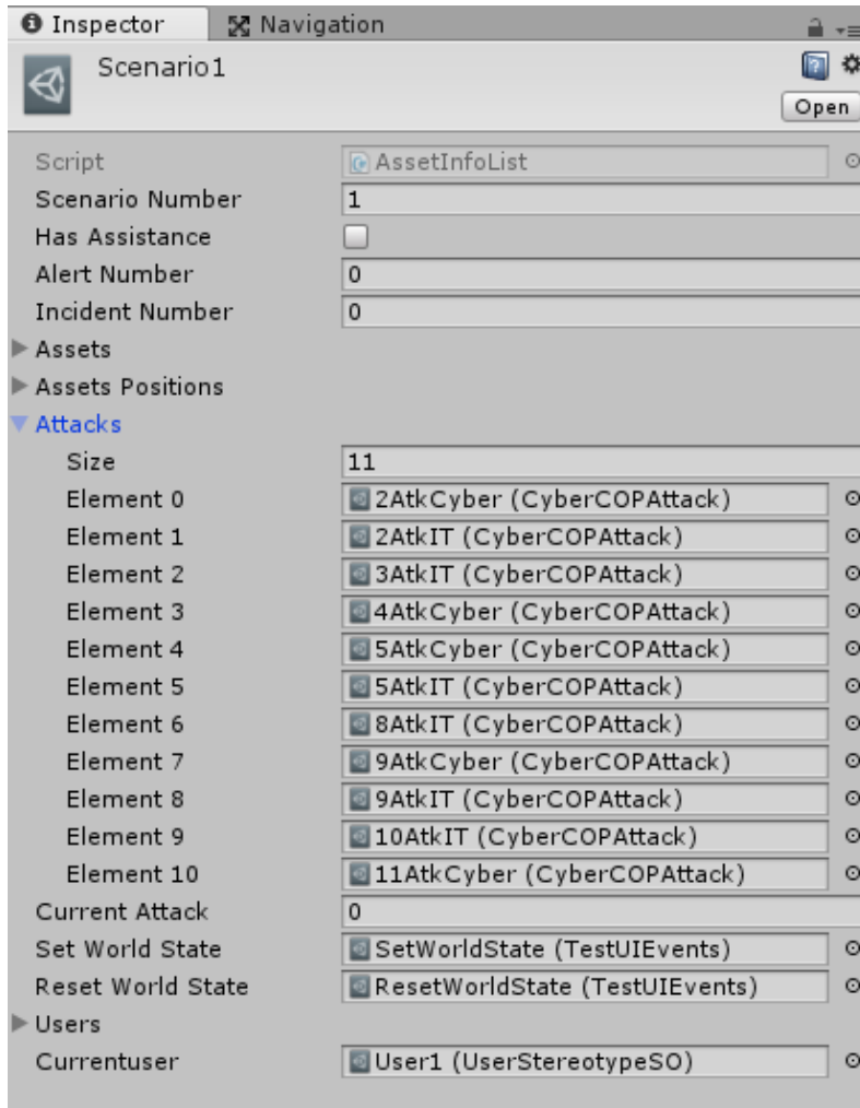
FIGURE 4.13 – Vue éditeur d'un scénario avec les informations des assets, des attaques et des utilisateurs. Ce scénario se prépare à la main en glissant-déposant les Scriptable Objects relatifs aux attaques, assets et utilisateurs. La référence à ce Scriptable Object est utilisée pour accéder aux informations durant l'exécution.
