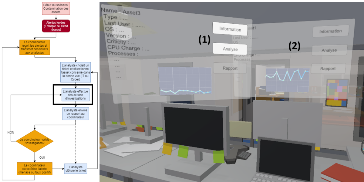
FIGURE 5.5 – (1) Menu contextuel de récupération d'informations sur l'asset concerné. (2) Les autres assets ne peuvent pas être analysés.
