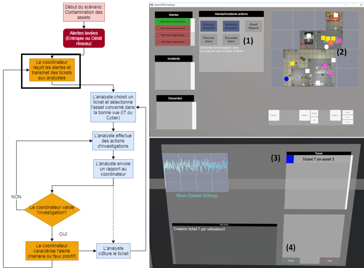
FIGURE 5.2 – Demande d'analyse par le coordinateur. Les boutons d'actions d'analyse changent de couleur (1) pour préciser que l'action de demande a été effectuée. Sur la minicarte, l'asset concerné par la demande d'analyse change de couleur (2). (3) Apparition d'une notification d'analyse sur le tableau de bord disponible dans l'environnement 3D. Un analyste doit alors le sélectionner et accepter le ticket, via un bouton en bas de l'interface (4).
