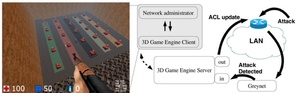
FIGURE 1.22 – Exemple d'application immersive pour la détection d'intrusions basée sur la métaphore du jeu de tir à la première personne, extrait de [59] (© 2006, ACM). L'utilisateur peut 'tirer' sur les données d'intrusion afin de les filtrer et de les signaler.
