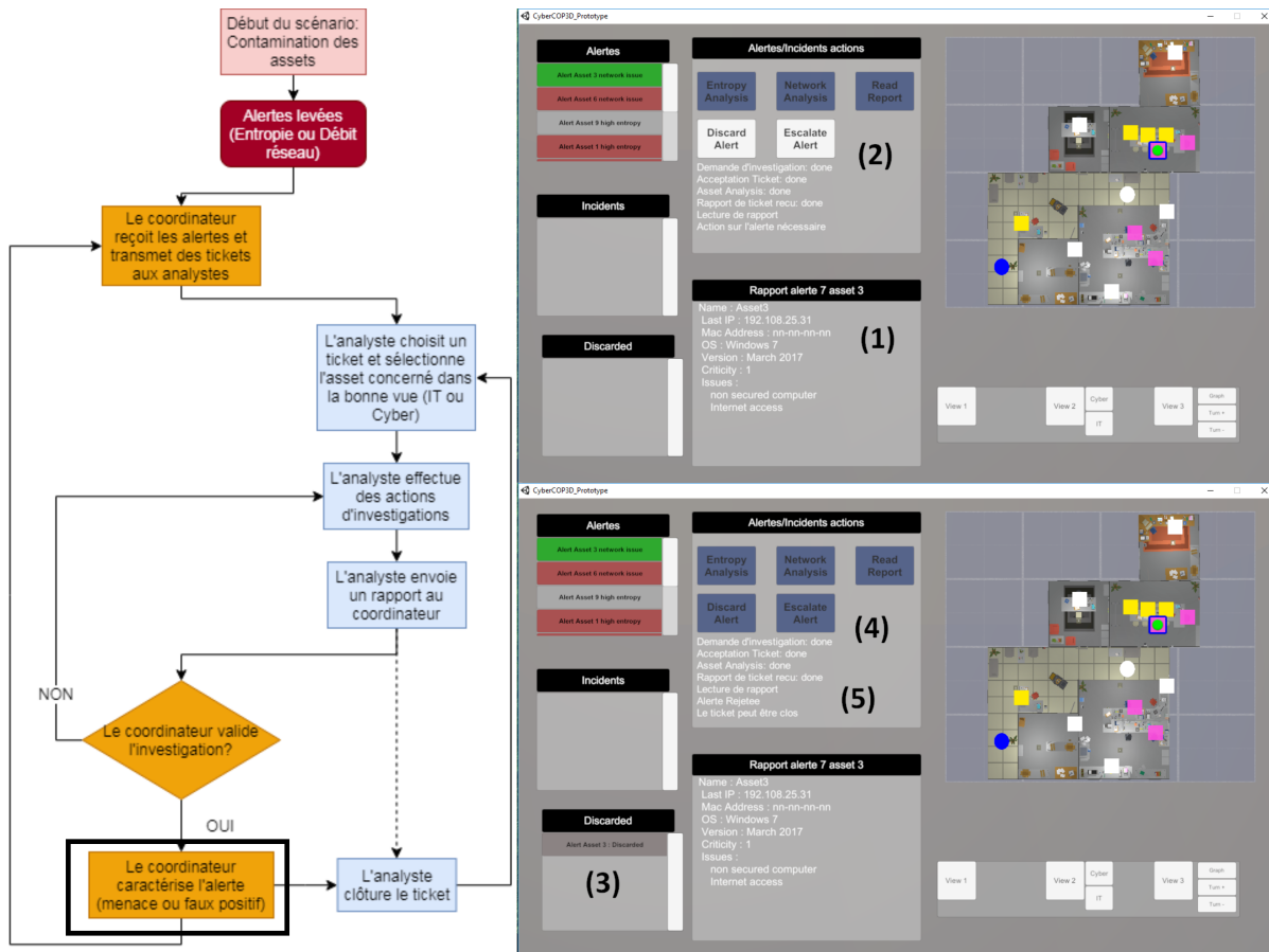
FIGURE 5.8 – (1) Lecture du rapport par le coordinateur (qui contient dans cet exemple les données de l'asset), ce qui active (2) les actions de caractérisation. Une fois l'alerte caractérisée, elle apparaît dans la liste des incidents ou des (3) faux positifs. (4) Les boutons d'actions de l'interface sont ensuite désactivés et (5) l'historique d'actions concernant le ticket est mis à jour.
