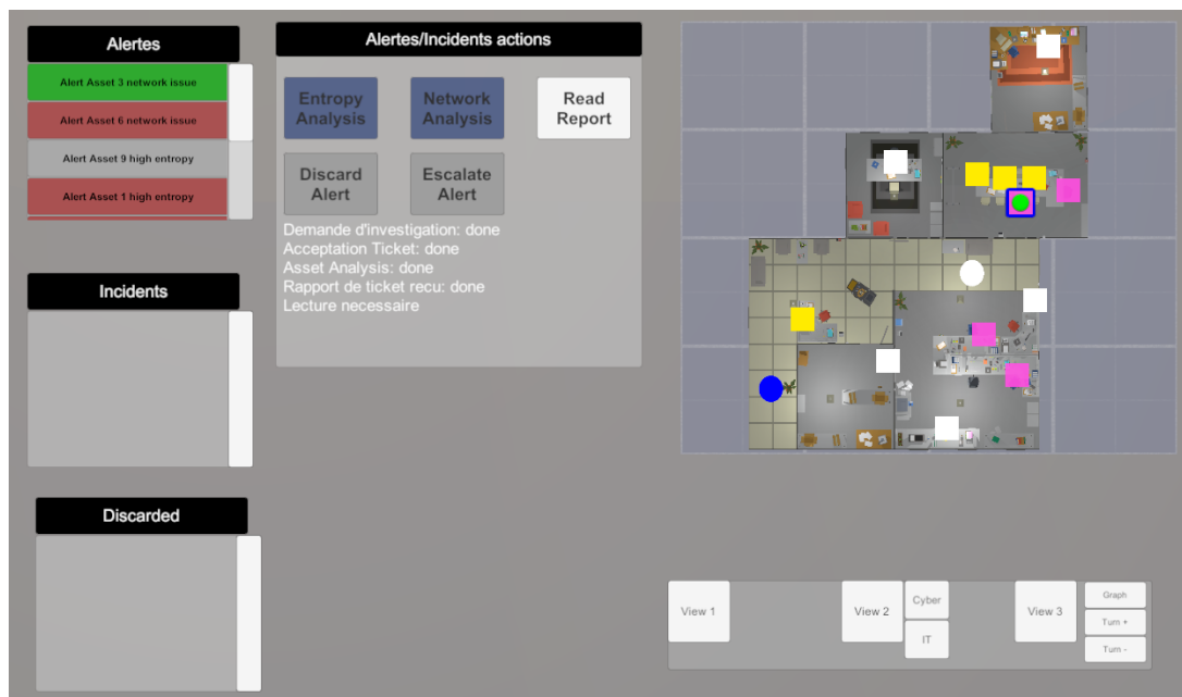
FIGURE 4.14 – Interface 2D du coordinateur, avec la liste des alertes reçues ainsi que les actions possibles. La minicarte permet de suivre l'évolution des analyses (les alertes IT et Cyber sur les assets sont représentées respectivement par des carrés jaunes et roses) et de localiser les utilisateurs (l'utilisateur local est représenté ici par un rond bleu et l'utilisateur distant par un rond blanc).
