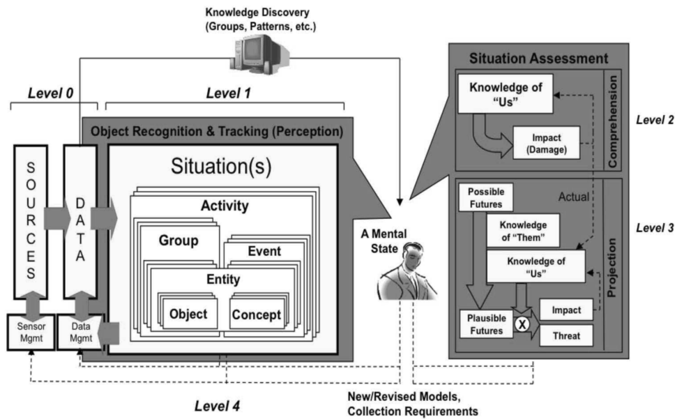
FIGURE 1.12 – Modèle de Tadda et Salerno regroupant à la fois les étapes du modèle de fusion de données JDL de Giacobe et les étapes cognitives du modèle d’Endsley, extrait de [119] (© 2010, Springer). Les différents niveaux de traitement concernent à la fois la fusion d’informations par des outils et le modèle mental d’un analyste.
