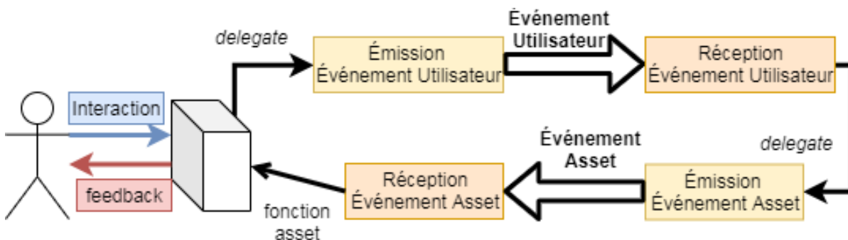
FIGURE 4.5 – Propagation d'événements, de l'interaction utilisateur à l'appel de fonction sur l'asset concerné. L'interaction déclenche un appel de fonction déléguée qui appelle une fonction d'émission d'événement utilisateur, qui est réceptionné, filtré, et transmis aux assets.
