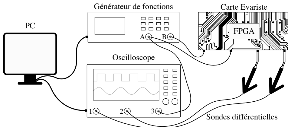
FIGURE 4.1: Banc d'expérimentation
