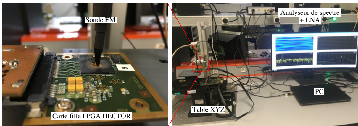
FIGURE 5.5: Banc d'expérimentation
