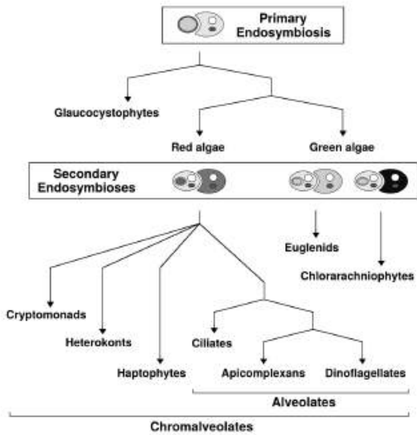
FIGURE 17 – Hypothèse Chromalvéolée)
