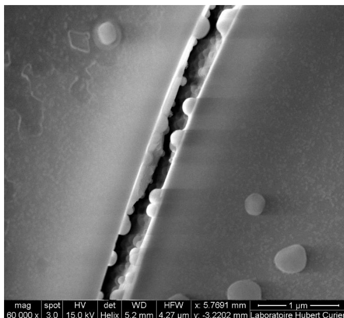
Figure 88 : image MEB d'une fissure à la surface d'un trait laser insolé à 400 µm/s et à 120 mW révélant la présence de nombreuses nanoparticules sphériques de diamètre voisin de 100 nm
