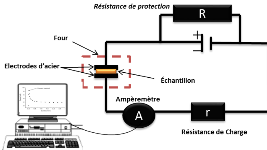
Figure 29 : schéma électrique du dispositif expérimental de poling thermique
