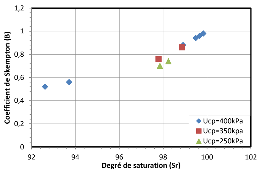
Figure 7.1. Variation de degré de saturation Sr en fonction du coefficient de Skempton B
