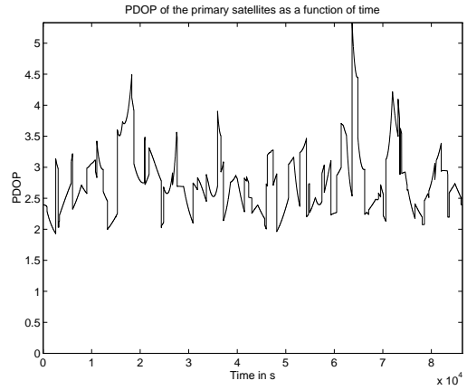
(d) PDOP of the primary satellites (first case).
