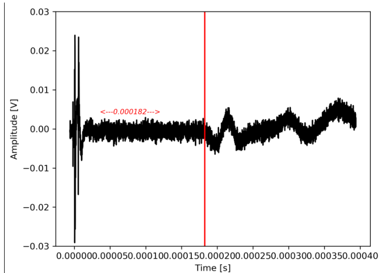
Figure II.37 : Même mesure que la figure précédente mais ici avec 3x256 stacks (ondes P)
