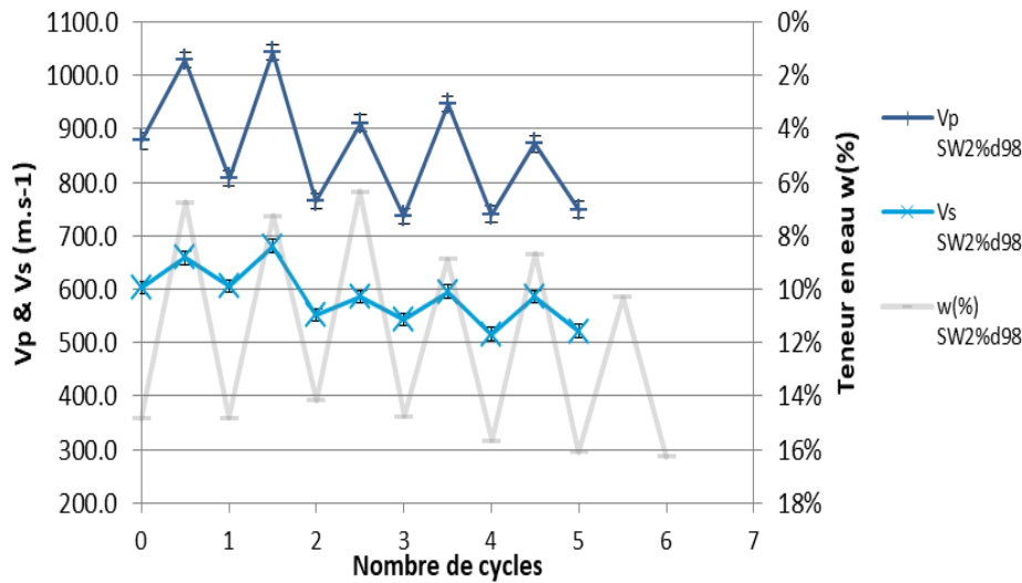
Figure IV.7 : Vitesse de propagation des ondes P et S dans les différents matériaux au cours des 6 cycles hydriques à l'eau de mer après 365 jours.
