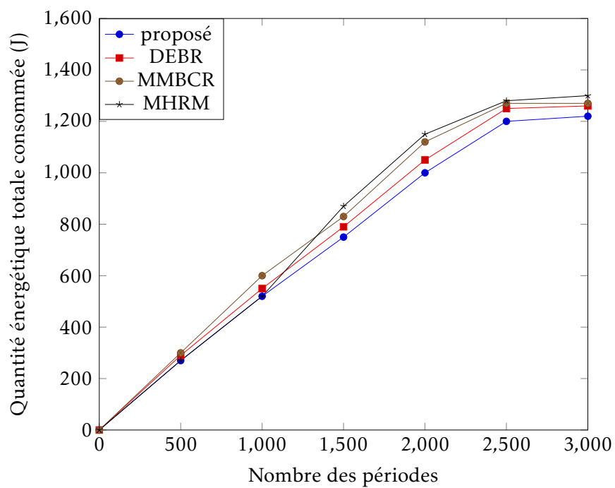
FIGURE 4.5 – Comparaison des algorithmes en termes de la consommation énergétique totale des réseaux
