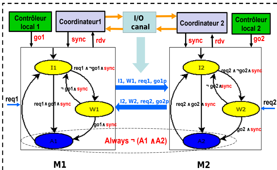
FIGURE 3.7 – établissement de la barrière de synchronisation entre deux noeuds communicants
