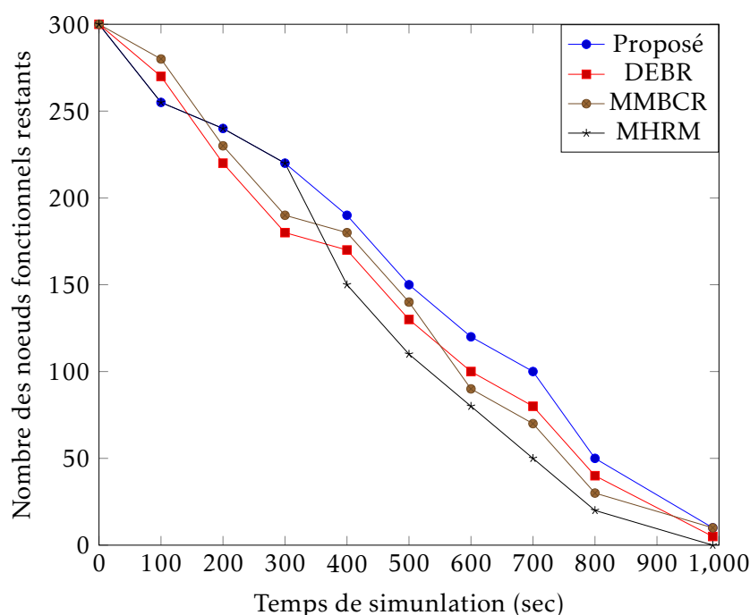
FIGURE 4.4 – Comparaison de l'algorithme proposé aux algorithmes existants en terme des durées de vie des réseaux
