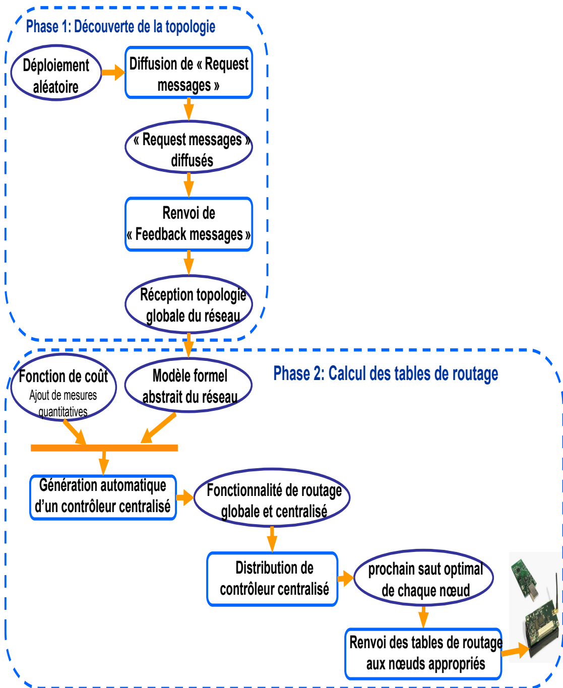
FIGURE 4.1 – une vue d'ensemble de la méthode adoptée pour la génération du protocole de routage optimal
