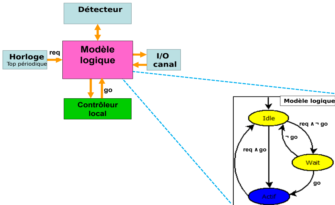
FIGURE 3.3 – Modèle formel abstrait d'un noeud-capturer
