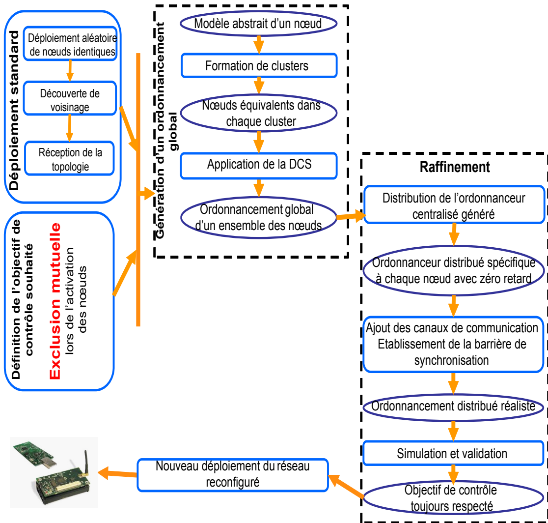
FIGURE 3.2 – Méthode proposée pour la conception et l'implémentation d'un ordonnancement automatique d'un ensemble redondant des noeuds
