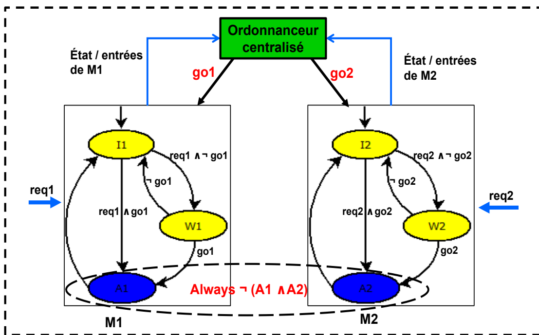
FIGURE 3.4 – Supervision centralisée appliquée à un cluster composé de deux nœuds
