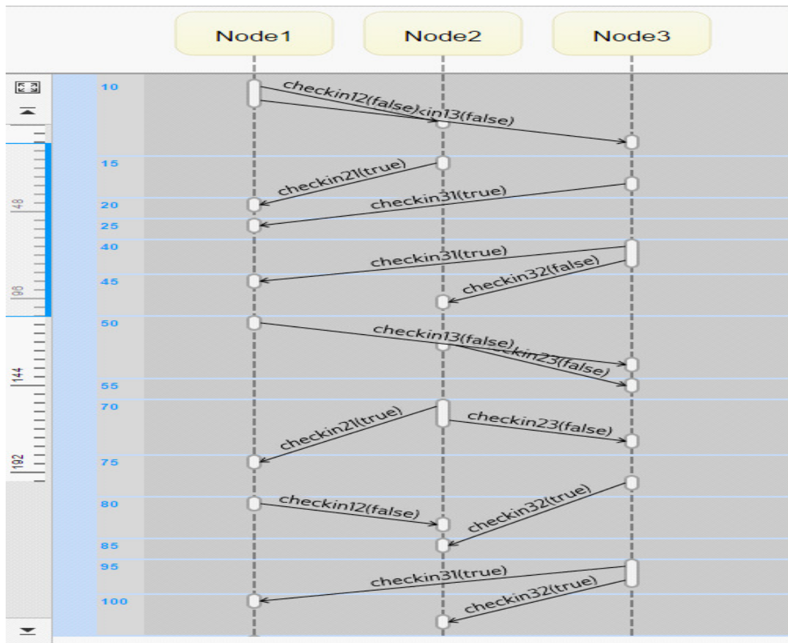
FIGURE 3.11 – Échange des messages au cours de temps entre les noeuds d'un cluster
