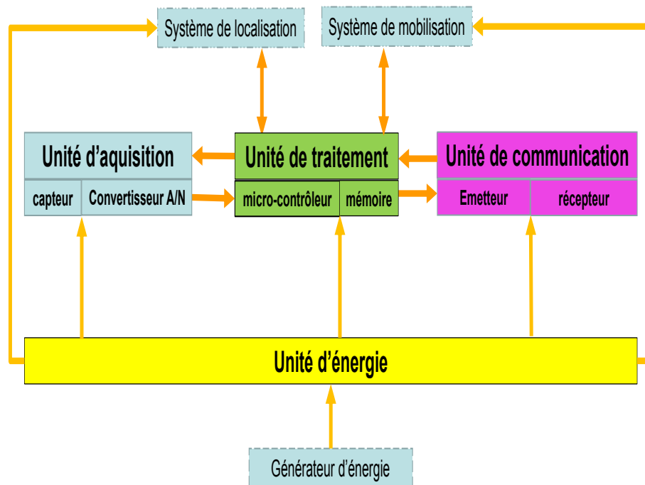
FIGURE 1.1 – Architecture d'un nœud
