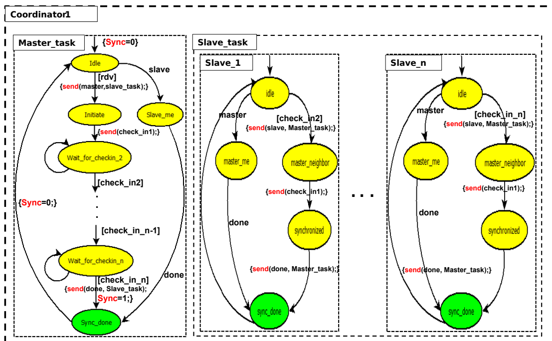
FIGURE 3.8 – établissement de la barrière de synchronisation entre deux nœuds communicants
