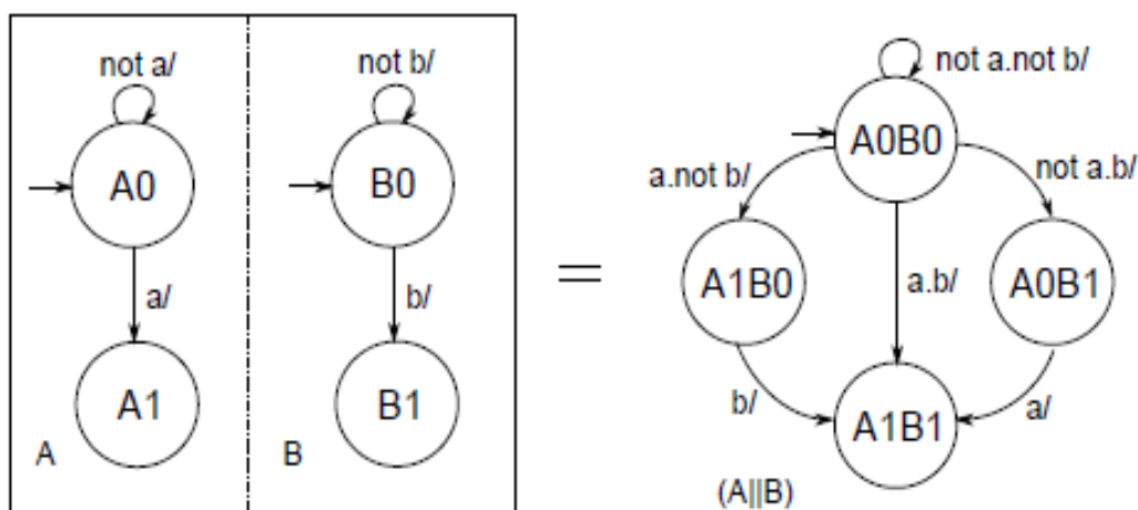
FIGURE 2.1 – Exemple de composition synchrone de deux automates
