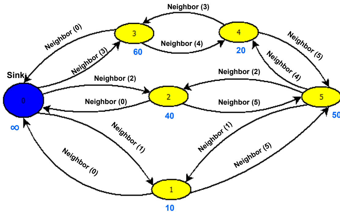
FIGURE 4.3 – Modèle formel abstrait d'un réseau de capteurs
