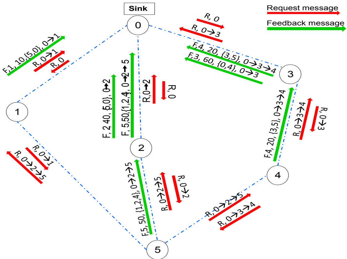
FIGURE 4.2 – Découverte de la topologie du réseau
