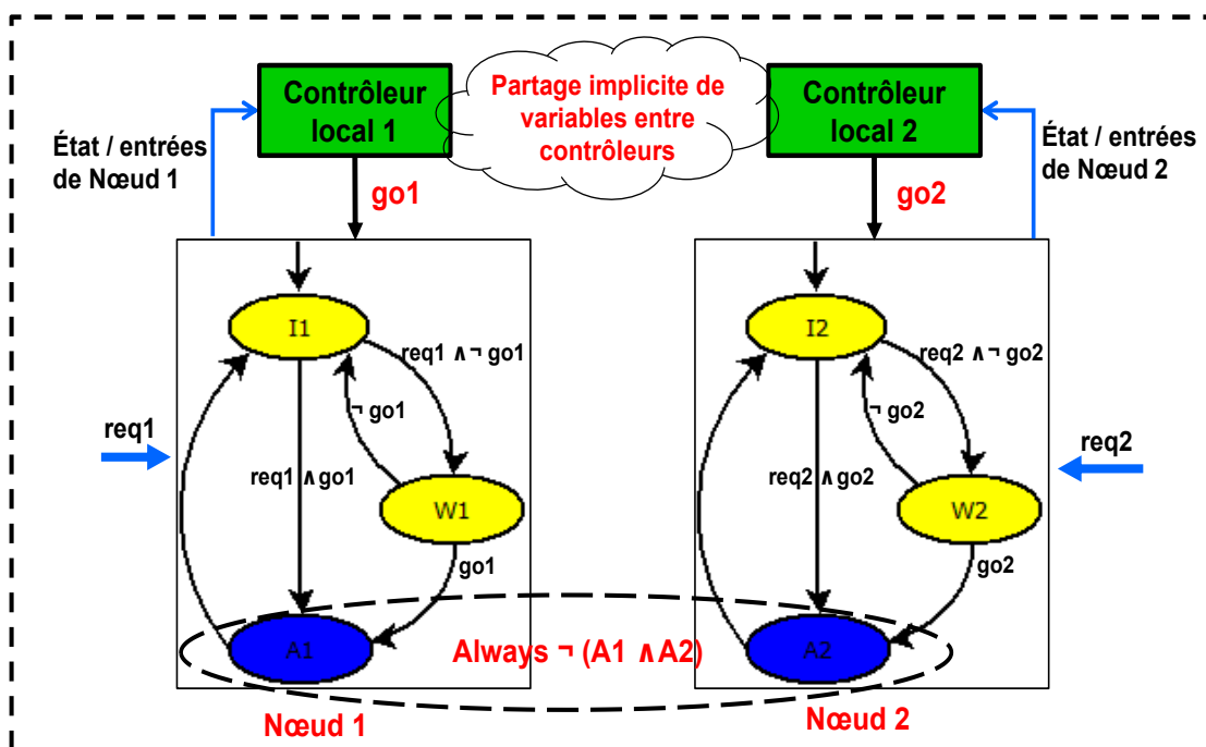
FIGURE 3.6 – Ordonnancement distribué d'un cluster formé de deux noeuds
