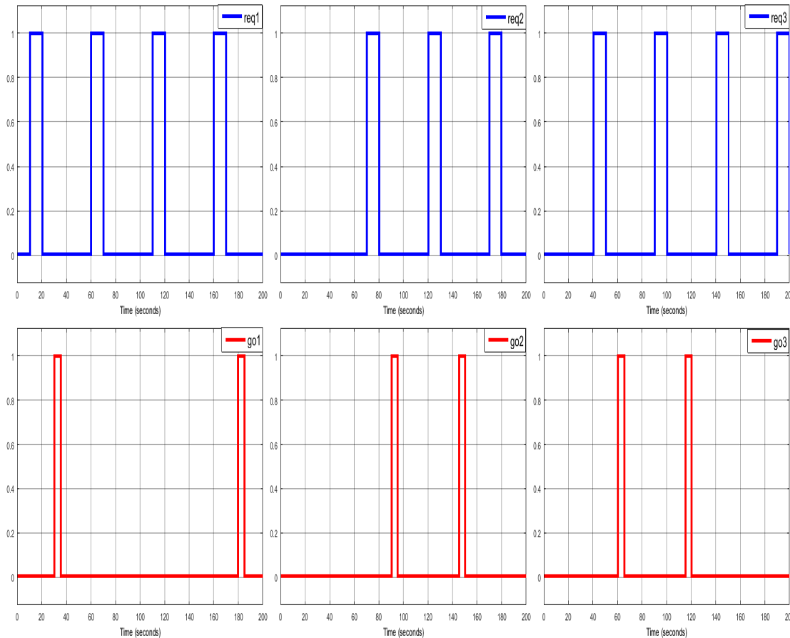
FIGURE 3.10 – Simulation d’un réseau de capteurs composé de 3 nœuds ordonné par DCS
