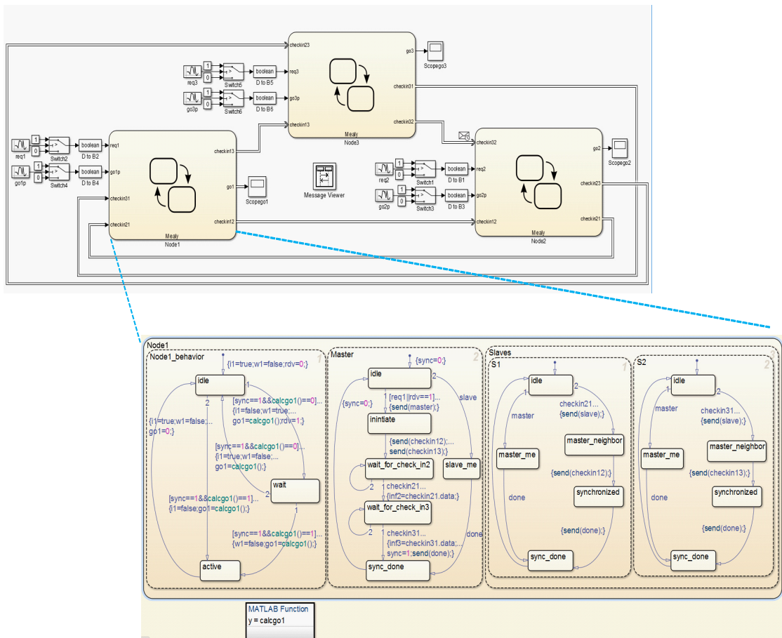
FIGURE 3.9 – Simulation d'un réseau de capteurs composé de 3 noeuds ordonné par DCS
