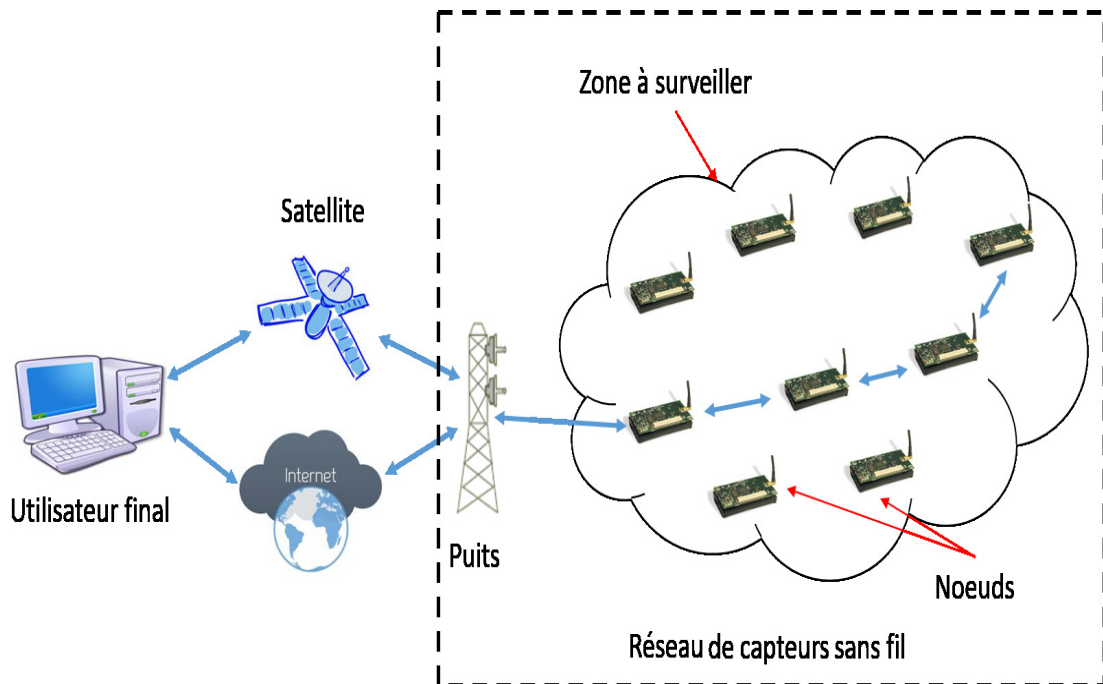
FIGURE 1.2 – Architecture d'un réseau de capteurs sans fil
