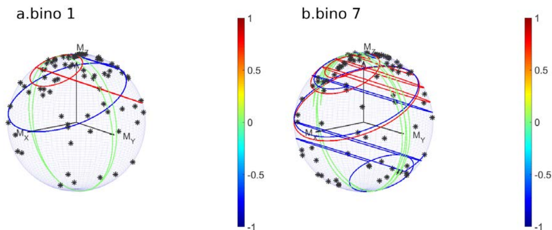
FIGURE 8.8 – Simulations des trajectoires des aimantations dans la sphère de Bloch. 3 trajectoires ont été représentées correspondant à des \Delta B_0 positif, négatif et proche de 0. Réalisées à l’aide du logiciel de simulation d’E. Van Reth, pour des binomiales 1 et 7, de durée 3 ms.
