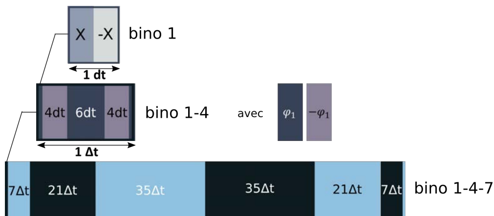
FIGURE 6.3 – Schéma explicatif de la nomenclature des impulsions binomiales composées
