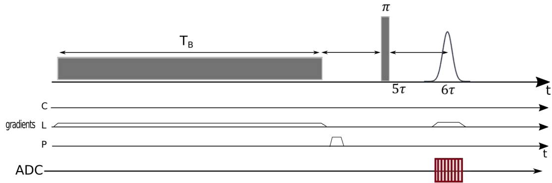
FIGURE 6.4 – Chronogramme de la séquence RFProfile.
