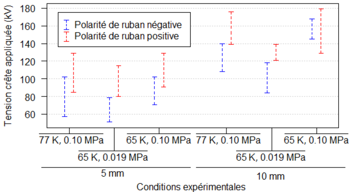
Figure 77 : Tensions de claquage V_{BD} minimales et maximales relevées pour chaque condition expérimentale dans l'azote liquide non chauffé en choc STI.
