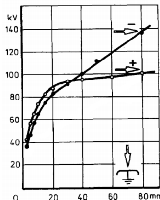
Figure 27 : Tensions de claquage dans l'azote liquide avec en fonction de la distance pour différentes polarités, en géométrie pointe-plan (rayon de courbure de la pointe = 100 \mu m). Adapté de [Fleszyński1979].
