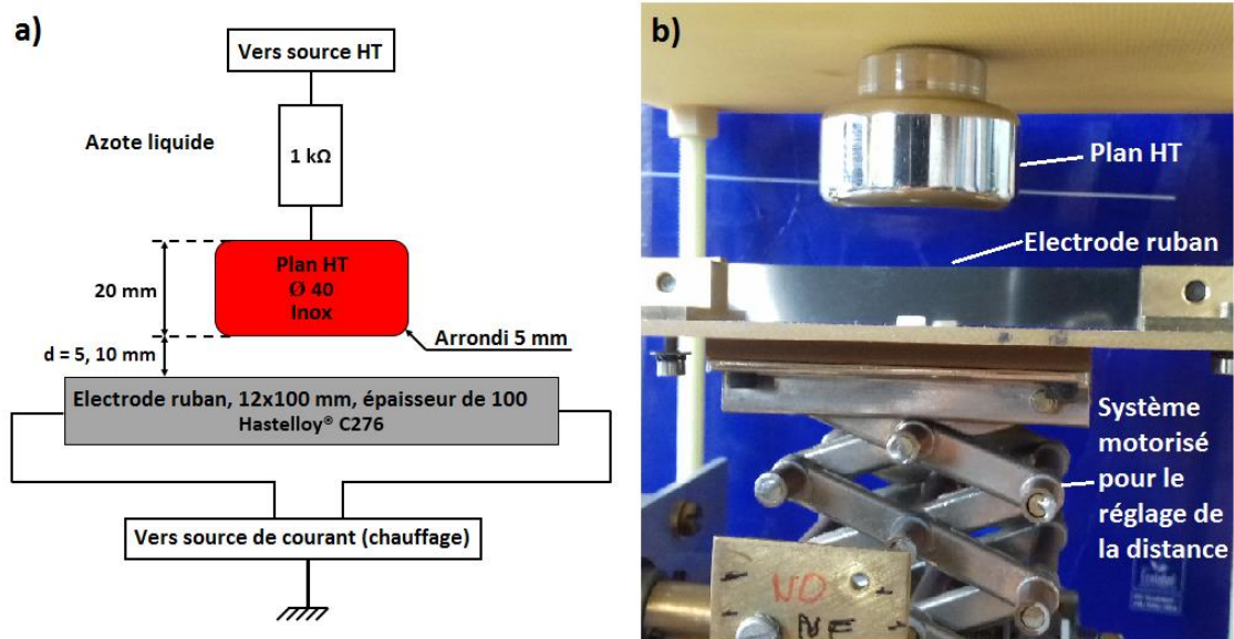
Figure 55 : Système d'électrodes utilisé pour les essais. (a) Vue schématique. (b) Photographie
