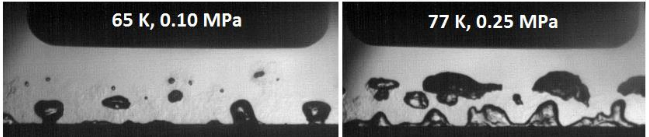
Figure 101 : Condensation des bulles d'azote dans un bain d'azote sous-refroidi, 100 ms après le début du chauffage transitoire. (a) Bain d'azote liquide à T = 65 K, P = 0.10 MPa. (b) Bain d'azote liquide à T = 77 K, P = 0.25 MPa.
