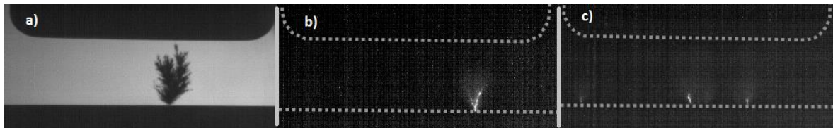
Figure 88 : Images de streamers négatifs ne menant pas au claquage. Azote liquide à 0.10\text{ MPa} , distance inter-électrode de 10\text{ mm} . (a) A 77\text{ K} , onde LI, 145\text{ kV} . (b) A 65\text{ K} , onde SI, 144\text{ kV} (c) A 65\text{ K} , onde LI, 185\text{ kV} .
