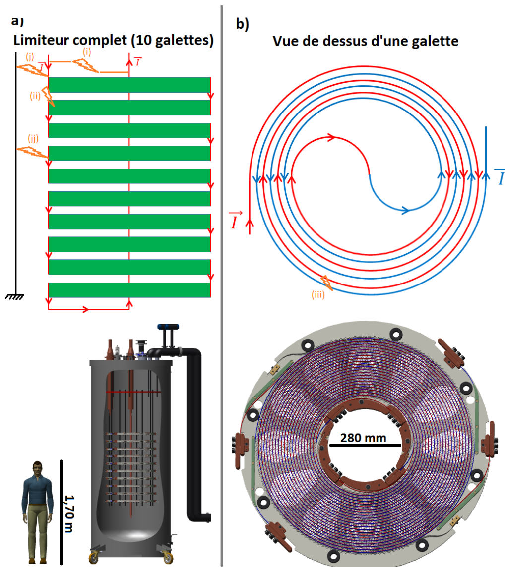
Figure 41 : Schéma simplifié et Modèle 3D du limiteur de courant développé dans le cadre du projet FastGrid. (a) Limiteur complet (10 galettes en séries) (b) Vue de détail d'une galette
