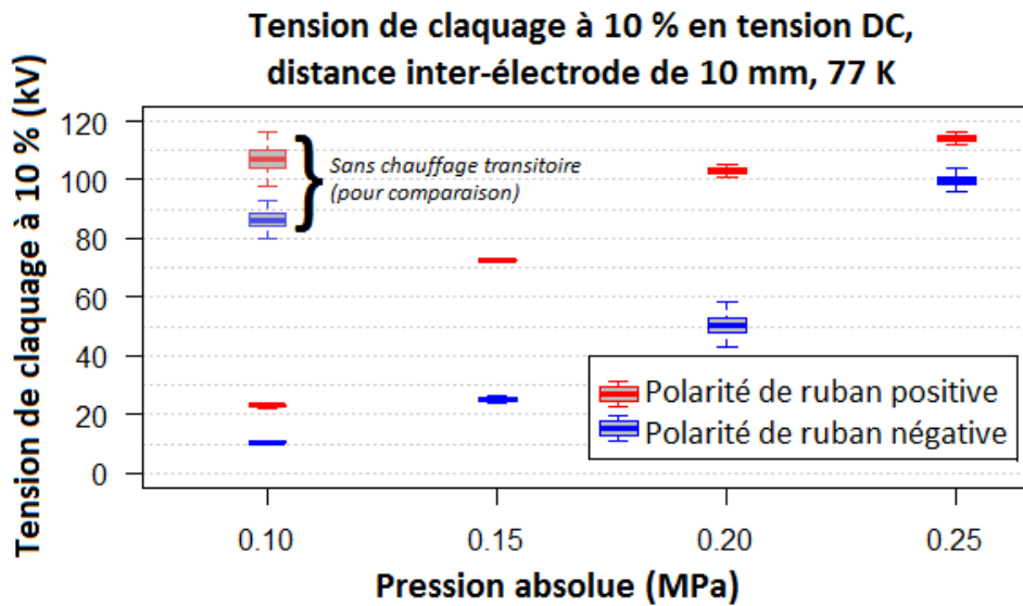
Figure 128 : Tensions de claquage V_c^{10\%} , en polarité positive et négative, T = 77\text{ K} , entre P = 0.10 et 0.25\text{ MPa} , ainsi que la référence sans chauffage à P = 0.10\text{ MPa} .
