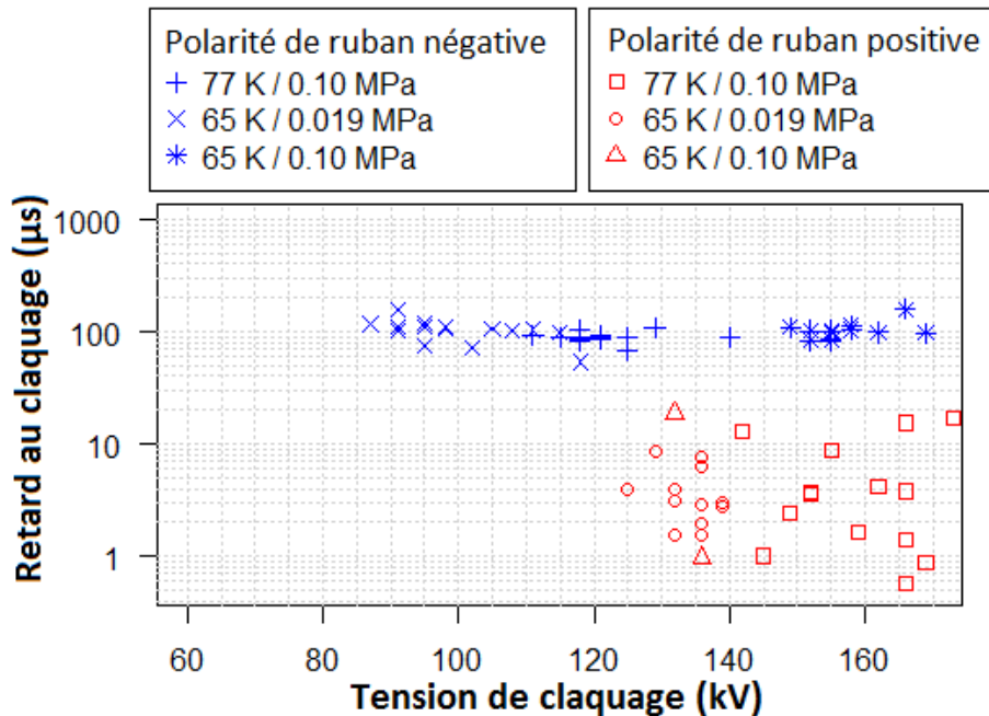
Figure 79 : Retards au claquage t_c dans l'azote liquide en fonction de la tension de claquage, en onde STI, pour trois conditions expérimentales différentes. d = 10 mm.
