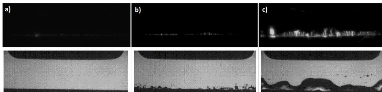
Figure 104 : Décharges non disruptives dans le film d'azote gazeux, et images de l'ébullition avec différents retards. (a) \Delta t = 5 ms. (b) \Delta t = 15 ms. (c) \Delta t = 40 ms.
