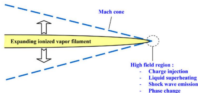
Figure 13 : Modèle de propagation des streamers de 2 nd mode : analogie avec une source d'énergie mobile [Lesaint2016]
