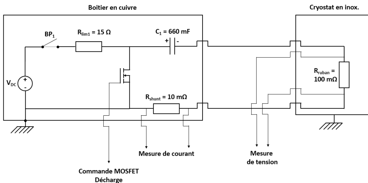
Figure 59 : Schéma électrique du système de chauffage transitoire connecté au cryostat avec les systèmes de mesure
