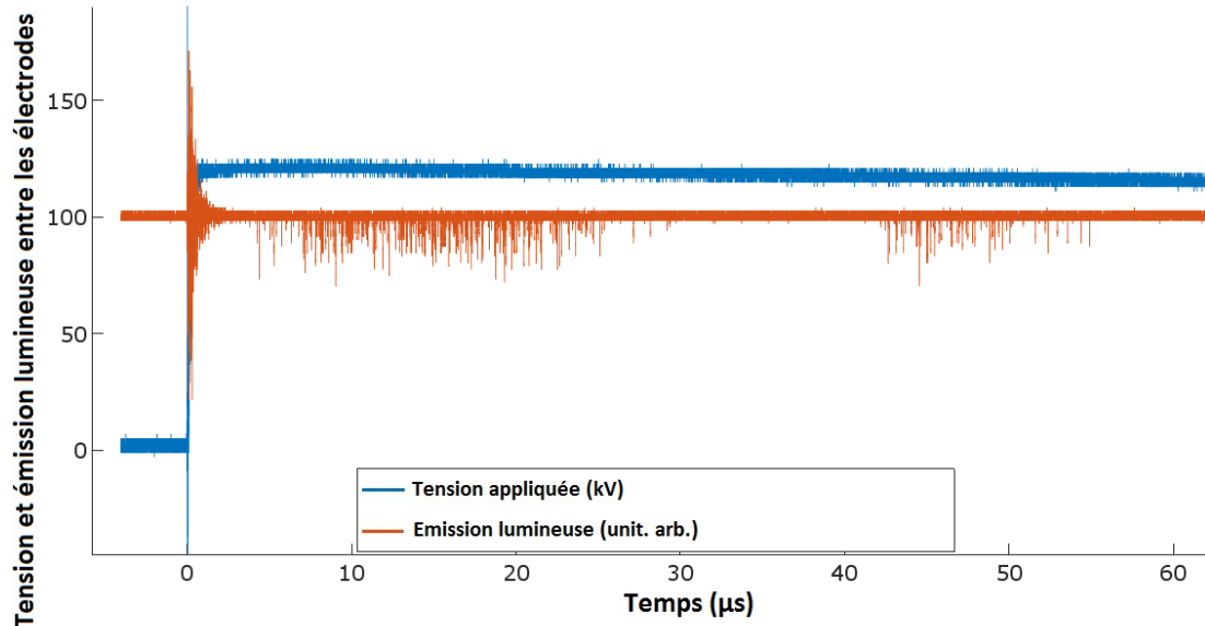
Figure 74 : Signaux lumineux caractéristiques d'un streamer ne menant pas au claquage en conditions de sous-refroidissement et en polarité de ruban négative. T = 65 \text{ K} , P = 0.10 \text{ MPa} , distance inter-électrode de 10 mm, V_a = 121 \text{ kV} .
