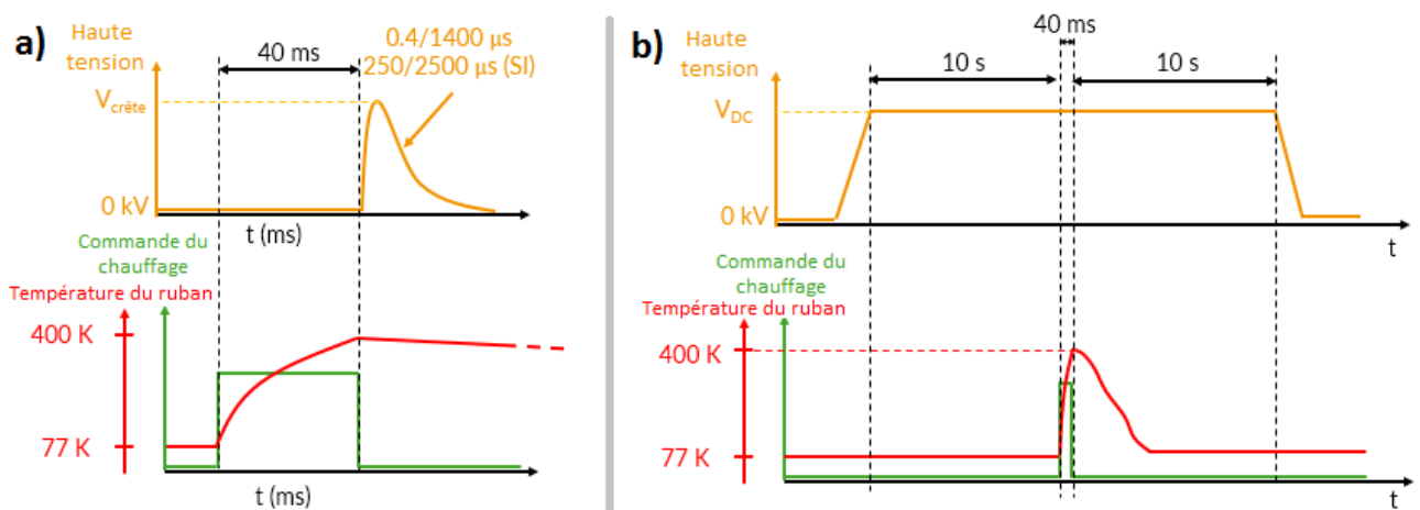
Figure 66 : Illustration du protocole de montée de descente
