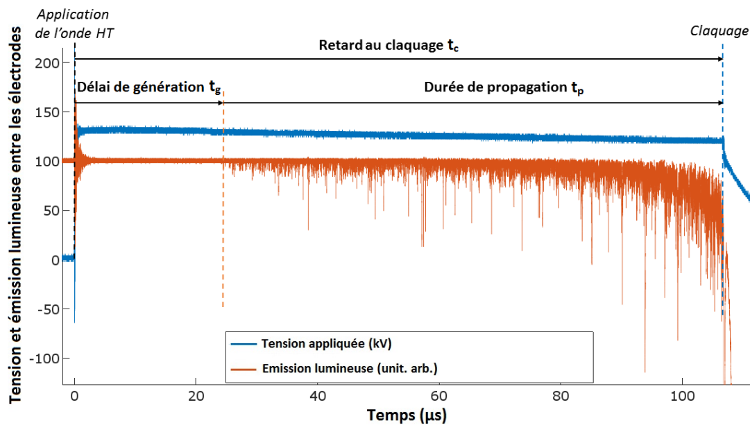
Figure 72 : Tension instantanée et lumière pré-claquage émise (signal du PM). Azote liquide à 77 K, 0.10 MPa, d = 10 mm, polarité de ruban négative, V_a = 129 kV sur le plan HT.
