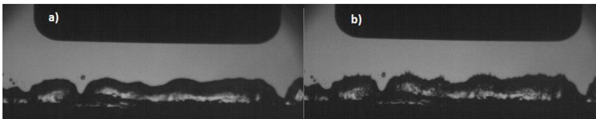
Figure 105 : Déformation des bulles suite à l'application de l'onde HT ( SI , V_a = 91 kV sur l'électrode ruban), ne menant pas au claquage. T = 77 K, P = 0.10 MPa, d = 10 mm, \Delta t = 40 ms. (a) Image avant l'application du choc HT. (b) Image suivante ( 250 \mu s plus tard), choc HT en cours d'application.
