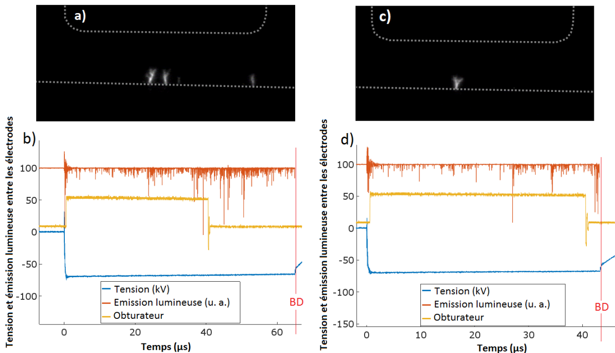
Figure 107 : Streamers positifs de 1 er mode «en buisson» dans l'azote chauffé. T = 77 K, P = 0.10 MPa, \Delta t = 5 ms, d = 10 mm, polarité positive ( V_0 = -71 kV). (a, c) Images prises durant la propagation avec la caméra à intensificateur. (b, d) Oscillogrammes correspondants.
