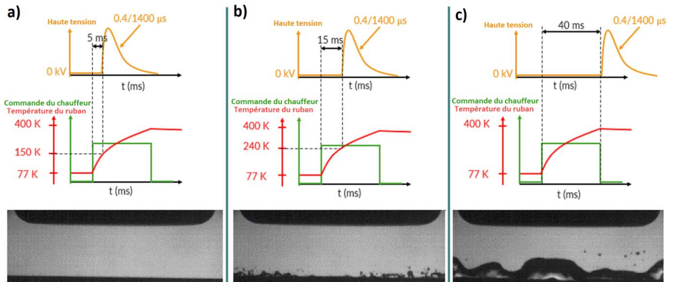
Figure 102 : Protocole d'essai réalisé en choc 0.4 / 1400 \mu s dans l'azote liquide chauffé transitoirement, et images typiques de l'ébullition juste avant le déclenchement de l'onde HT. (a) Avec un retard \Delta t = 5 ms (un fin film de bulles est présent autour du ruban). (b) Avec un retard \Delta t = 15 ms. (c) Avec un retard \Delta t = 40 ms.
