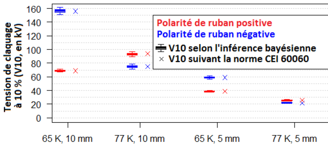
Figure 70 : Comparaison de quelques évaluations de tension de claquage à 10 % déterminées à partir des mêmes données expérimentales, via la norme CEI60060, et via le calcul bayésien (distribution de Weibull)
