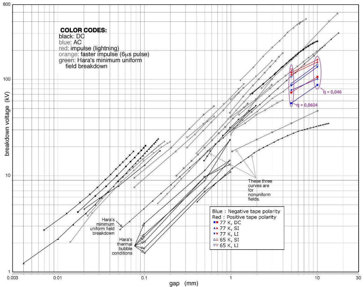
Figure 95 : Superposition des résultats expérimentaux obtenus dans l'azote liquide non chauffé avec des résultats de la littérature. Les données en couleur sont des ajouts sur la courbe présentée dans [Sauers2009]. Voir en Figure 18 pour la courbe initiale.
