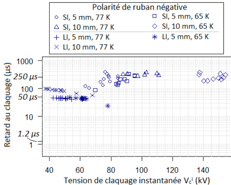
Figure 90 : Retards au claquage dans l'azote liquide en fonction de la tension instantanée de claquage V_c^i , en onde SI et LI, à 77 K et 0.10 MPa, pour deux distances inter-électrodes et en polarité négative.
