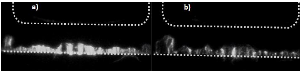
Figure 103 : Images de décharges filamenteuses dans la vapeur entourant l'électrode ruban chauffée. Azote liquide à T = 77 K, P = 0.10 MPa, d = 10 mm, délai \Delta t = 40 ms entre le début du chauffage et l'onde HT STI ( 0.4 / 1400 \mu s), obturateur ouvert entre 400 ns et 10 \mu s après le début du choc HT. (a) Décharges négatives, V_a = 93 kV sur l'électrode plane. (b) Décharges positives, V_a = -101 kV
