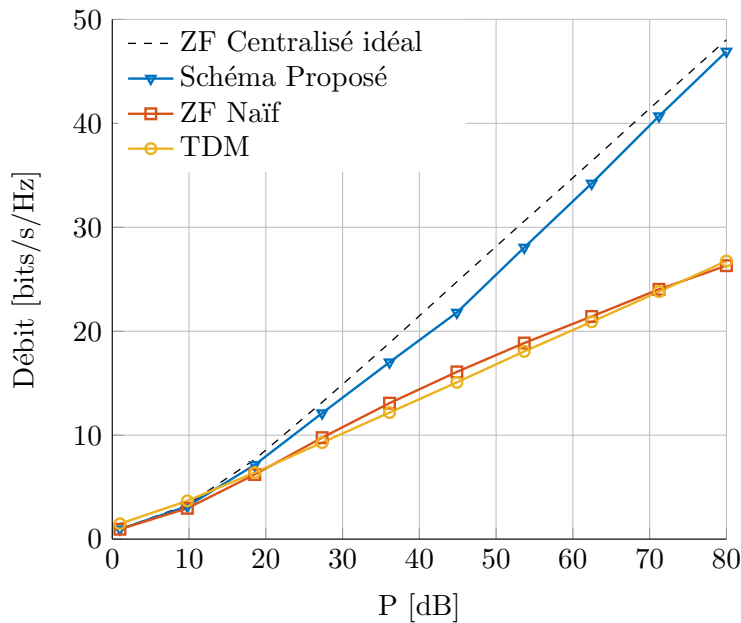
FIGURE I.4 – Débit total pour le cas où l'information de canal du RX 1 est « locale » et celle de RX 2 est « opposée ».
