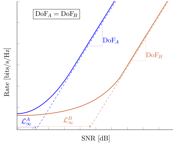
FIGURE I.2 – Illustration qualitative de l'approximation affine de deux systèmes différents avec le même DoF (pente) mais un décalage de débit différent \mathcal{R}_\infty = \text{DoF} \mathcal{L}_\infty .
