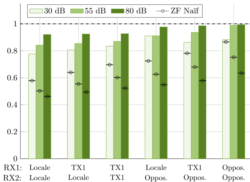
FIGURE I.5 – Pourcentage du débit centralisé « idéal » atteint par le schéma proposé et par zéro-forçage naïf pour P \in \{30, 55, 80\} dB.
