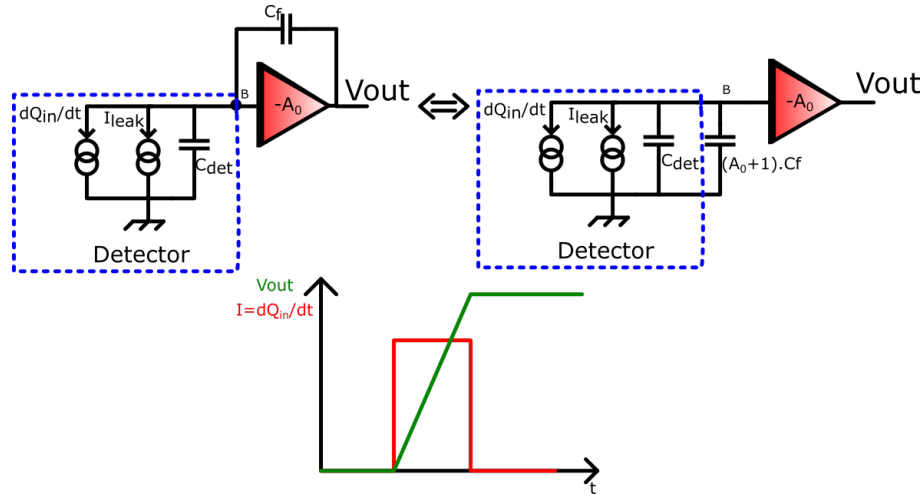
FIGURE 2.2 – Illustration de l'effet Miller dans un CSA
