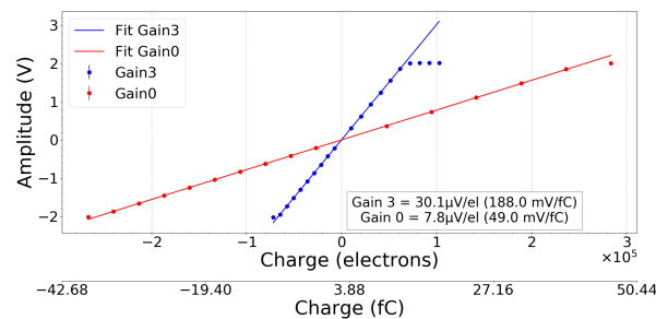
FIGURE 3.6 – Variation d'amplitude pour les deux modes de gain de l'ASIC (gain 1 et gain 4) dans les deux modes de polarité, anodes et cathode.
