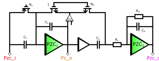
FIGURE 4.7 – Schéma de l'étage de filtrage; les deux premières parties agissent comme une suppression zéros-poles, le dernier amplificateur agit comme un filtre passe bas. Une résistance R_c permet de gagner un ordre sur le filtre de manière astucieuse.
