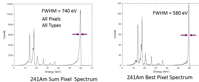
FIGURE 3.4 – Spectre de la source d' ^{241}Am effectué à -6^\circ C . A gauche les spectres sommés des pixels, à droite le spectre du meilleur pixel
