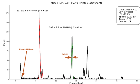
FIGURE 3.8 – Superposition de source d' ^{241}\text{Am} et de ^{55}\text{Fe} sur le système refroidit à -8^\circ\text{C} . la courbe rouge correspond aux deux raies de Fer K_\alpha et K_\beta à respectivement 5.9 et 6.4 keV. La courbe verte correspond à la raie L_\alpha de l' ^{241}\text{Am} à 13.9 keV.
