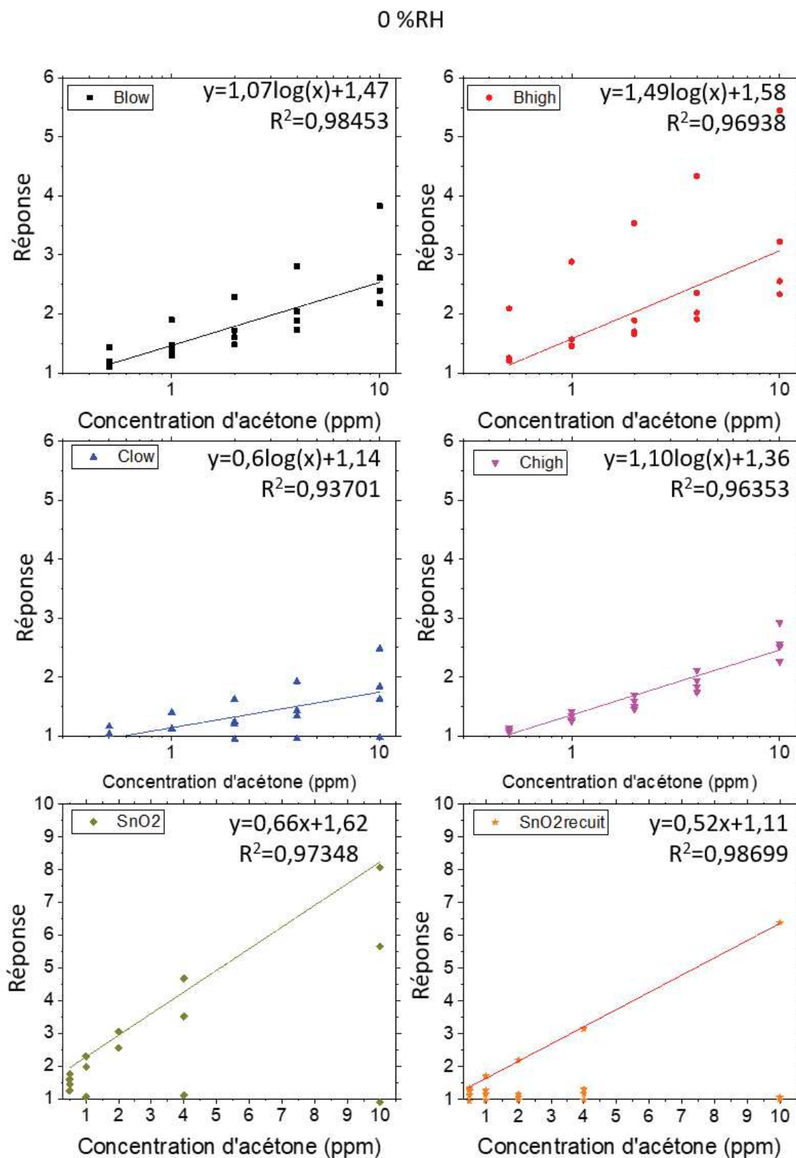
FIGURE VI.26: Evolution de la réponse des dispositifs en fonction de la concentration d'acétone en condition sèche et à 370 °C.
