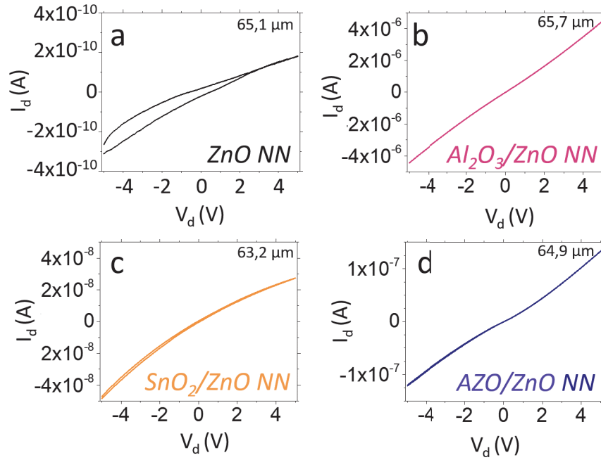
FIGURE III.16: Caractéristiques électriques 75 jours après intégration de dispositifs à base de nanonet de ZnO : a) sans passivation, b) passivés Al_2O_3 , c) passivés SnO_2 et d) passivés AZO.
