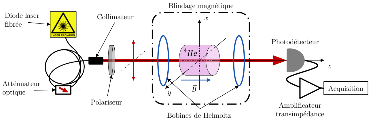
Figure 13 : Schéma de l'expérience d'effet Hanle en absorption en alignement.
