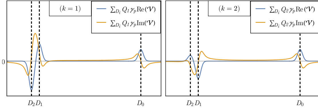
Figure 22 : Allure de la dépendance fréquentielle des propriétés d'absorption (bleu) et de dispersion (orange) de l'hélium liées à la population ( k=0 ), à l'orientation ( k=1 ) ou à l'alignement ( k=2 ) autour des transitions atomiques 2^3S_1 \rightarrow 2^3P . Toutes les courbes sont normalisées pour donner la même intensité à la raie D_0 .
