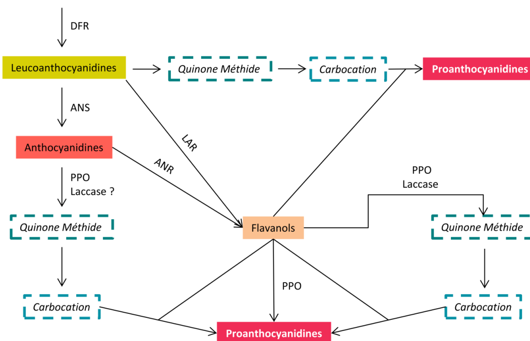
Figure 15 : Les potentielles voies de polymérisation des flavanols Schéma adapté de Dixon et al., 2005 et Terrier et al., 2009
