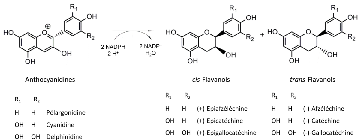
Figure 13 : Réaction catalysée par l'anthocyanidine réductase (ANR)
