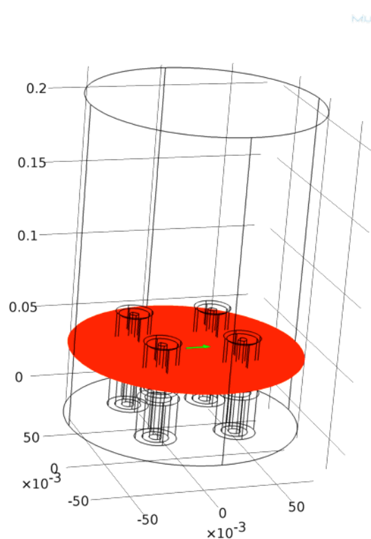
Figure. VII.5 Coupe dans ROSAE-III, section suivant le milieu des aimants (Sec-AA), simulée par COMSOL® Multiphysics.
