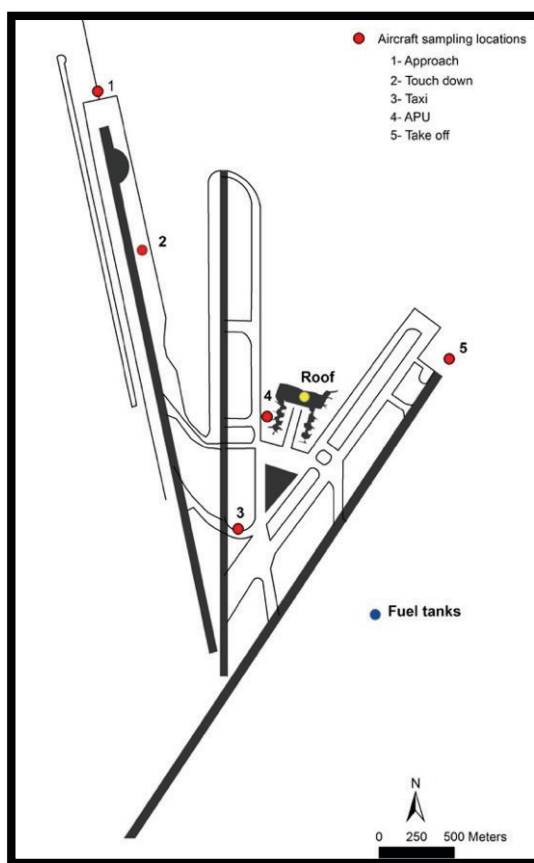
Figure 2: Localisation des sites de mesure pour les campagnes de signatures effectuées à l'aéroport de Beyrouth (Octobre 2014 et Juin 2015)
