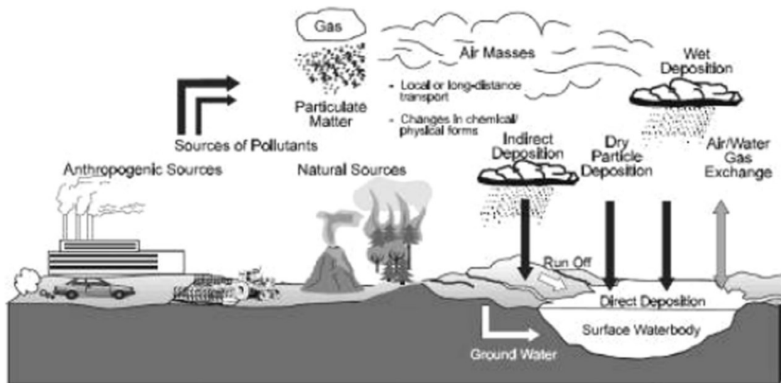
Figure 8. Dépôt sèches et humides des HAPs dans l'atmosphère (d'après Abdel-Shafy and Mansour, 2016).
