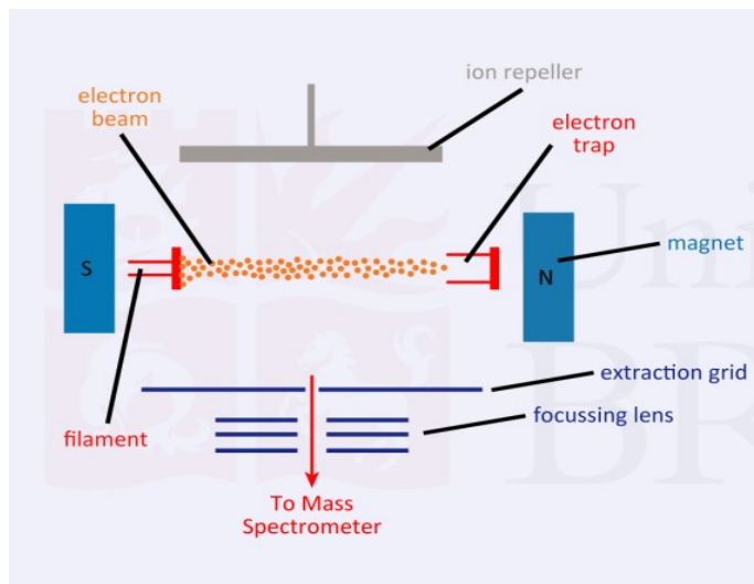
Figure 24. Représentation schématique d'une source d'ionisation par impact électronique (d'après University of Bristol, 2014)
