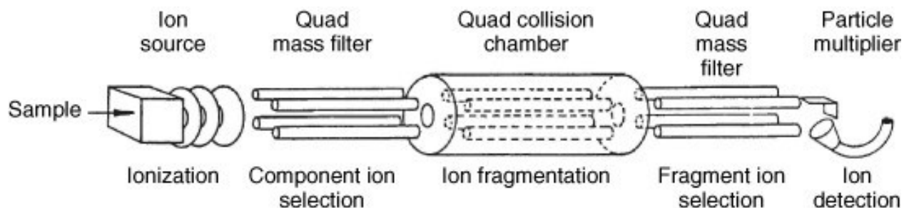
Figure 26. Schéma d'un spectromètre de masse quadripolaire triple (TQMS) (d'après Kero et al., 2005)
