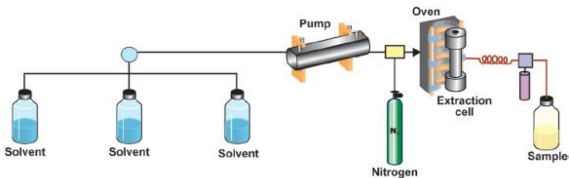
Figure 18. Représentation schématique d'une extraction ASE (d'après Dorich et al., 2008)
