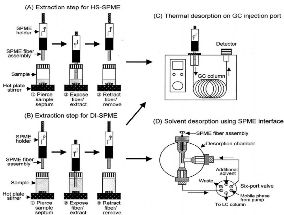
Figure 20. Procédés d'extraction par espace de tête et d'immersion par fibre SPME, et systèmes de désorption pour les analyses par GC et LC (d'après Kataoka et al., 2000)
