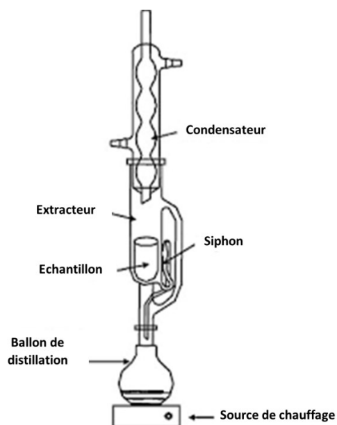
Figure 17. Schéma d'un soxhlet (d'après Luque de Castro and Priego-Capote, 2010)
