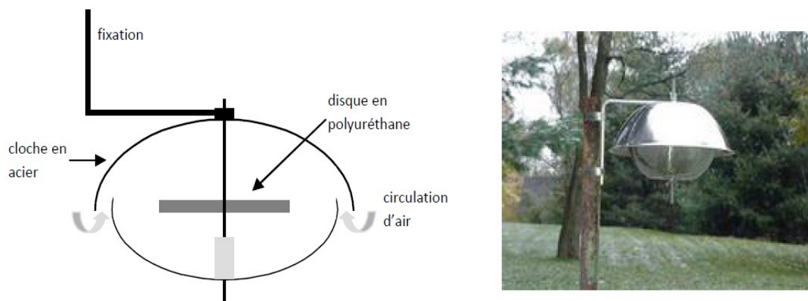
Figure 15. Schéma et photo d'un capteur passif de type PUF (« flying saucer design ») (d'après Harner et al., 2006b)
