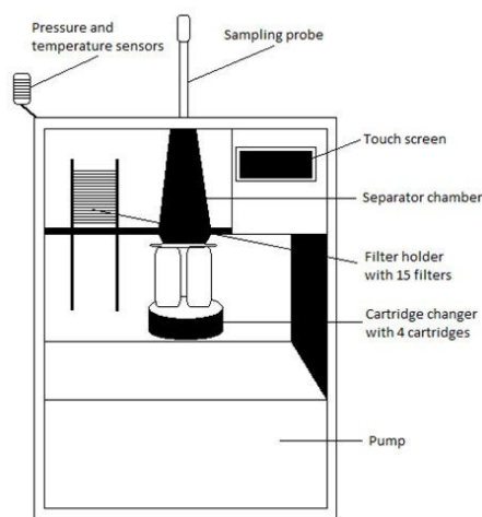
Figure 14. Schéma d'un échantillonneur actif d'air à volume élevé conçu pour l'échantillonnage extérieur (d'après MonAirNet, 2007)
