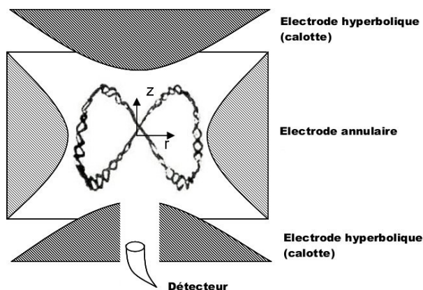
Figure 28. Trajectoire en 8 tridimensionnel des ions dans une trappe (d'après L.S.A., 2008)
