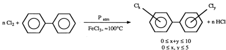
Figure 11. Réaction de synthèse des PCBs
