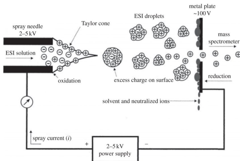
Figure 23. Processus d'ionisation ESI (d'après Staniforth and Stavros, 2013)
