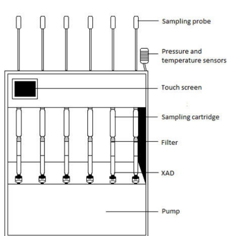
Figure 13. Schéma d'un échantillonneur actif d'air à faible volume conçu pour l'échantillonnage intérieur (d'après MonAirNet, 2007)
