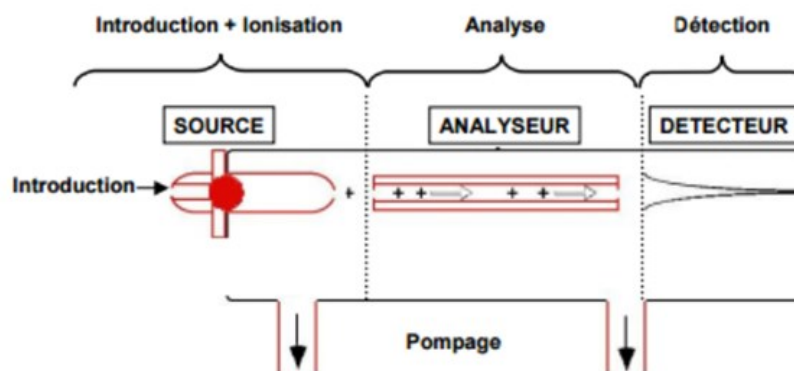
Figure 22. Composants généraux d'un spectromètre de masse (d'après Czeszak, 2003)
