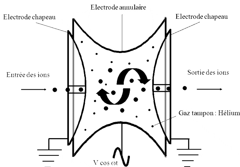
Figure 27. Représentation schématique d'une trappe ionique (modifiée de Droit, 2007)
