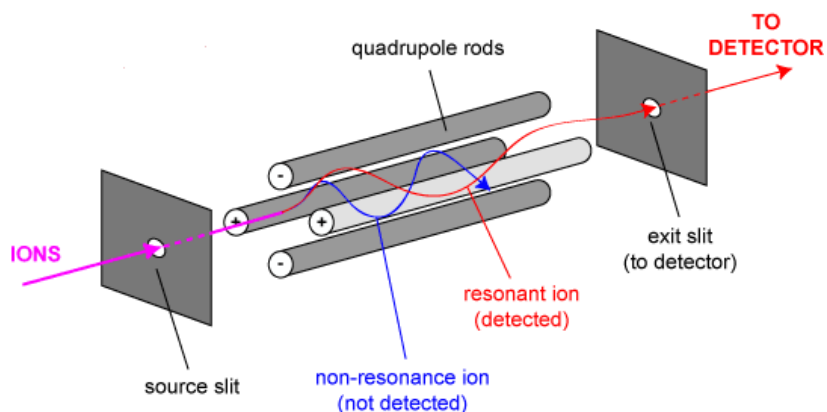
Figure 25. Schéma d'un analyseur quadripolaire (d'après Yinon, 2007)
