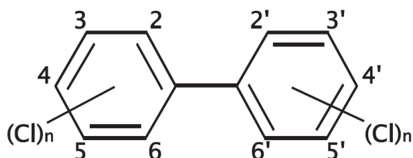
Figure 10. Structure chimique générale des polychlorobiphényles
