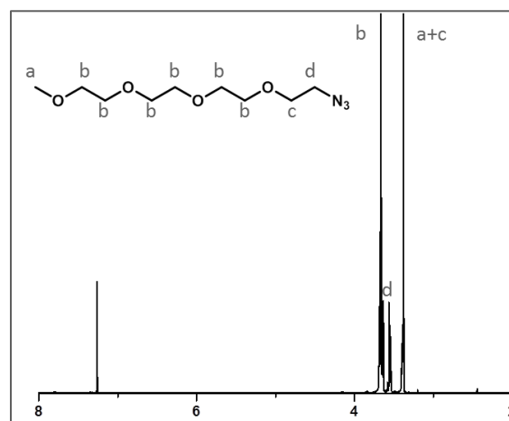
Figure 108 : RMN ^1\text{H} ( \text{CDCl}_3 ) de l'azoture PEGylé.
