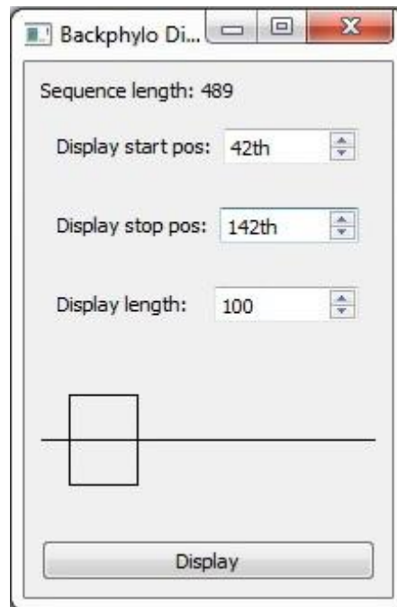
Figure 121 : Interface générale de BackPhylo, interface de sélection du display du newick. La ligne en bas représente la longueur de l'alignement de séquences et le carré représente la portion que l'on souhaite afficher dans l'arbre.
