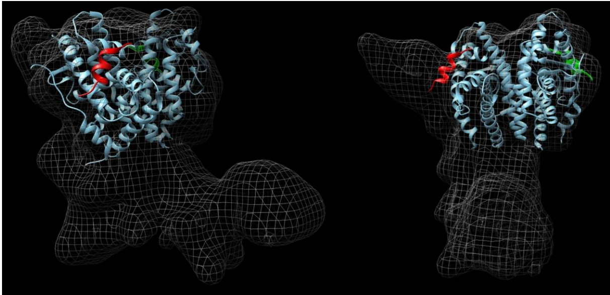
Figure 104 : Positionnement d'une structure cristallographique des LBD de ERR \alpha avec un petit fragment de PGC-1 \alpha dans la carte de cryo-ME.
