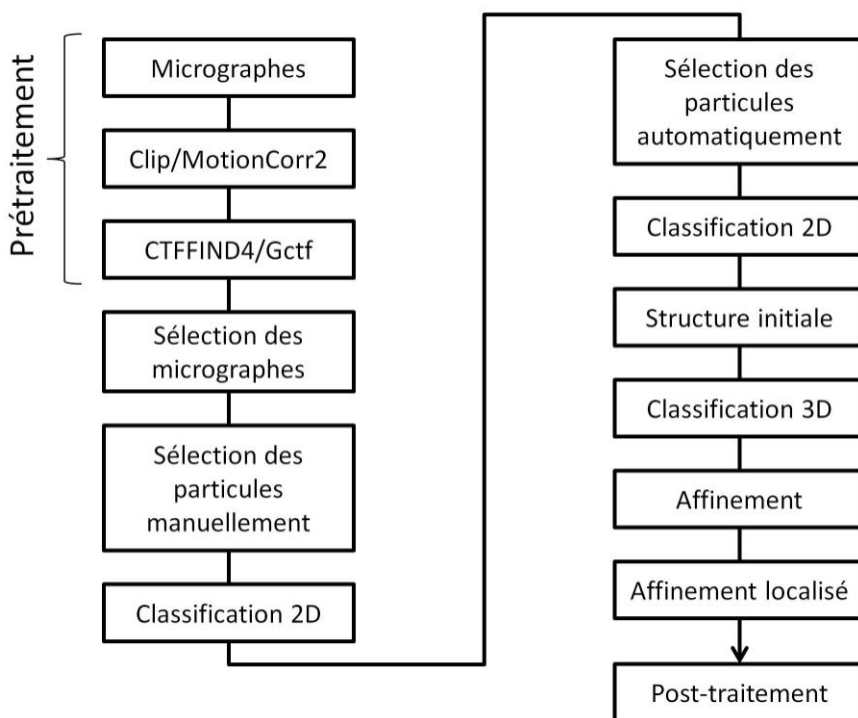
Figure 109 : Schéma des différentes étapes de traitement d'images.
