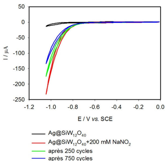
Figure IV. 13: Stability of 15 μL Ag@SiW 12 O 40 + 2 μL Nafion by sweep successively with 200 mmol·L -1 NaNO 2 in pH 5 1 mol·L -1 CH 3 COOLi + CH 3 COOH. \nu = 20 \text{ mV}\cdot\text{s}^{-1} .
