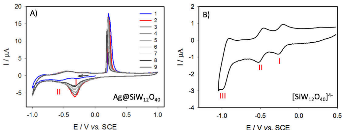
Figure IV.6: A) CV of 20 μL Ag@SiW 12 O 40 modified on GC electrode; B) CV of 0.1 mmol·L -1 [SiW 12 O 40 ] 4- in solution. Buffer solution: pH 5 1 mol·L -1 CH 3 COOLi + CH 3 COOH, \nu = 20 \text{ mV}\cdot\text{s}^{-1} .
