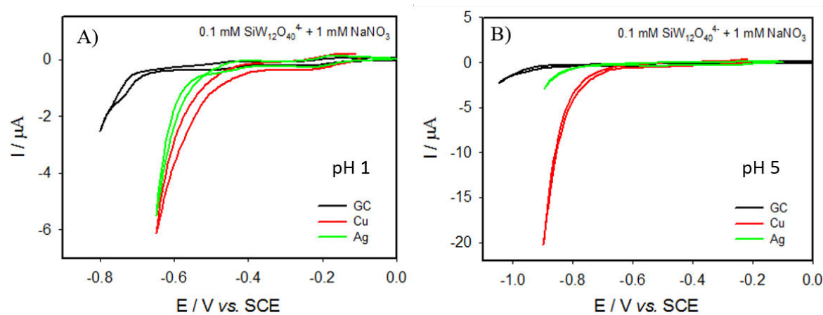
Figure II.21: Reduction of 1 mmol·L -1 NaNO 3 in the presence of 0.1 mmol·L -1 [SiW 12 O 40 ] 4- on GC, Cu and Ag electrodes, \nu = 2 \text{ mV}\cdot\text{s}^{-1} .
