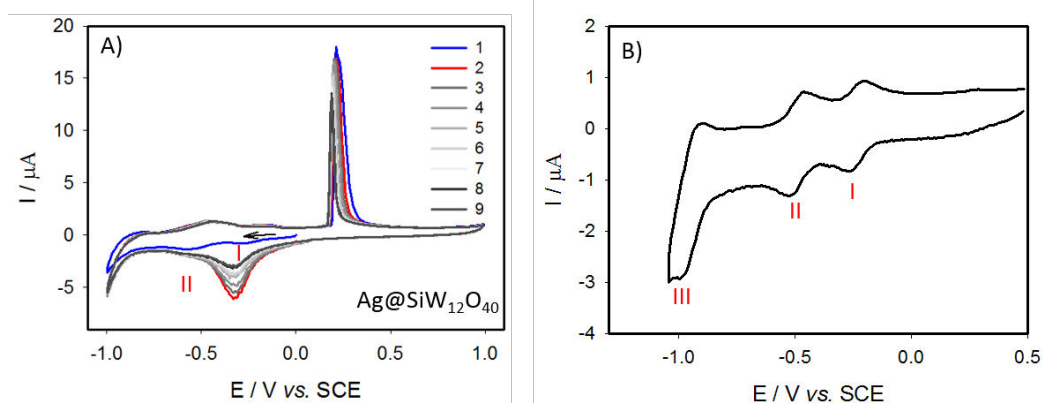
Figure 13 : A) CVs de la solution de nanoparticules Ag@SiW 12 O 40 . B) CV de [SiW 12 O 40 ] 4- en solution pH 5 (1 mol·L -1 CH 3 COOLi + CH 3 COOH), \nu = 20 \text{ mV}\cdot\text{s}^{-1} .
