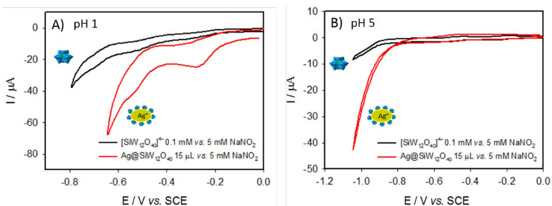
Figure 14 : Réduction de nitrite par Ag@SiW_{12}O_{40} déposé à la surface d'électrode ou par [SiW_{12}O_{40}]^{4-} dans la solution à pH 5 ( 1 \text{ mol}\cdot\text{L}^{-1} CH_3COOLi + CH_3COOH ) et à pH 1 ( 0,5 \text{ mol}\cdot\text{L}^{-1} Na_2SO_4 + H_2SO_4 ), v = 20 \text{ mV}\cdot\text{s}^{-1} .
