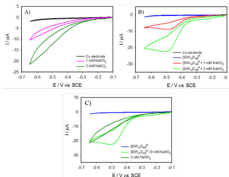
Figure 5 : Electroréduction de \text{HNO}_2 sur l'électrode de Cu en absence de \text{K}_4[\text{SiW}_{12}\text{O}_{40}]^{4-} (A) ou en présence de 0.1 \text{ mmol}\cdot\text{L}^{-1} \text{K}_4[\text{SiW}_{12}\text{O}_{40}]^{4-} (B). (C) comparaison de (A) et (B).
