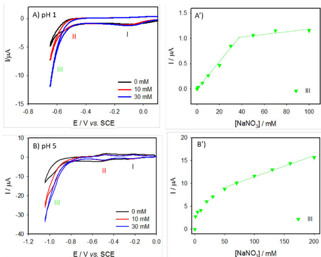
Figure 15 : Réduction de nitrate par Ag@SiW_{12}O_{40} déposé à la surface d'électrode à pH 5 ( 1 \text{ mol}\cdot\text{L}^{-1} CH_3COOLi + CH_3COOH ) et à pH 1 ( 0,5 \text{ mol}\cdot\text{L}^{-1} Na_2SO_4 + H_2SO_4 ), v = 20 \text{ mV}\cdot\text{s}^{-1} .
