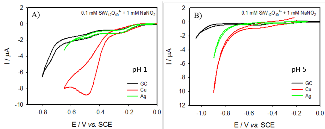
Figure II.13: Reduction of 1 mmol·L -1 NaNO 2 in the presence of 0.1 mmol·L -1 [SiW 12 O 40 ] 4- on GC, Cu and Ag electrodes, \nu = 2 \text{ mV} \cdot \text{s}^{-1} .
