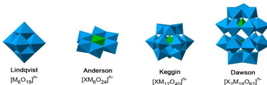
Figure 2 : Représentation de différentes structures de polyoxométallates (POMs).
