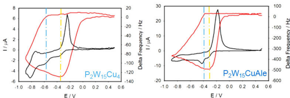
Figure 9 : Microbalance à Cristal de Quartz Electrochimique (EQCM) de \text{P}_2\text{W}_{15}\text{Cu}_4 et \text{P}_2\text{W}_{15}\text{CuAle} à \text{pH } 5 (1 \text{ mol} \cdot \text{L}^{-1} \text{ CH}_3\text{COOLi} + \text{CH}_3\text{COOH}) , v = 2 \text{ mV} \cdot \text{s}^{-1} .
