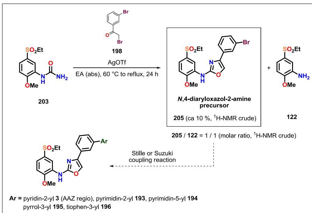
Schéme 28. Synthèse du précurseur de N ,4-diaryloxazol-2-amine 205 .
