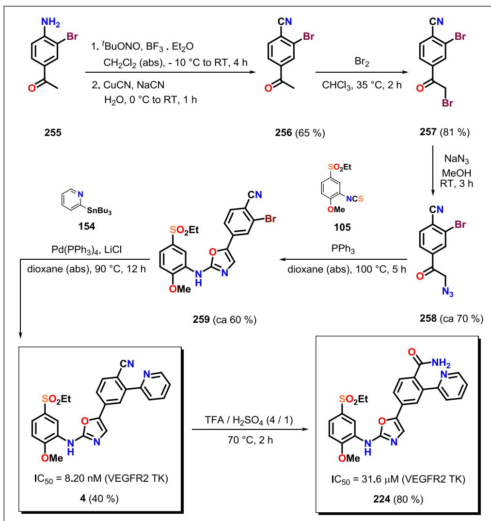
Schéme 37. Synthèse des N ,5-diaryloxazol-2-amines hétérocycliques p,m -disubstituées 4 et 224 .
