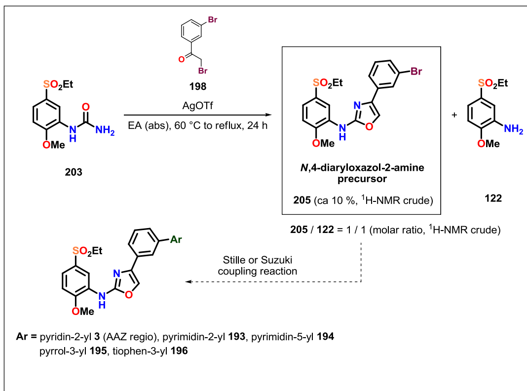
Scheme 28. Synthesis of N ,4-diaryloxazol-2-amine precursor 205.
