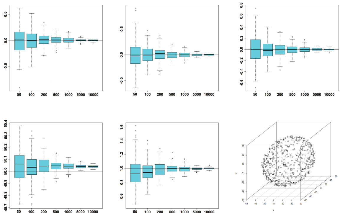
FIGURE 3.5.1 – Sur la première ligne, boîtes à moustaches des estimations (BF) de \mu_x , \mu_y et \mu_z respectivement. Sur la seconde ligne, boîtes à moustaches des estimations (BF) de r et \sigma^2 respectivement. En bas à droite, un échantillon de taille n = 1000 de la sphère considérée.
