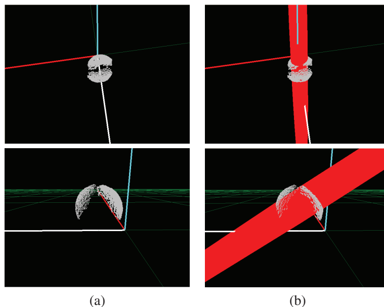
FIGURE 5.5.1 – En (a) le nuage de points 3D provenant des deux capteurs et en (b) l'ellipsoïde estimé.
